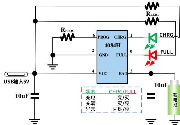
图 5.b 4084HB6 典型应用拓扑
