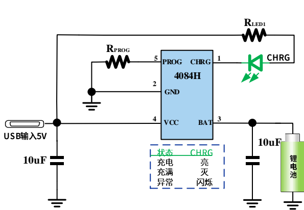
图 5.a 4084HB5 典型应用拓扑
