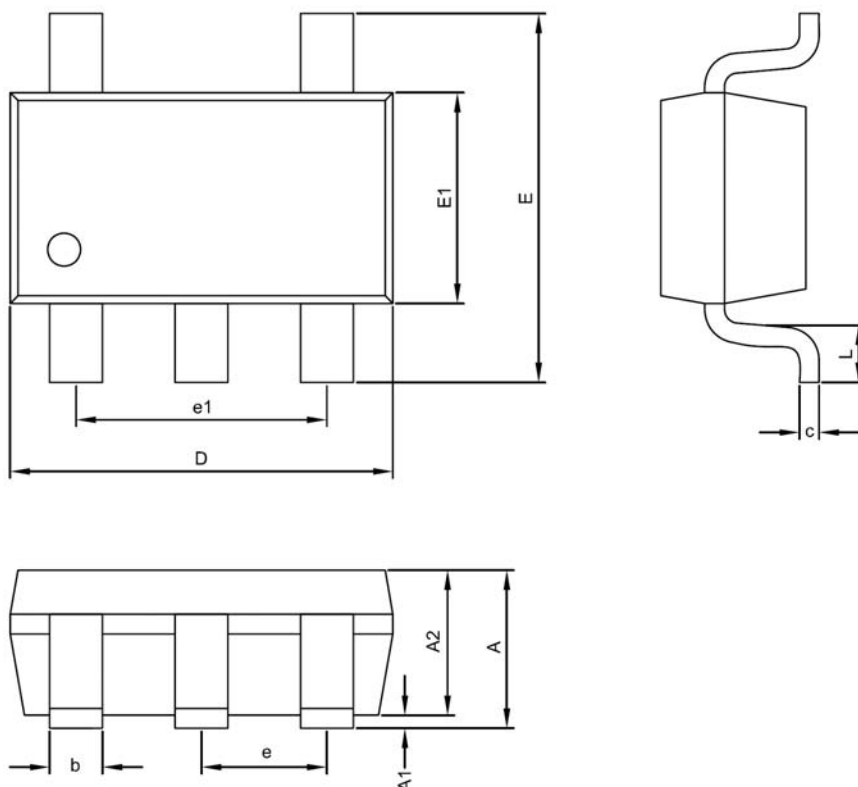
SOT-23-5 Package
