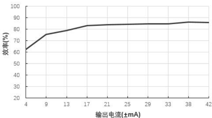
效率 VS 输出电流 E1212S-1W@ (Vin=12V)
