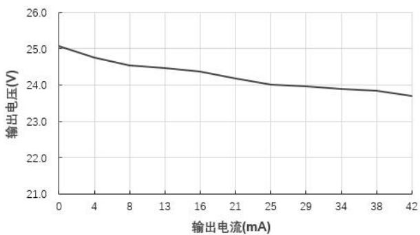
输出电压Vs输出电流(Vin=5V)@B0524LS-1WR2
