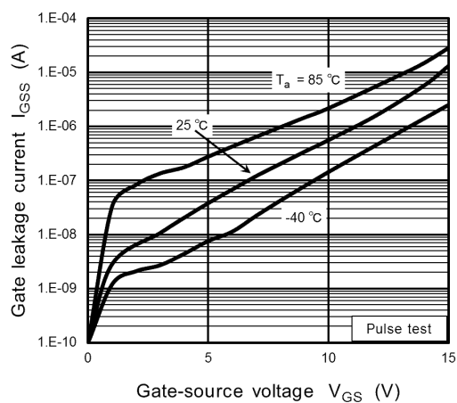
Fig. 9.6 I_{GSS} - V_{GS}
