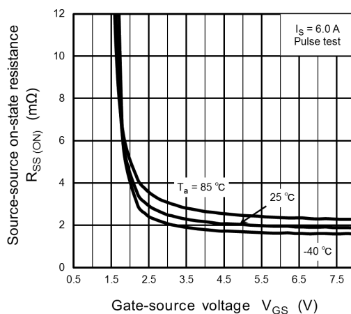
Fig. 9.4 R_{SS(ON)} - V_{GS}
