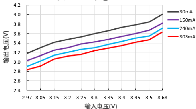
输出电压Vs输入电压@B0303LS-1WR2
