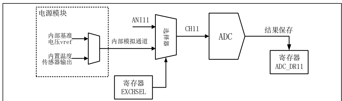
图 14-2 内部模拟通道选择
