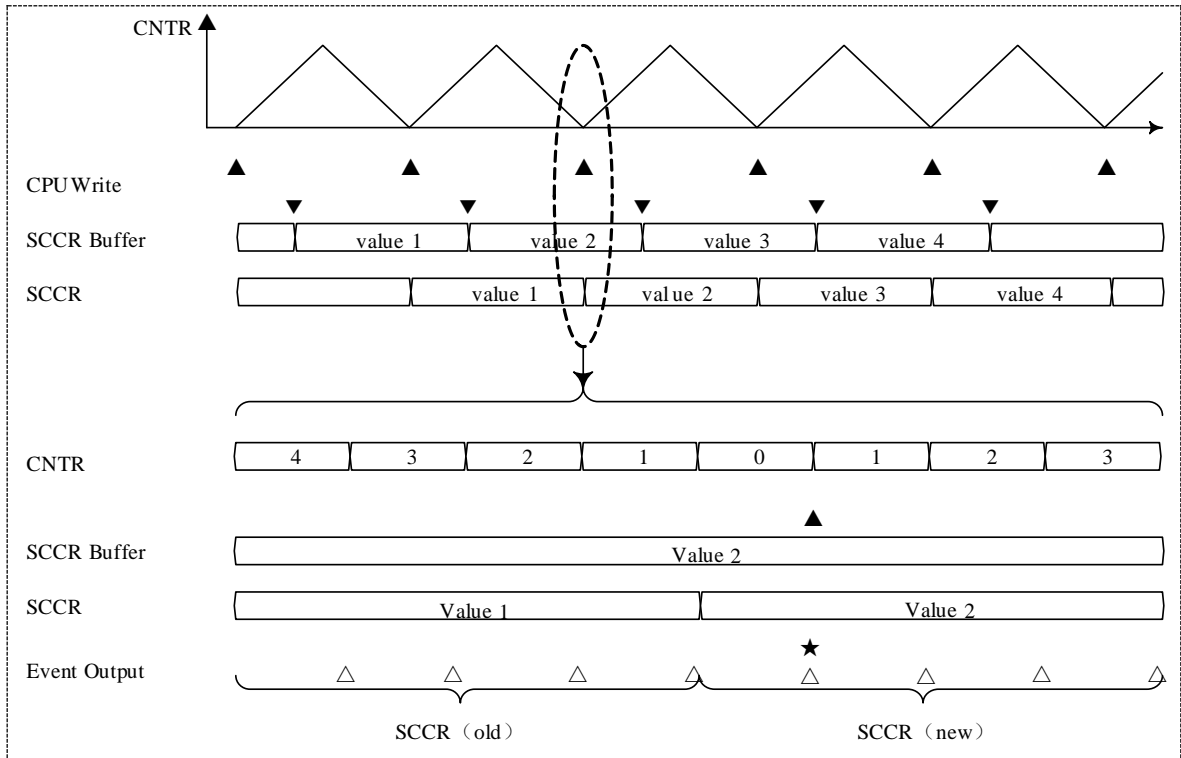
图 15-14 SCCR 缓冲传输操作（周期间隔响应链接传输禁止时）
