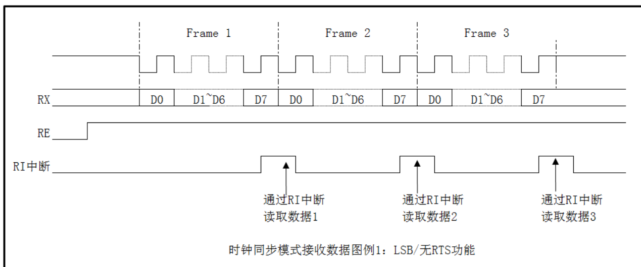
图 22-17 时钟同步模式接收数据图例 1
