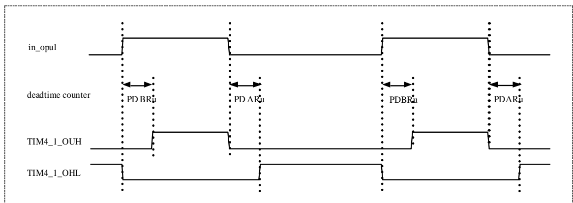
图 15-20 死区定时器模式下的互补 PWM 输出
