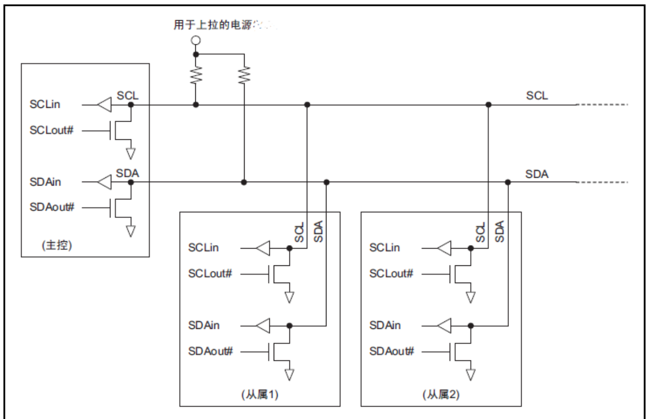
图 23-2 I2C 总线的结构例
