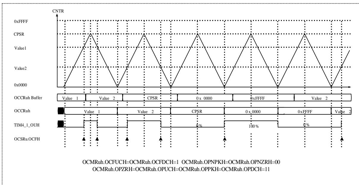
图 15-17 三角波独立 PWM 输出例
