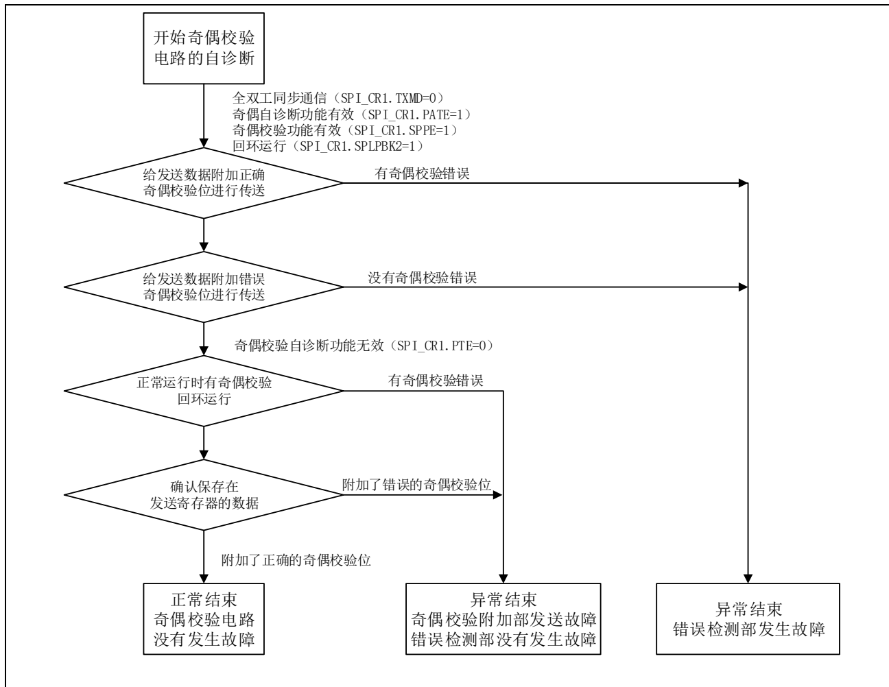
图 24-9 奇偶校验流程
