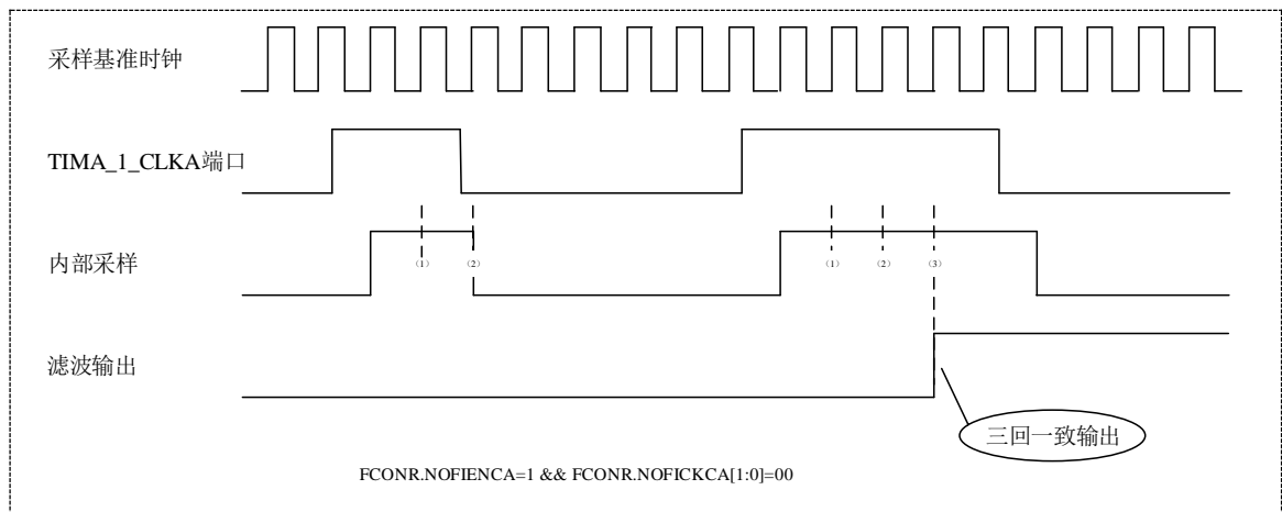
图 18-6 时钟输入端口的滤波功能
