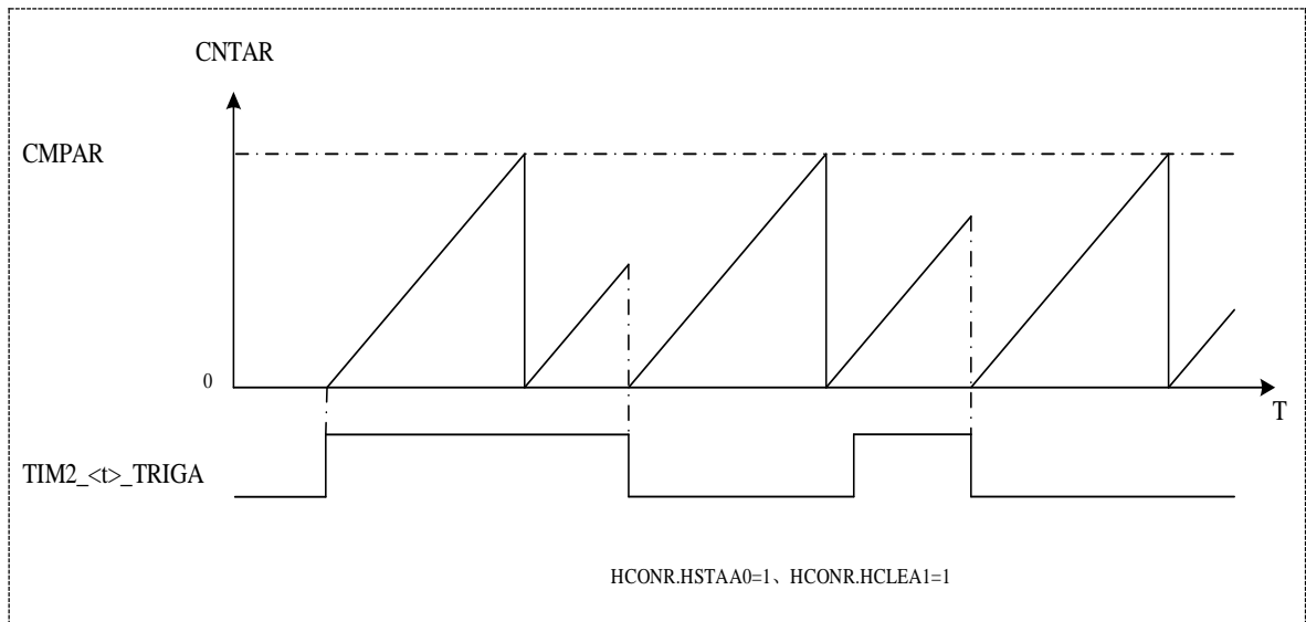
图 19-3 硬件启动、清零动作
