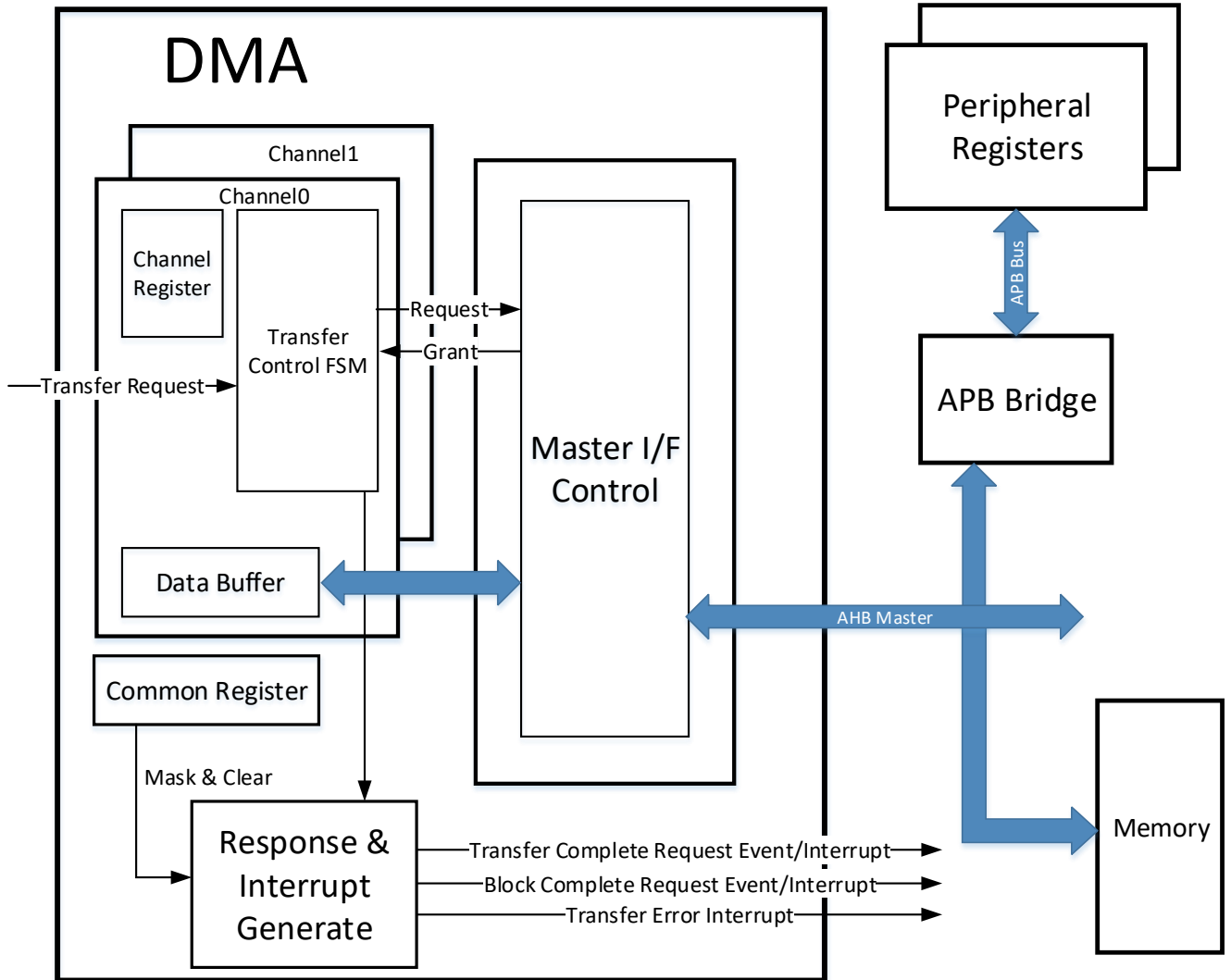
图 11-1 DMA 结构图
