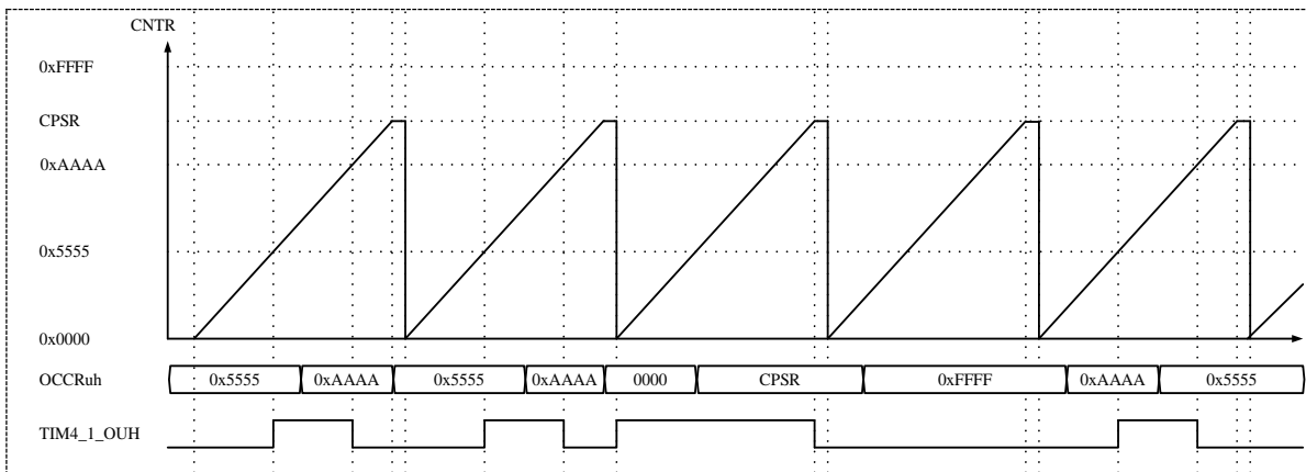
图 15-6 锯齿波模式波形输出例
