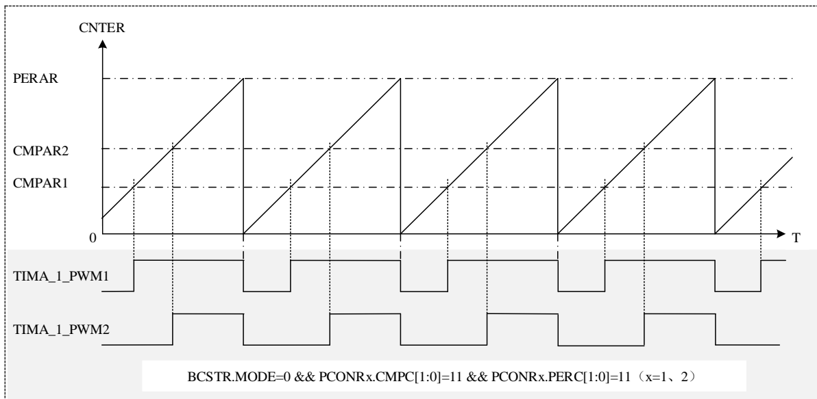
图 18-8 单边对齐 PWM 输出例
