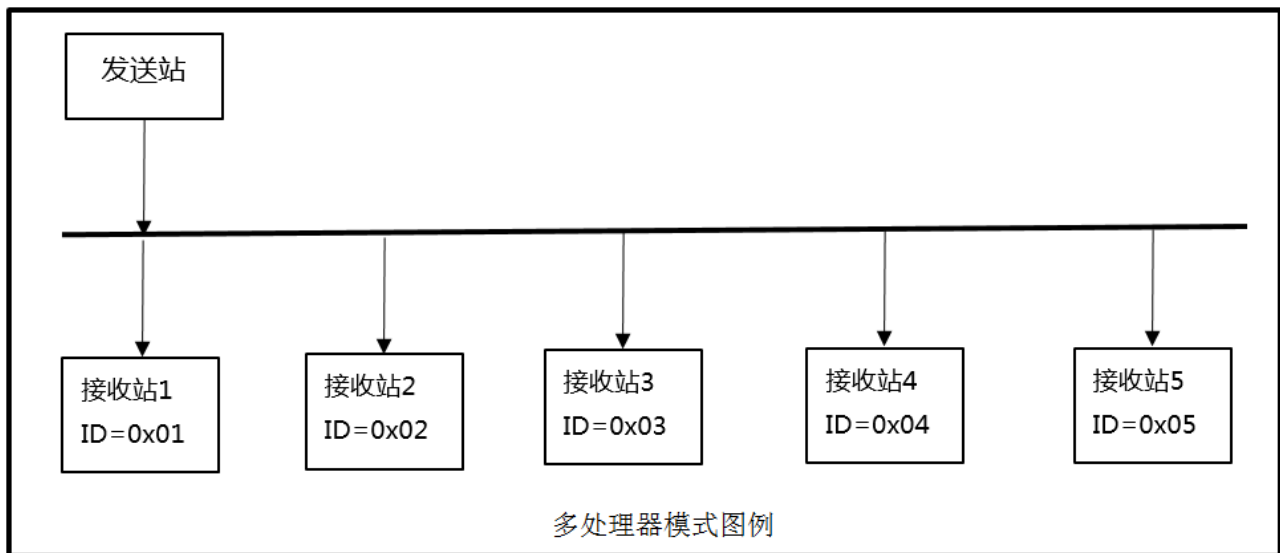
图 22-8 多处理器通信图例
