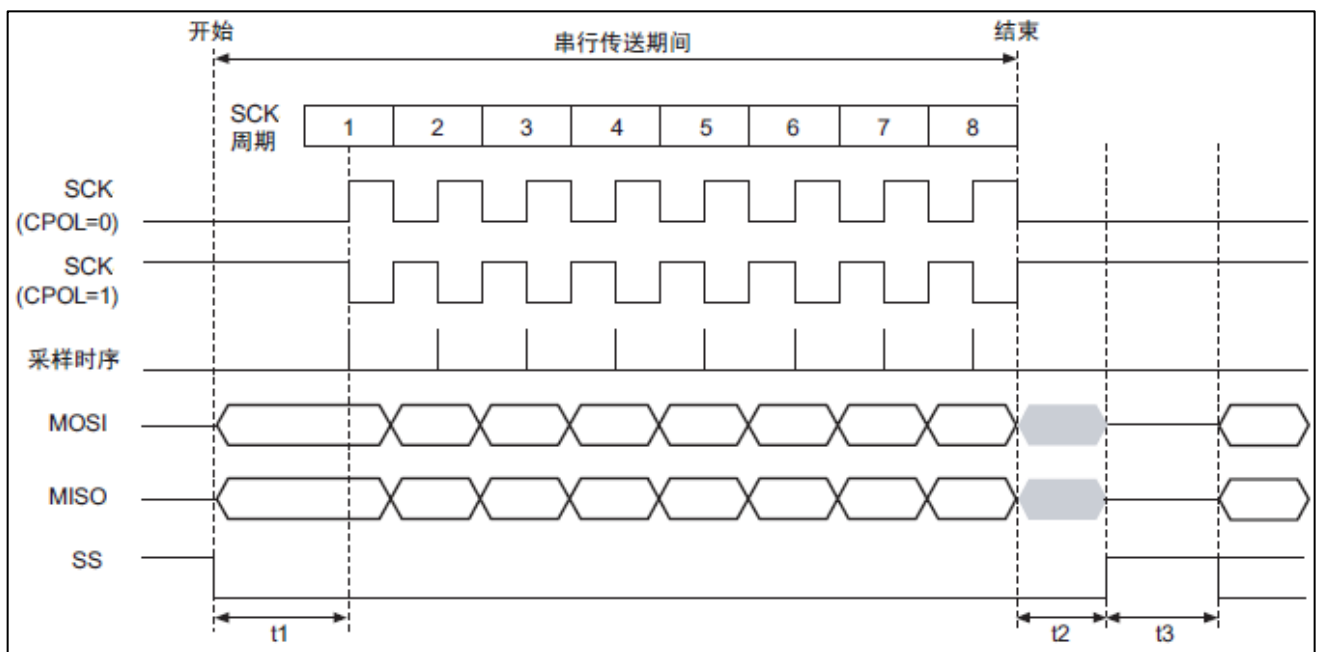
图 24-5 数据传送格式图 (CPHA=0)
