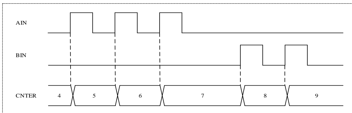
图 18-10 位置模式-基本计数
