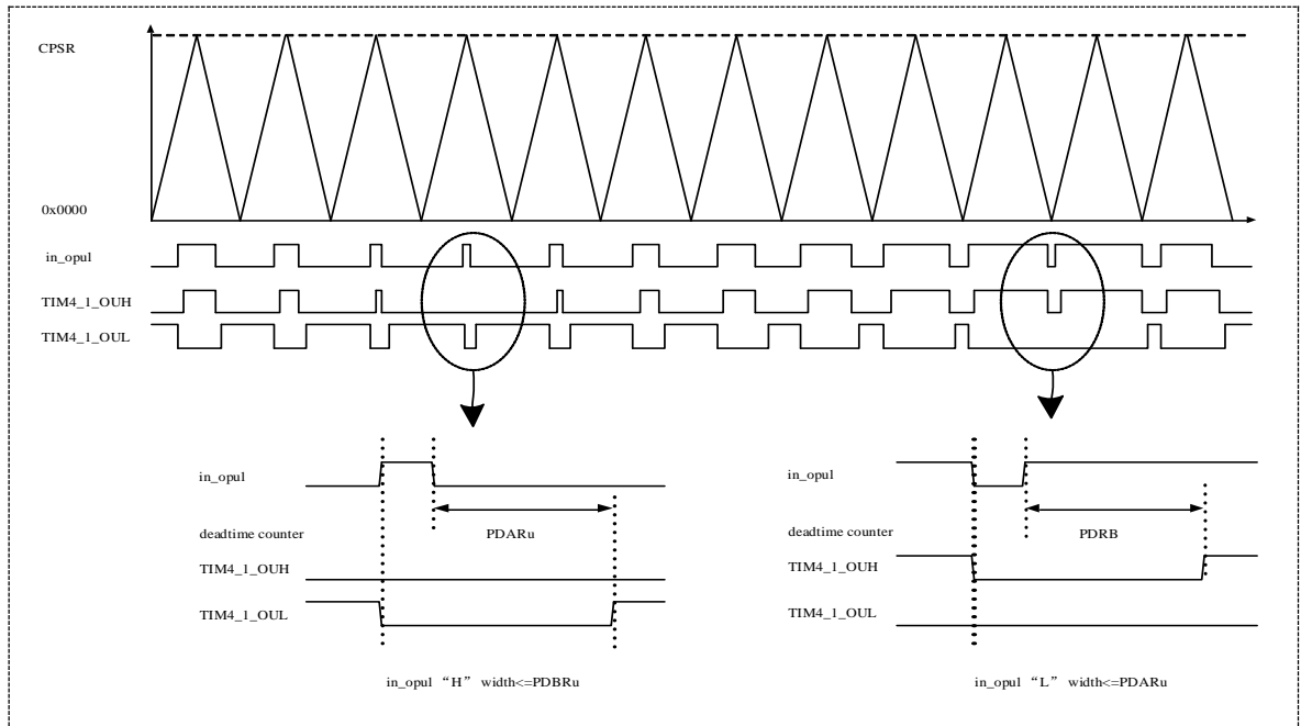
图 15-21 脉宽异常时的死区定时器模式下的波形输出
