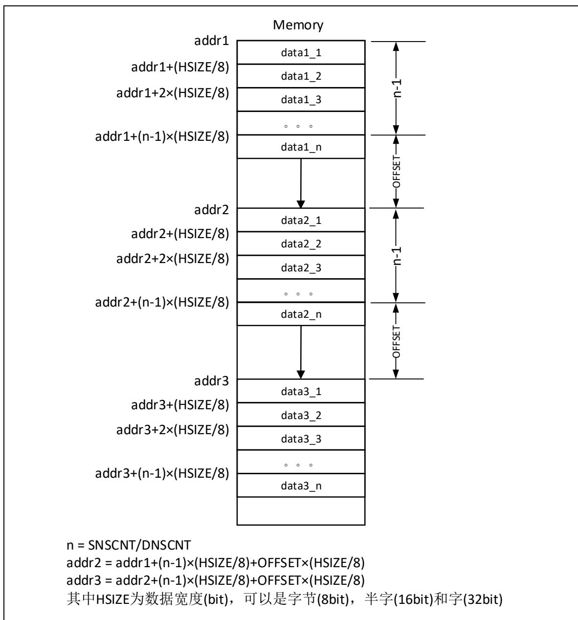
图 11-3 不连续地址传输示意图
