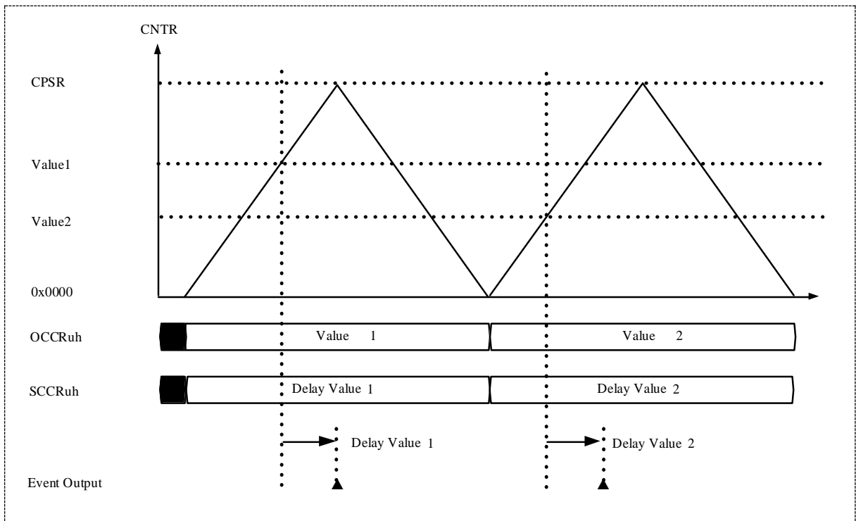
图 15-25 延时启动模式下专用事件输出信号的输出时序
