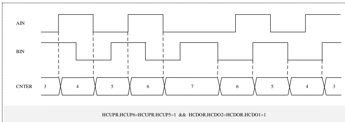
图 18-12 位置计数模式-相位差计数（2 倍计数）
