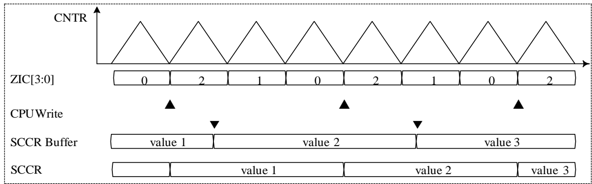
图 15-15 SCCR 缓冲传输操作（周期间隔响应链接传输使能时）
