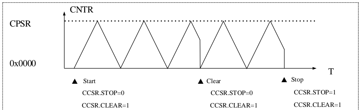
图 15-5 Timer4 三角波模式计数动作
