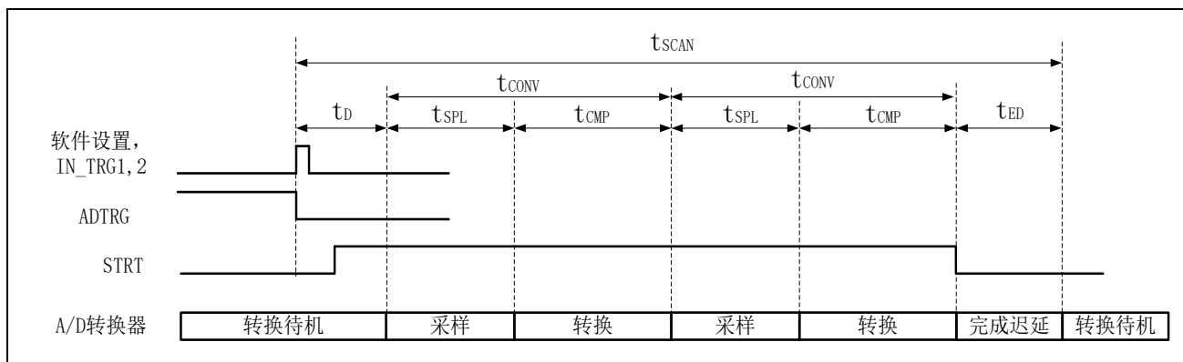
图 14-8 A/D 转换时间
