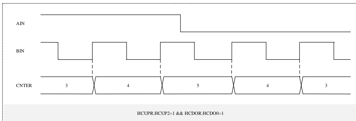
图 18-14 位置计数模式-方向计数
