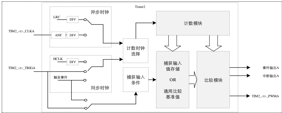
图 19-1 Timer2 基本框图
