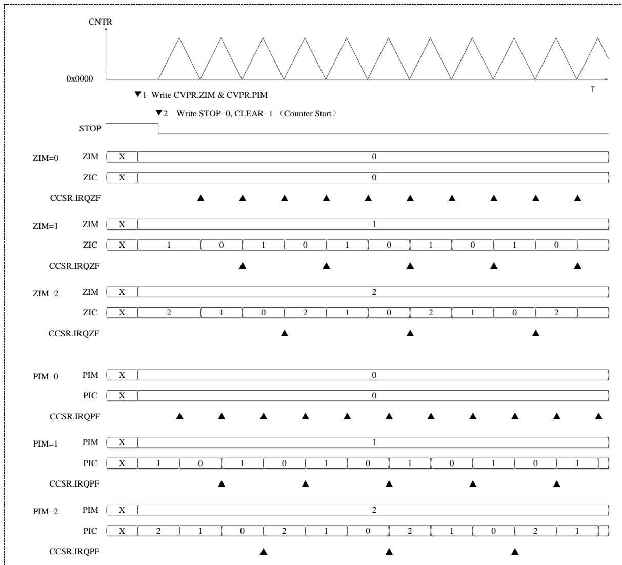
图 15-23 周期间隔响应时序图
