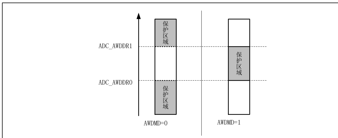
图 14-7 模拟看门狗保护区域（比较条件）
