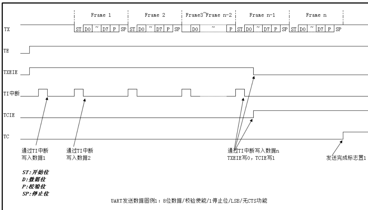
图 22-3 UART 发送数据图例 1
