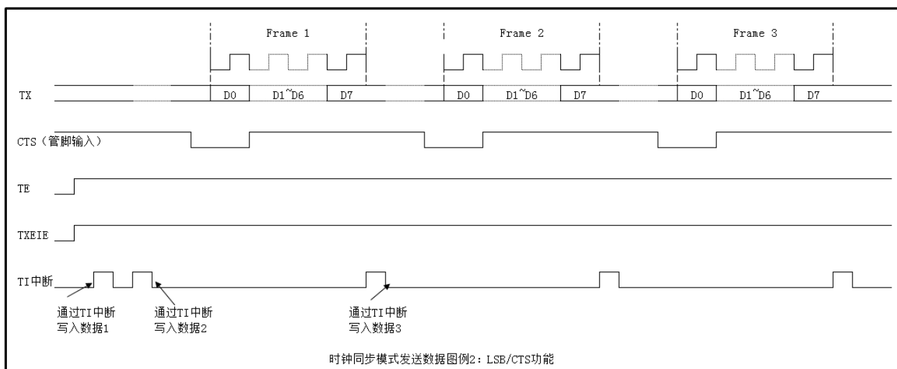
图 22-16 时钟同步模式发送数据图例 2
