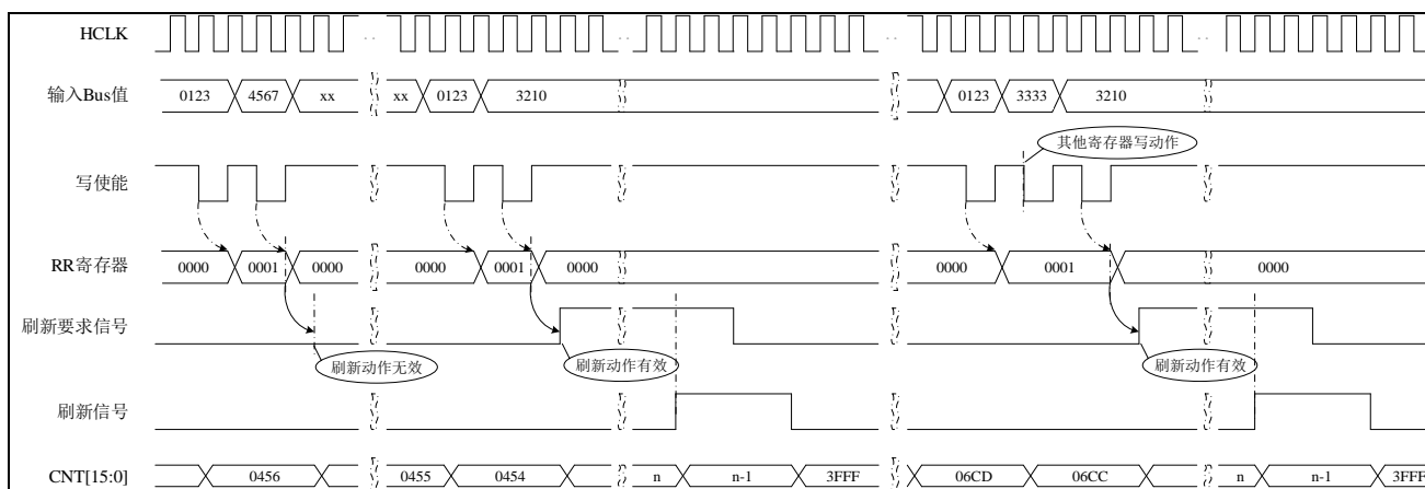
图 21-3 各种刷新动作时序示例（动作确认，刷新要求信号的下降沿等）
