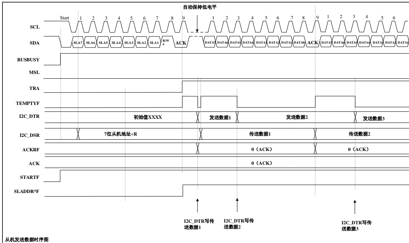
图 23-7 7 位地址格式的从机发送模式时序图（例）
