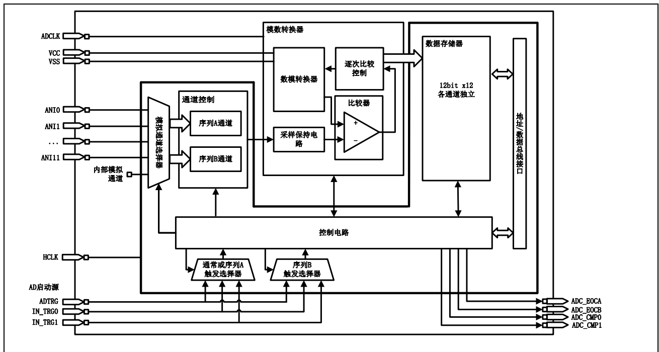
图 14-1 ADC 框图
