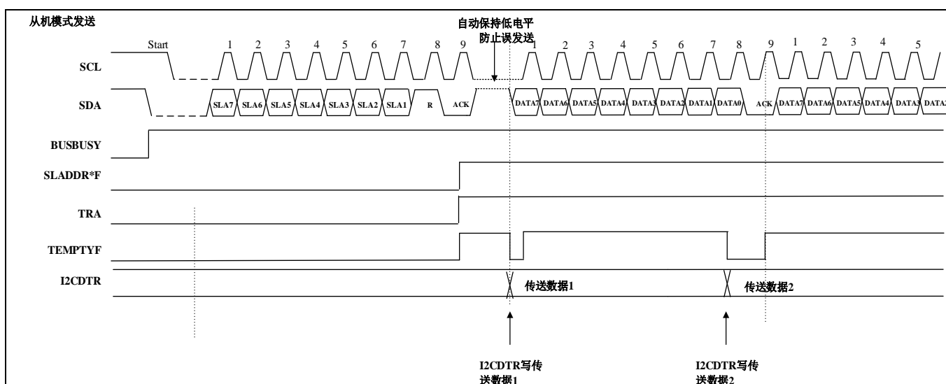
图 23-10 从机发送时序图（1）
