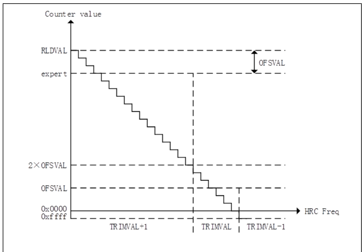
图 12-2 CTC 校准示意图
