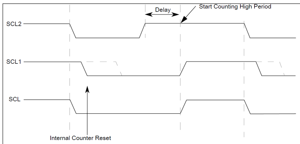
图 23-9 SCL 同步时序
