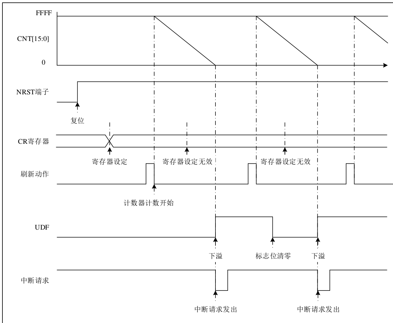
图 21-2 软件启动例
