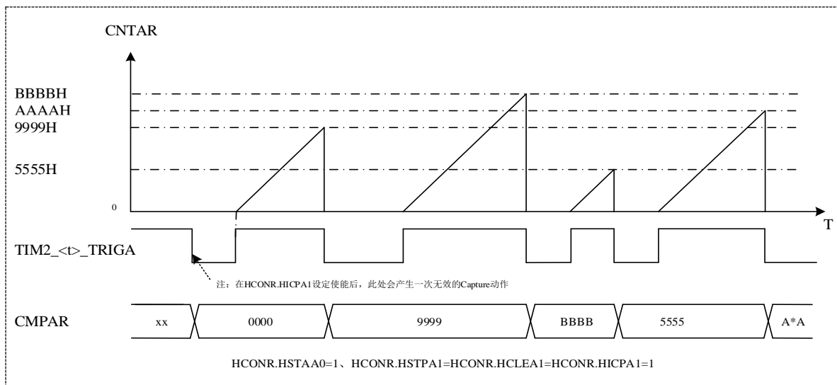
图 19-5 脉宽测量
