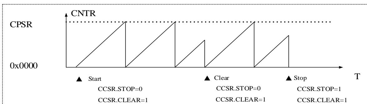
图 15-4 Timer4 锯齿波模式计数动作
