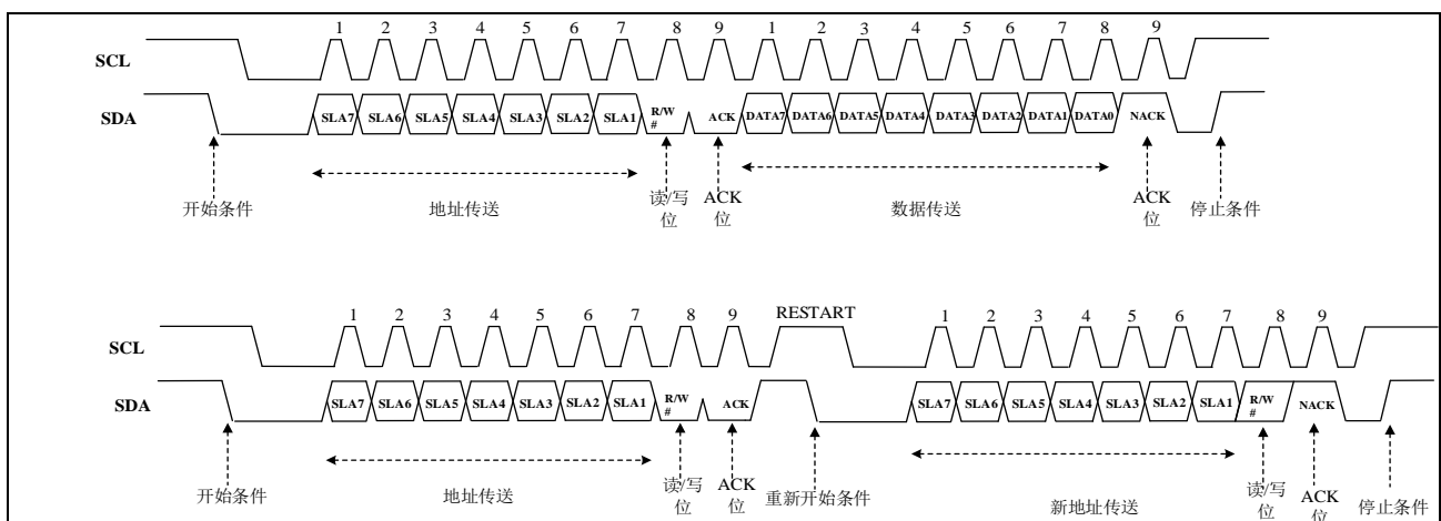
图 23-3 I 2 C 总线的时序图
