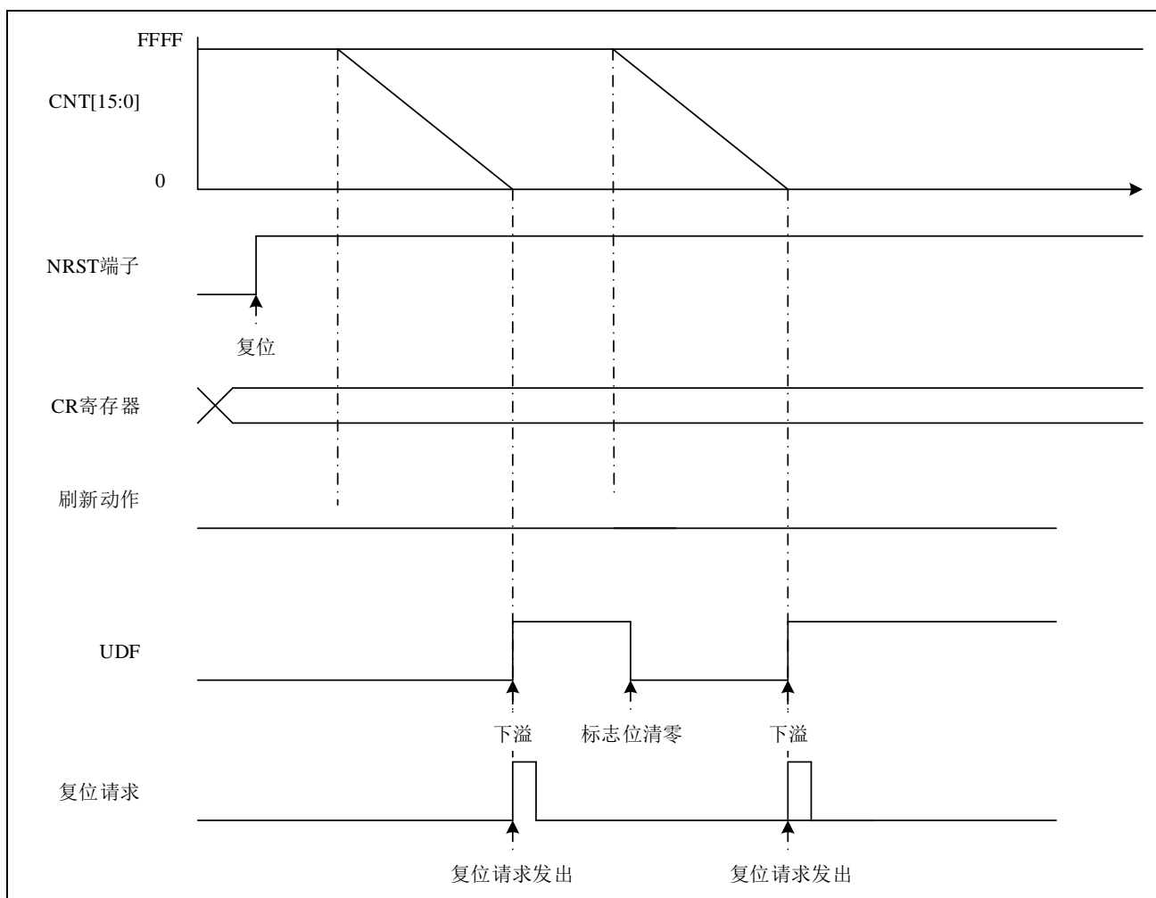
图 21-1 硬件启动例
