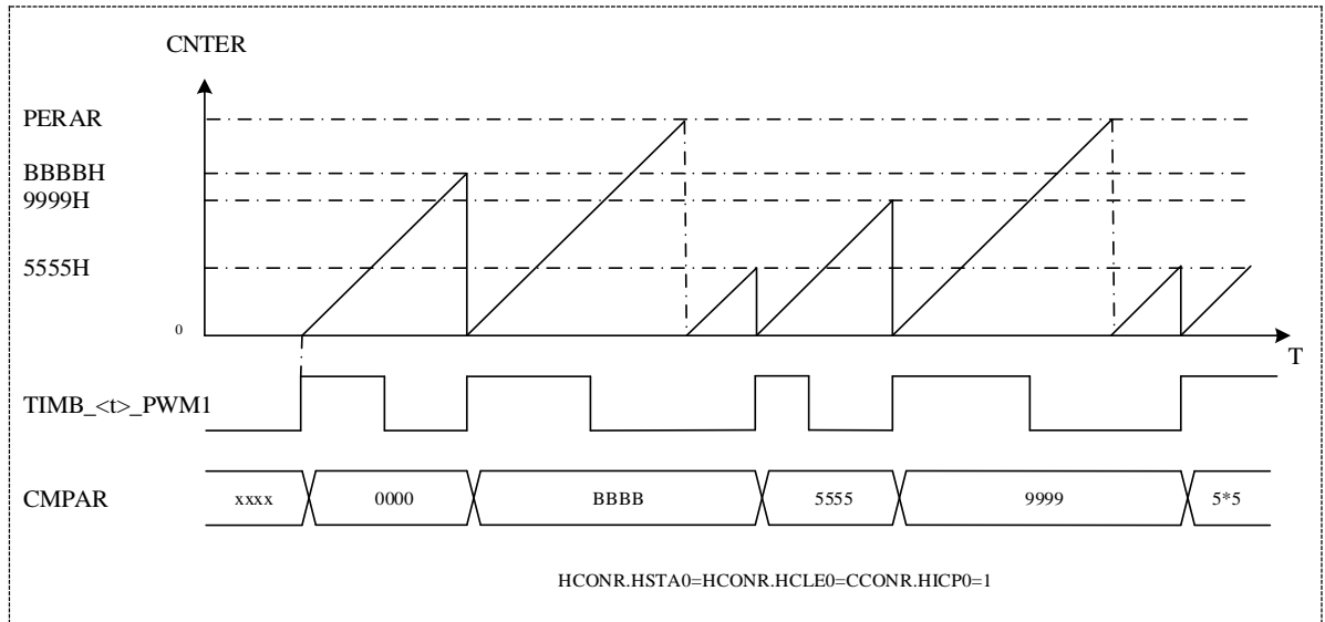
图 17-10 周期测量
