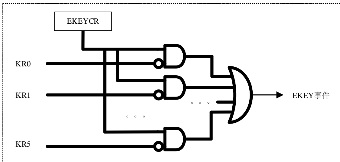
图 10-2 EKEY 事件产生
