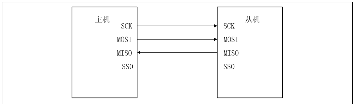
图 24-3 三线式时钟同步运行
