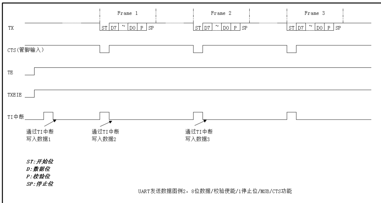
图 22-4 UART 发送数据图例 2
