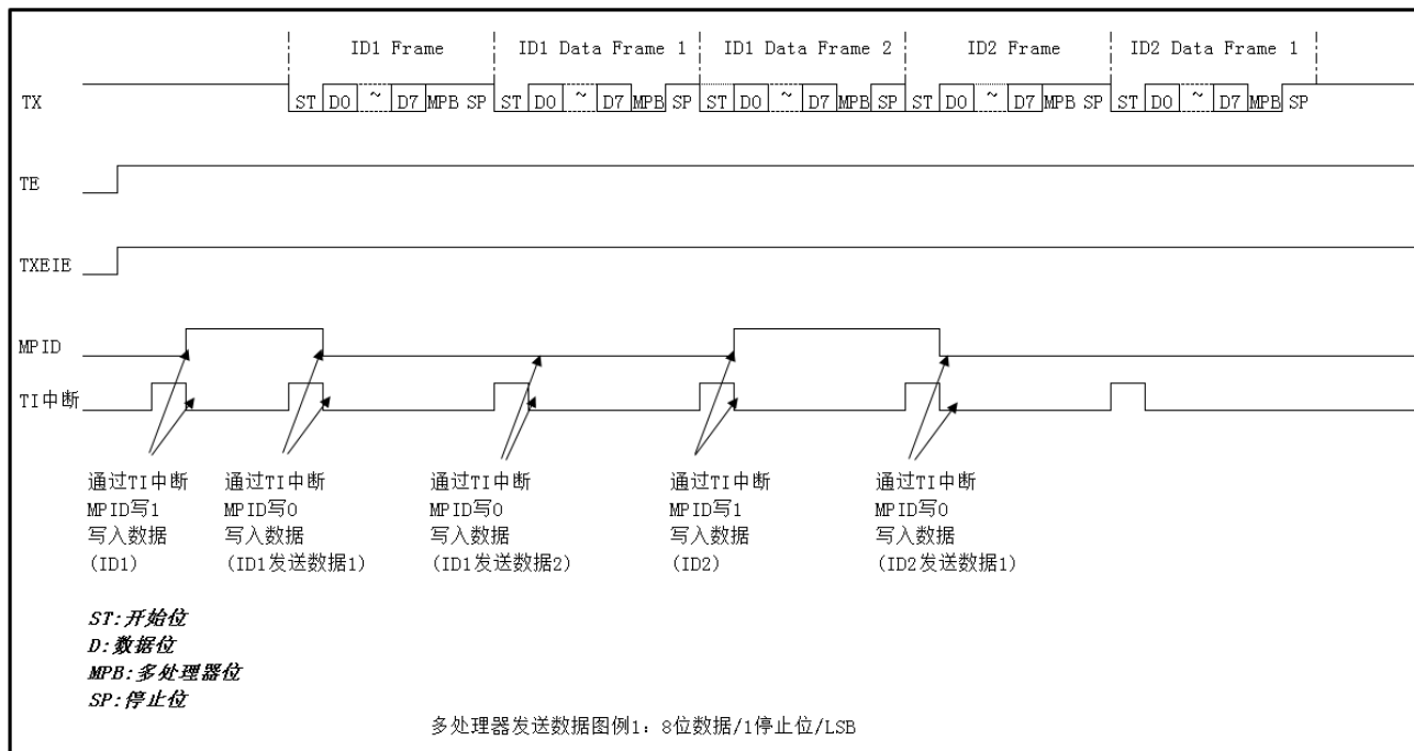
图 22-10 多处理器模式发送数据图例
