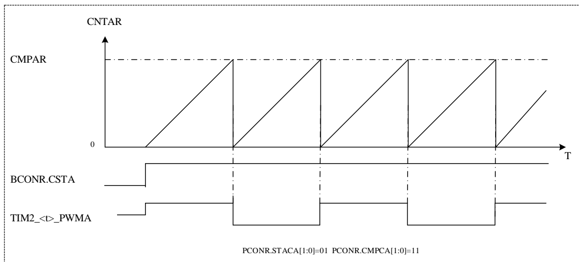
图 19-2 比较输出动作
