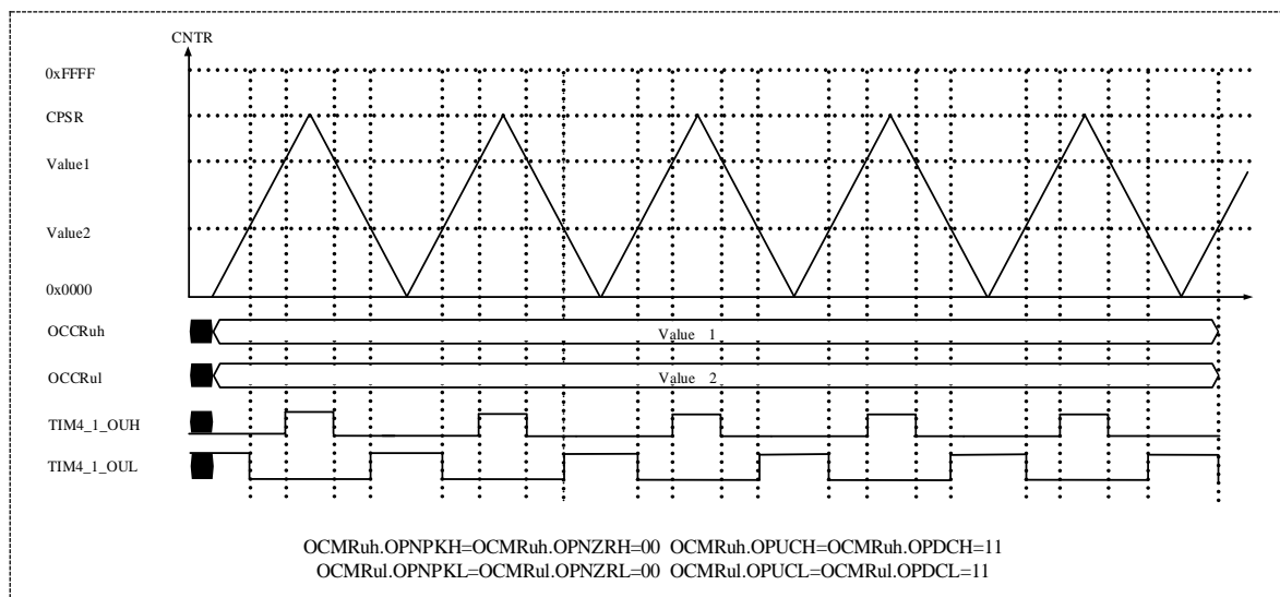
图 15-19 软件实现互补 PWM 输出
