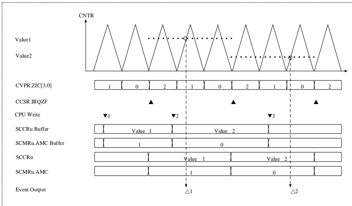
图 15-24 专用事件输出信号周期间隔响应输出
