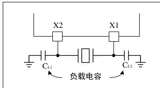
图 4-2 外部高速振荡器连接事例
