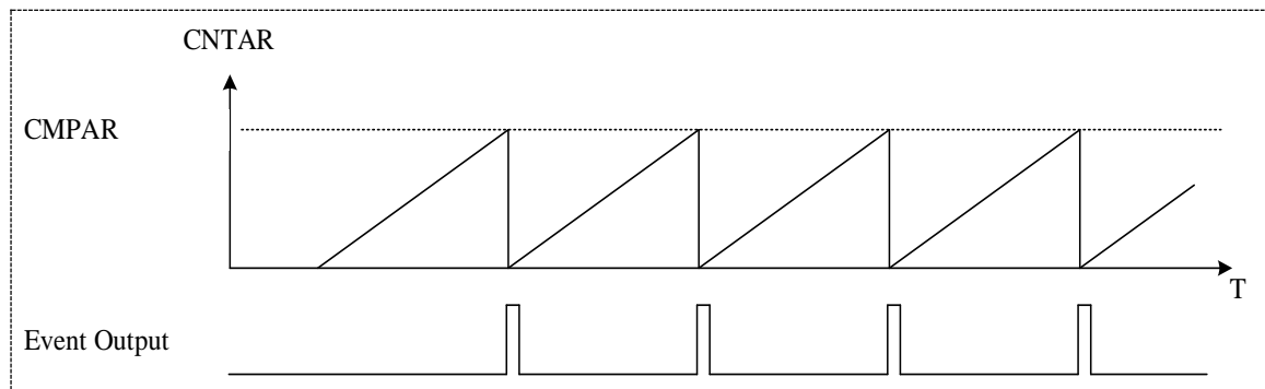
图 20-2 Timer0 计数时序图
