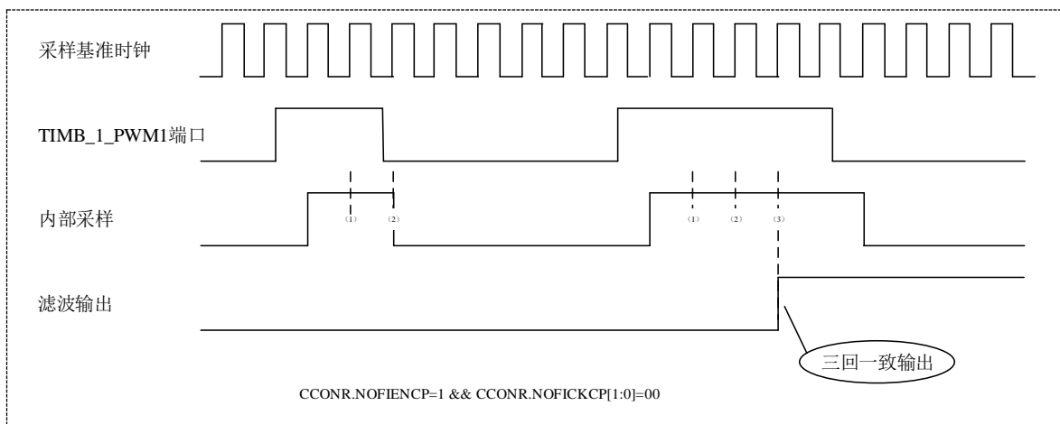
图 17-7 PWM 输入端口的滤波功能
