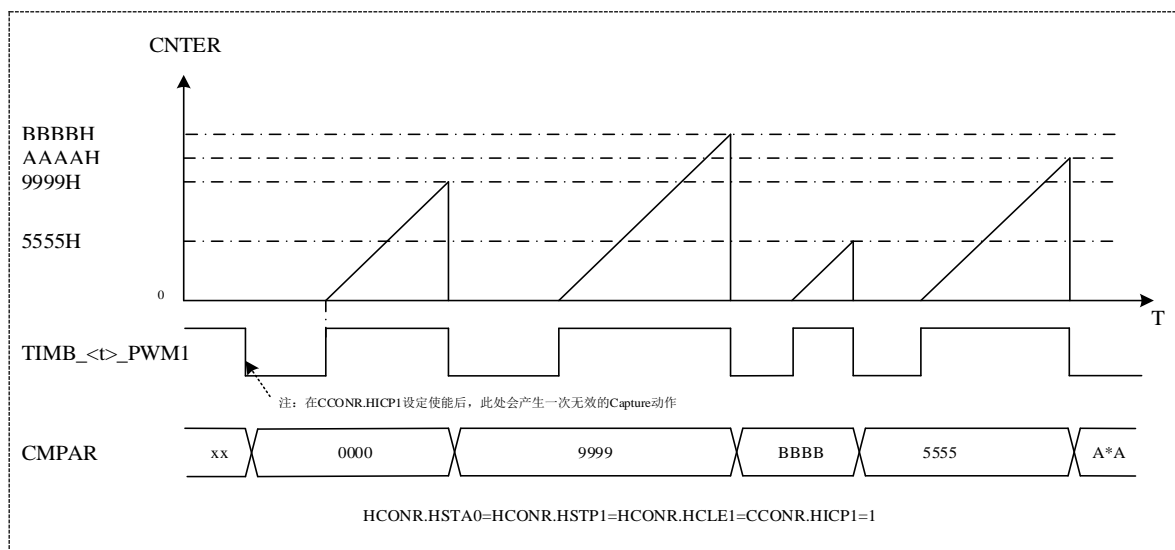
图 17-9 脉宽测量
