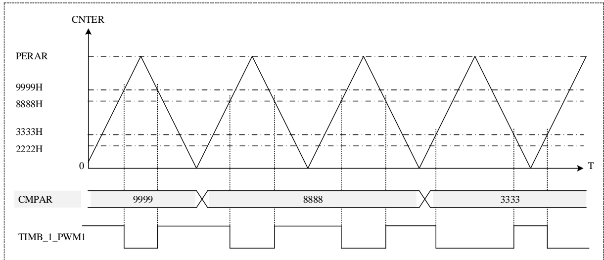
图 17-12 双边对称 PWM 输出例
