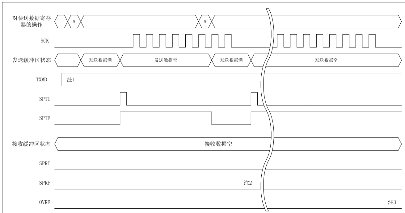
图 24-8 只进行发送通信
