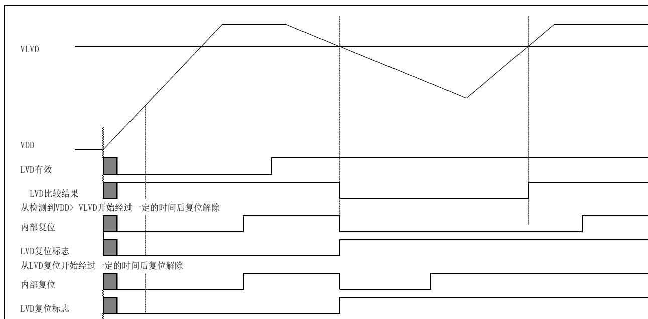
图 5-5 LVD 复位时序图
