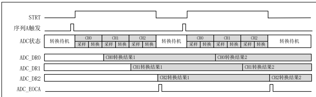
图 14-3 序列 A 单次扫描模式
