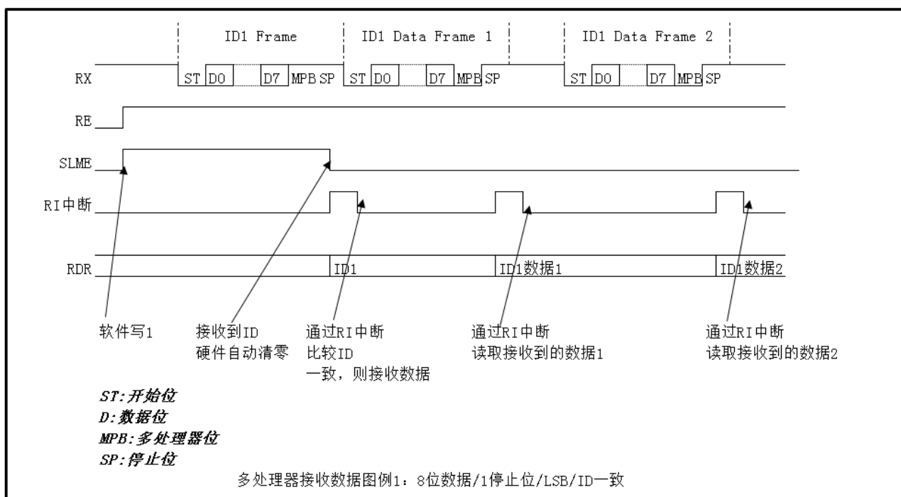
图 22-11 多处理器模式接收数据图例 1
