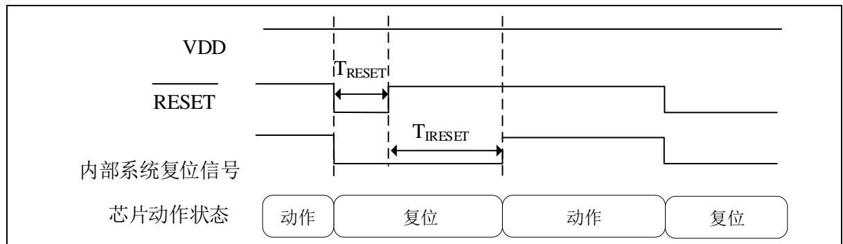
图 3-2 RESET 复位时序
