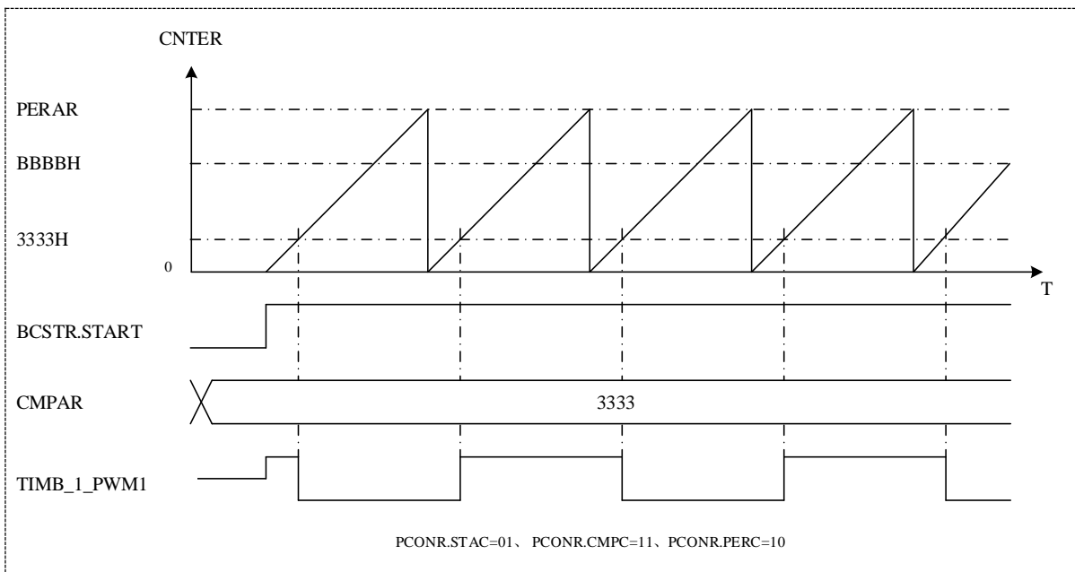
图 17-4 比较输出动作
