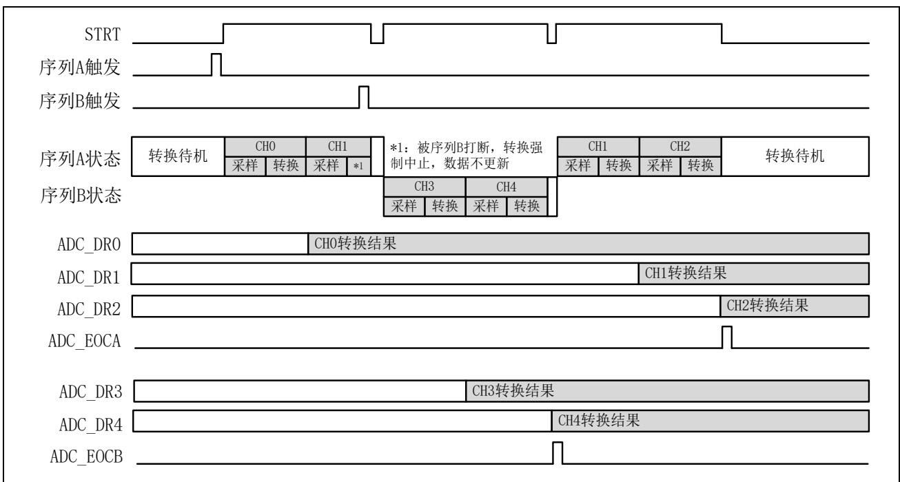
图 14-5 双序列扫描模式 (RSCHSEL=0 序列 A 从被中断通道重新启动)
