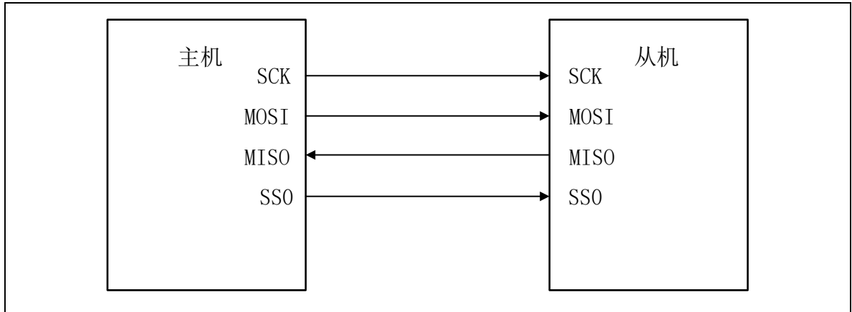
图 24-2 主机模式结构
