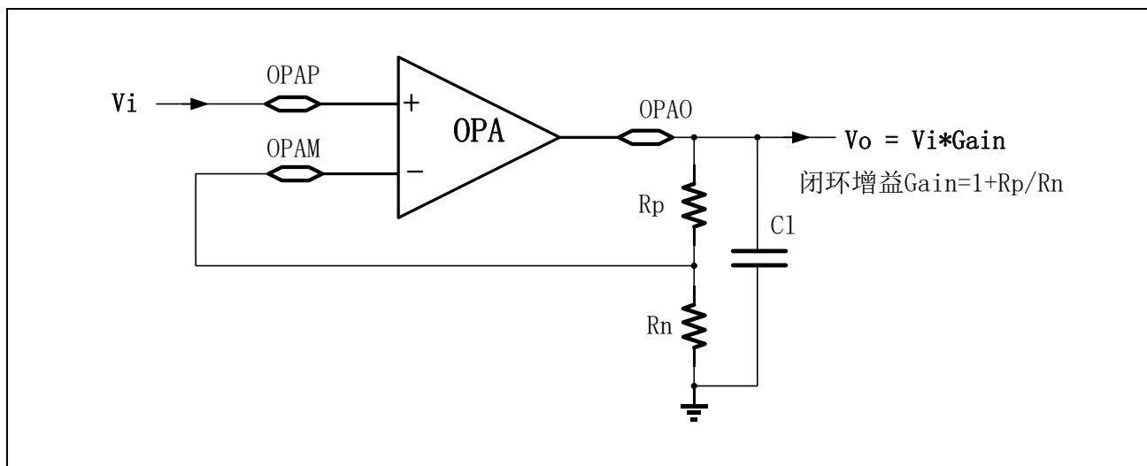
图 14-9 OPA 工作示意图
