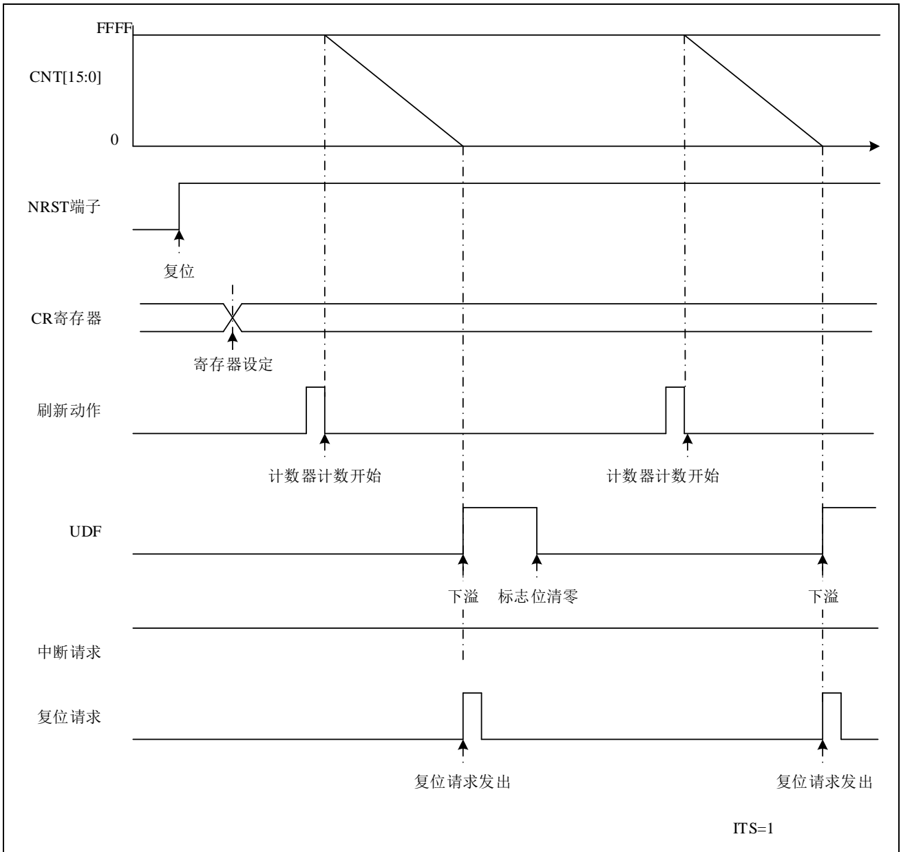
图 21-4 计数器下溢动作例
