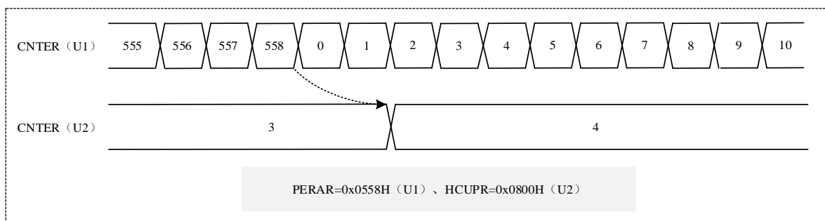
图 17-8 32 位级联计数动作
