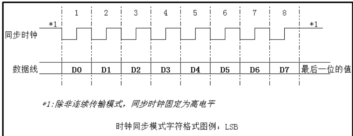
图 22-14 时钟同步模式数据格式
