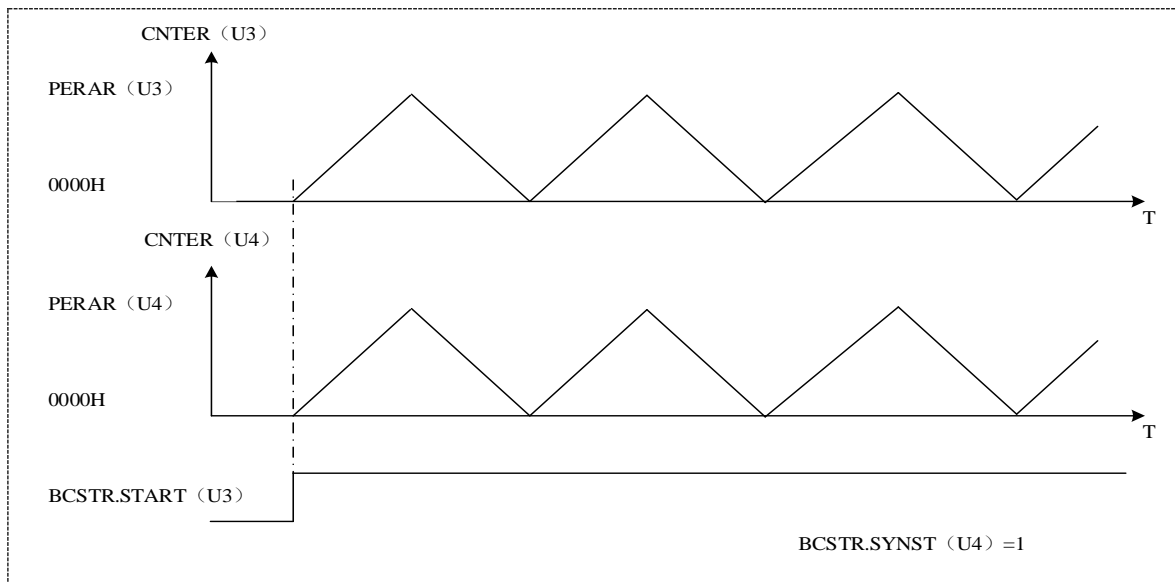
图 17-6 软件同步动作
