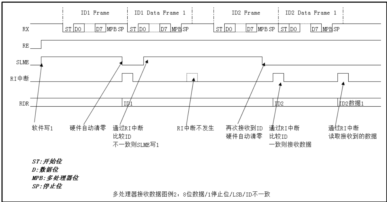
图 22-12 多处理器模式接收数据图例 2
