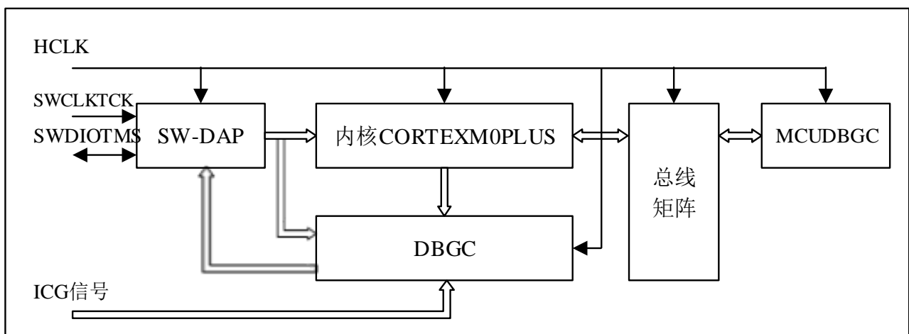
图 26-1 调试控制系统
