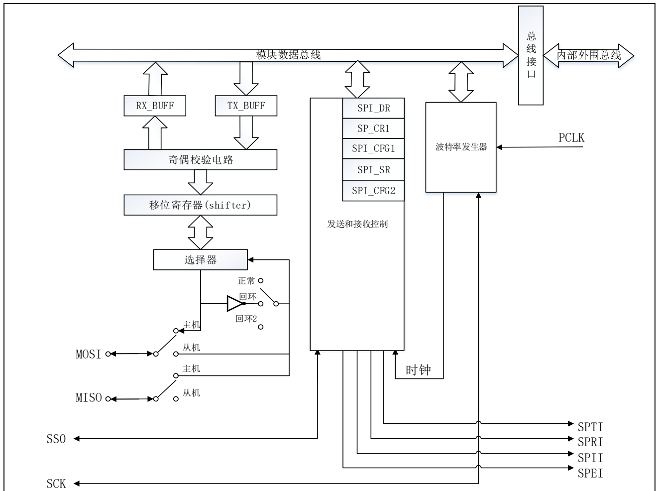
图 24-1 系统框图
