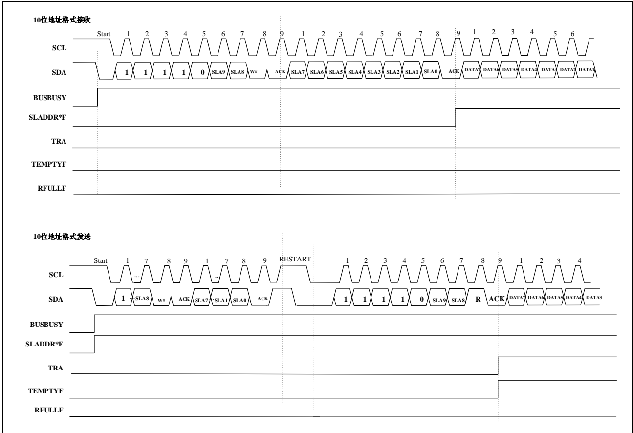
图 23-13 选择 10 位地址格式时的时序
