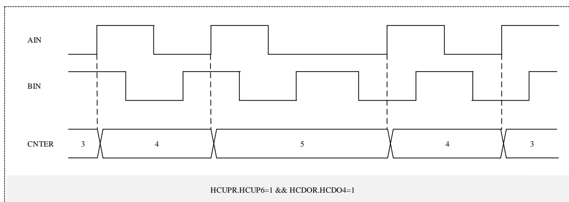
图 18-11 位置计数模式-相位差计数（1 倍计数）
