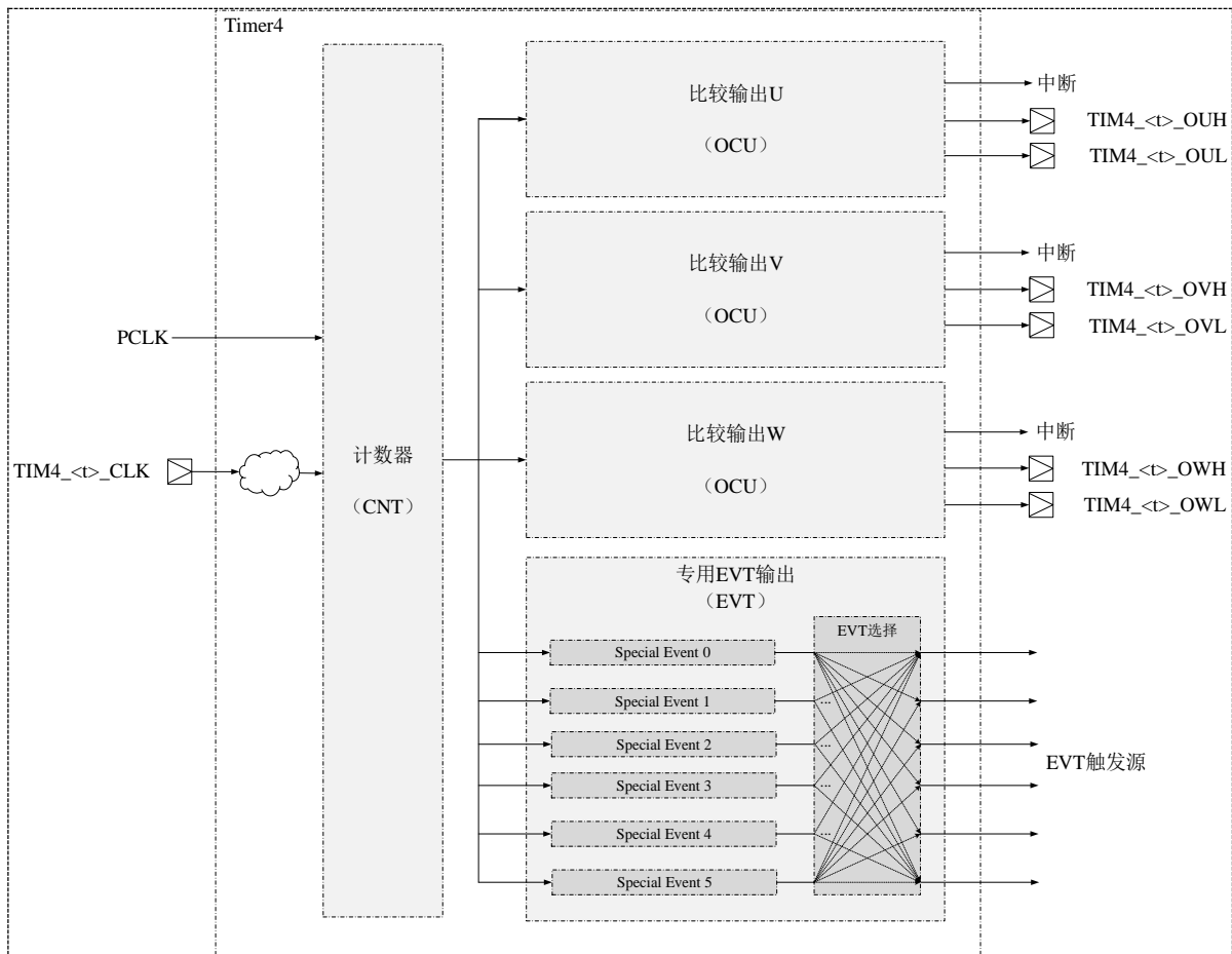
图 15-1 Timer4 基本框图
