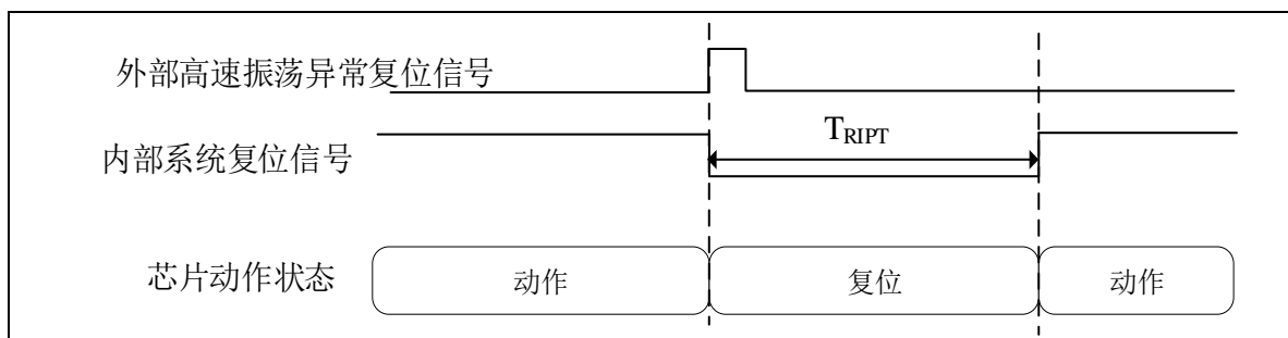
图 3-8 外部高速振荡异常复位
