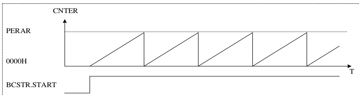
图 17-2 锯齿波波形（递加计数）
