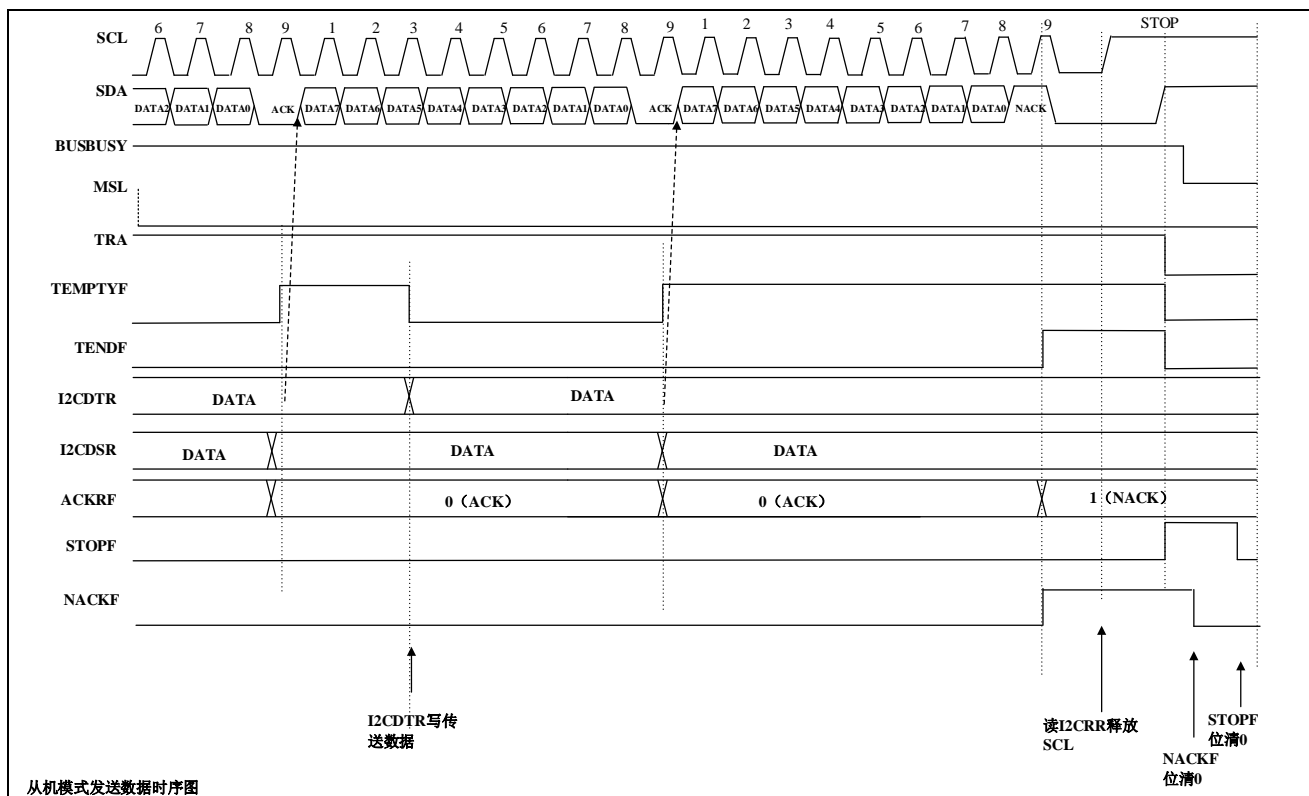
图 23-11 从机发送时序图 (2)
