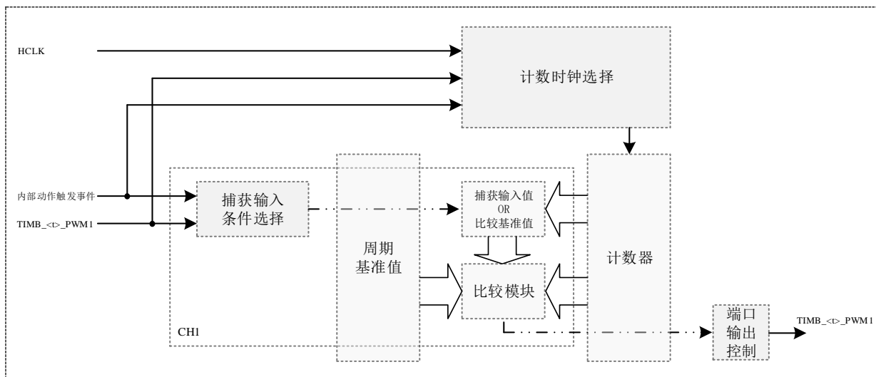
图 17-1 TimerB 基本框图
