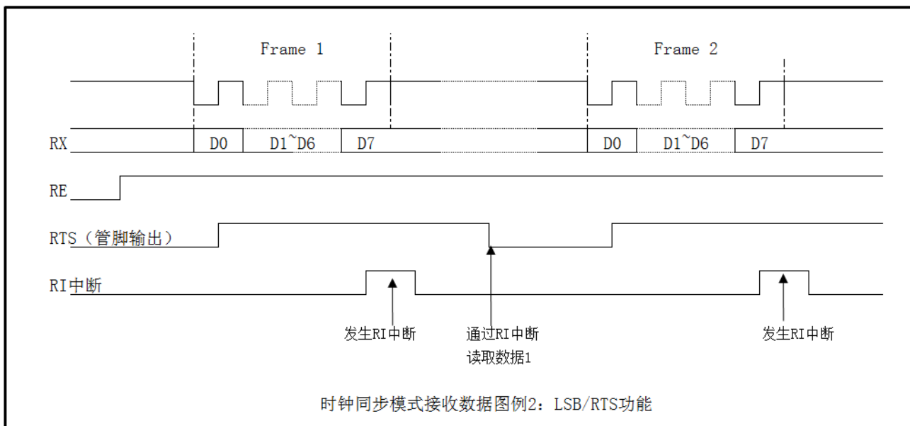
图 22-18 时钟同步模式接收数据图例 2
