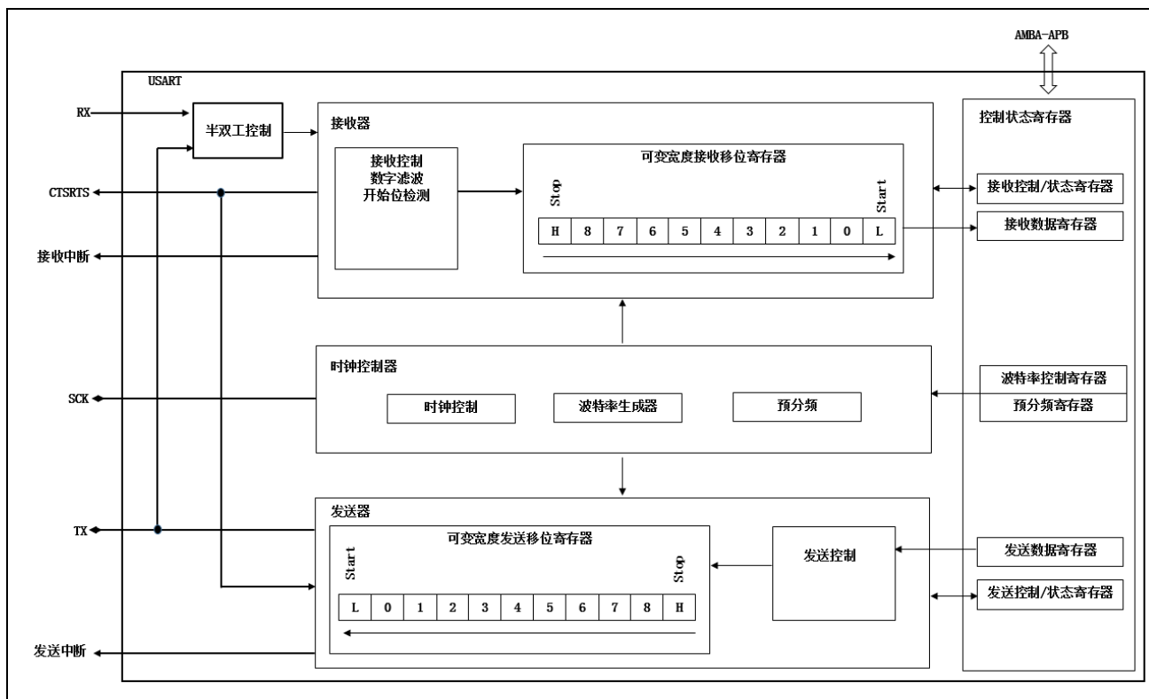
图 22-1 USART 系统框图
