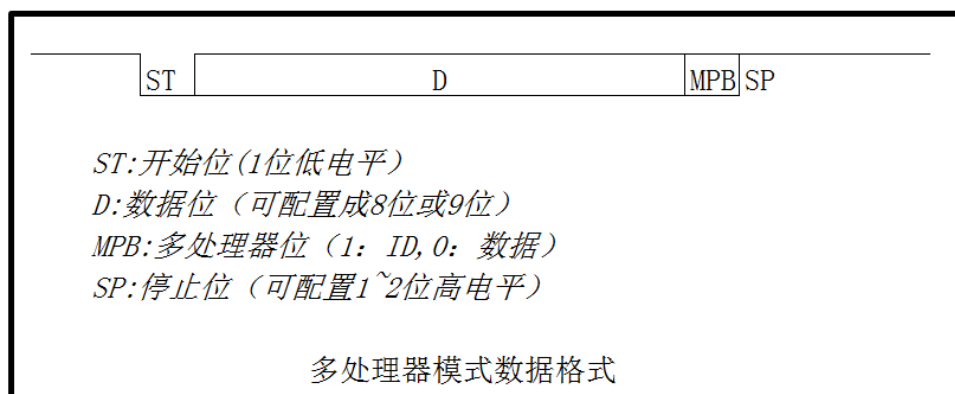
图 22-9 多处理器模式数据格式
