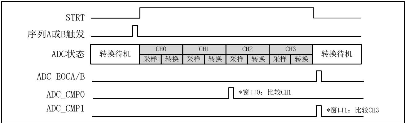
图 14-11 ADC 中断和事件输出时序
