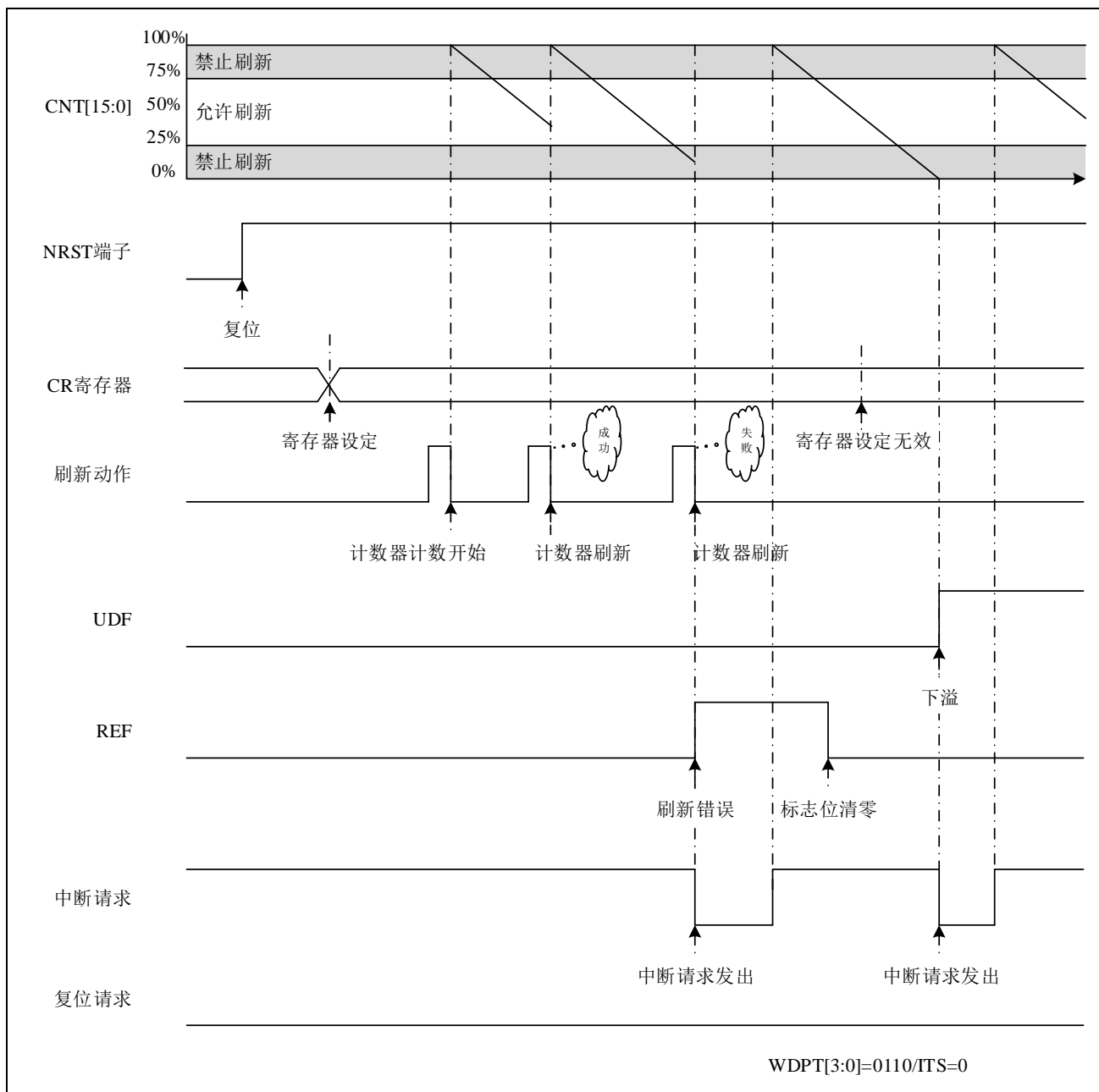
图 21-5 计数器刷新动作例
