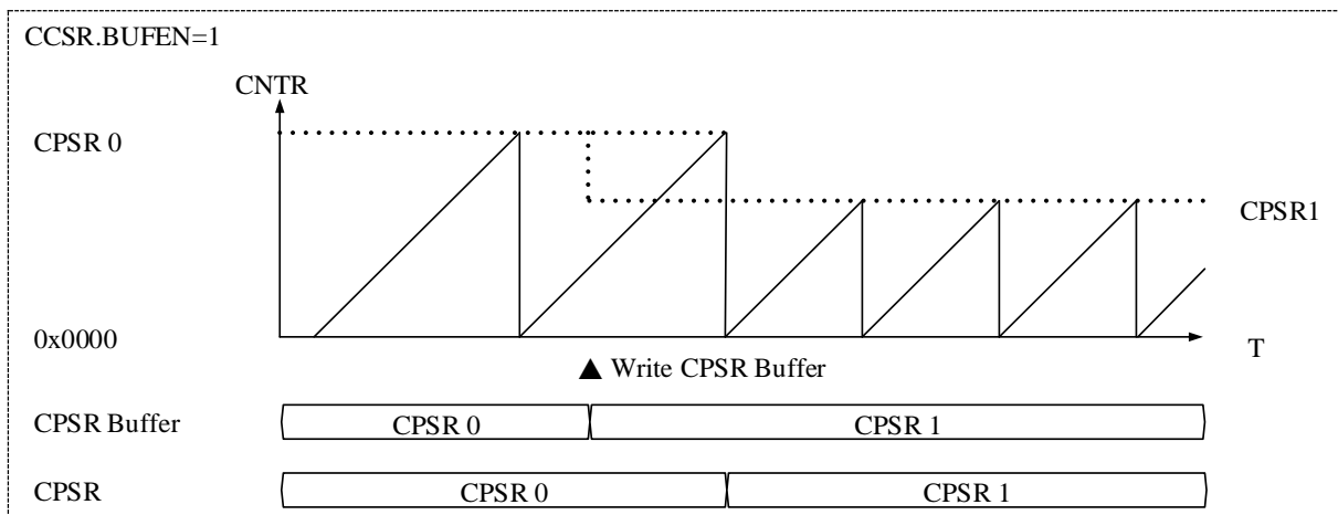
图 15-9 缓存使能时修改锯齿波计数周期
