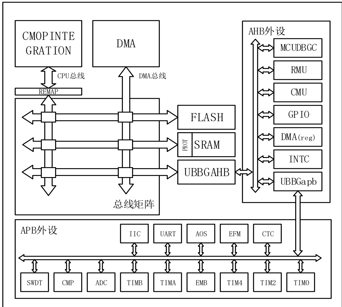
图 2-1 总线架构
