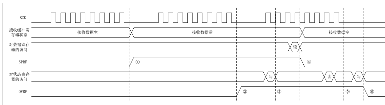
图 24-10 过载错误处理
