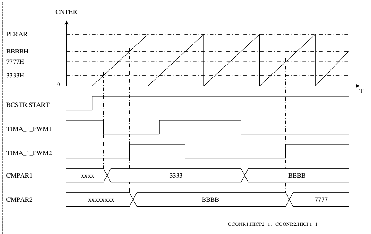
图 18-5 捕获输入动作
