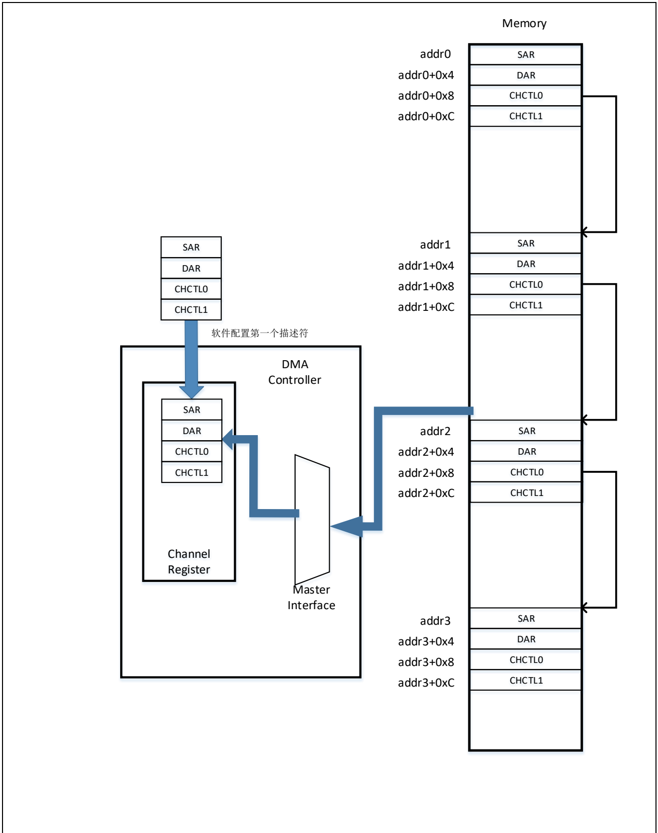
图 11-2 连锁传输示意图
