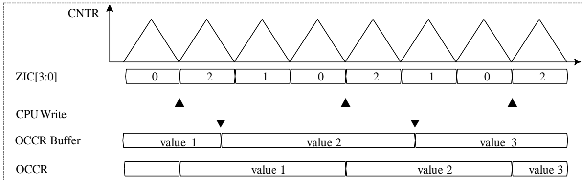
图 15-12 OCCR 缓冲数据传输（周期间隔响应链接使能）
