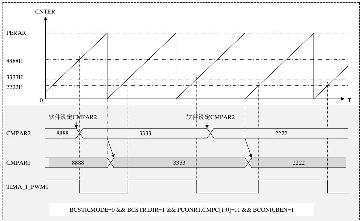
图 18-7 锯齿波模式时缓存动作
