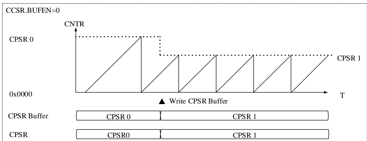
图 15-8 缓存无效时修改锯齿波计数周期
