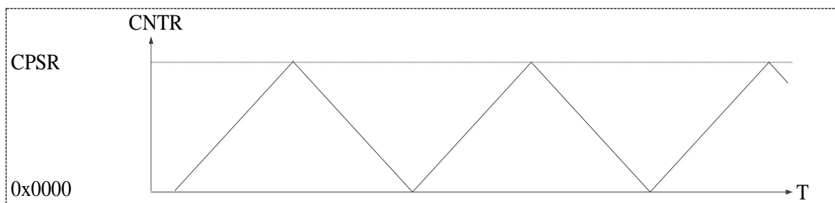
图 15-3 Timer4 三角波波形
