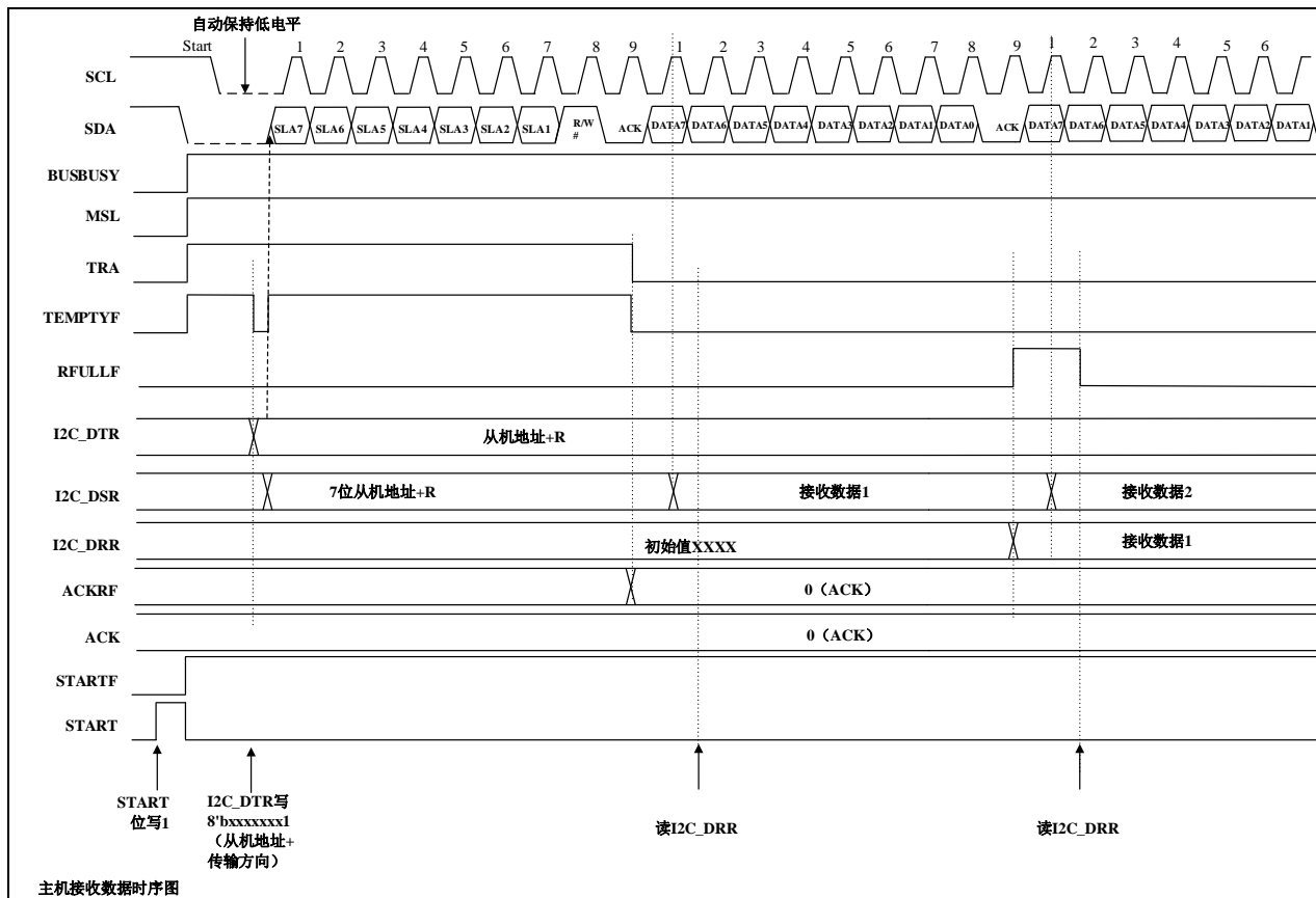
图 23-6 7 位地址格式的主机接收数据的时序图（例）
