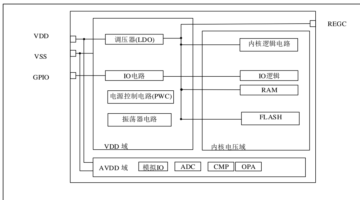
图 5-1 电源构成图
