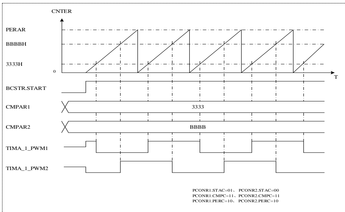
图 18-4 比较输出动作
