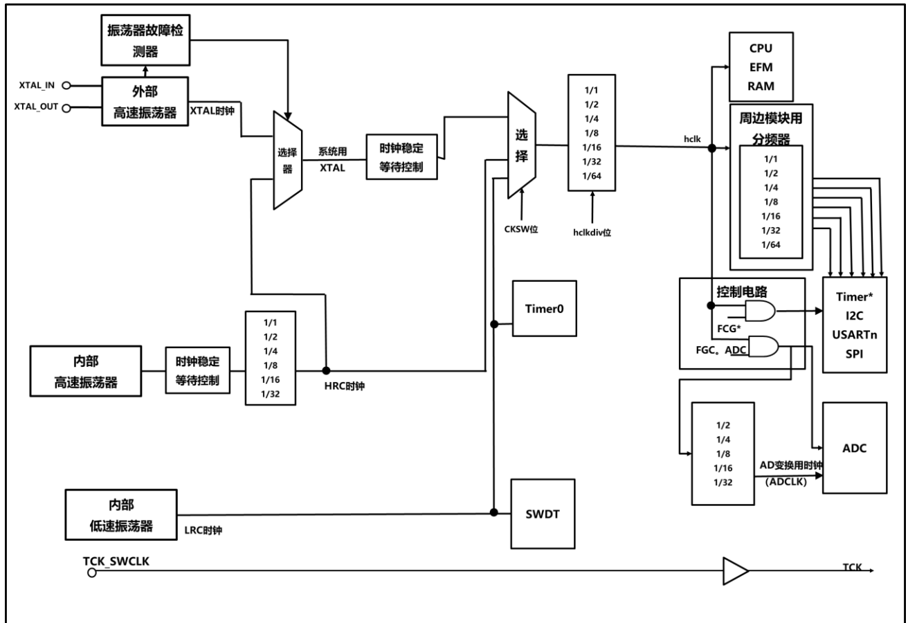
图 4-1 时钟系统框图
