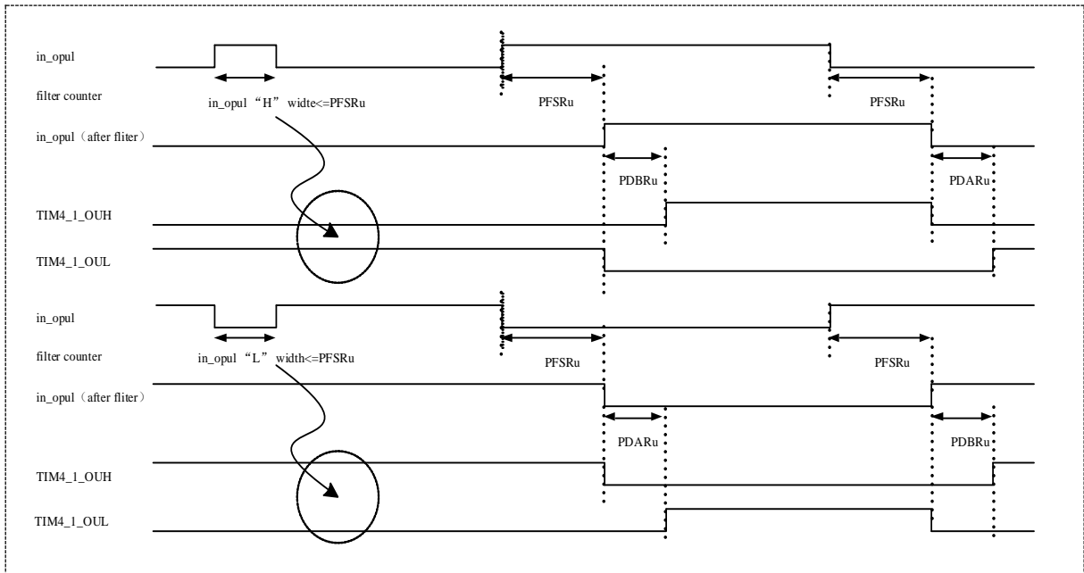
图 15-22 死区定时器滤波模式下的互补 PWM 输出
