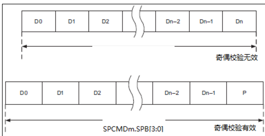
图 24-4 数据格式
