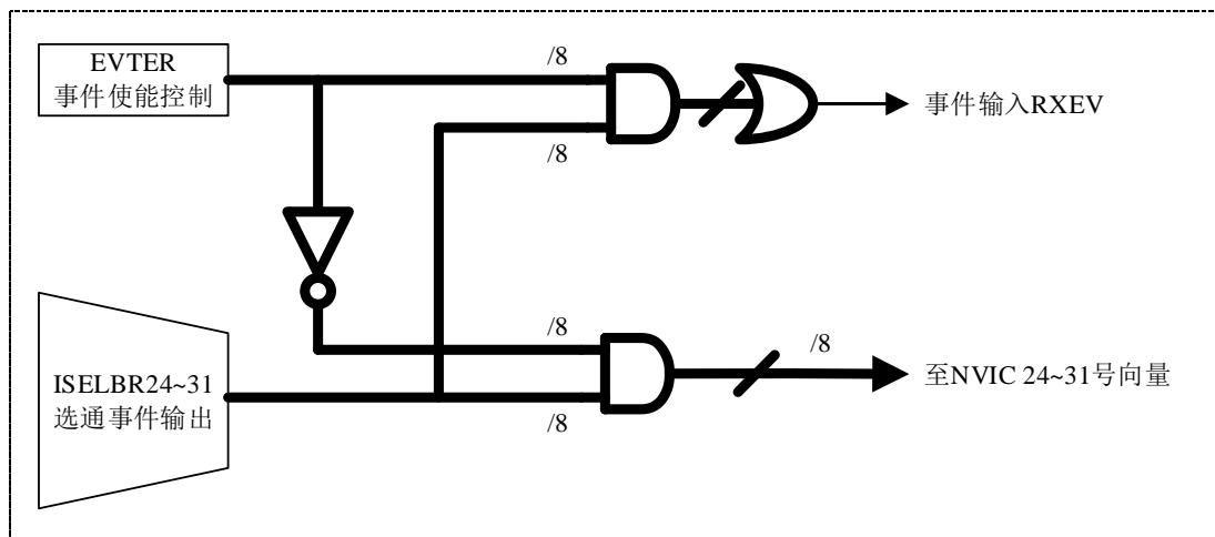
图 10-3 中断事件选择
