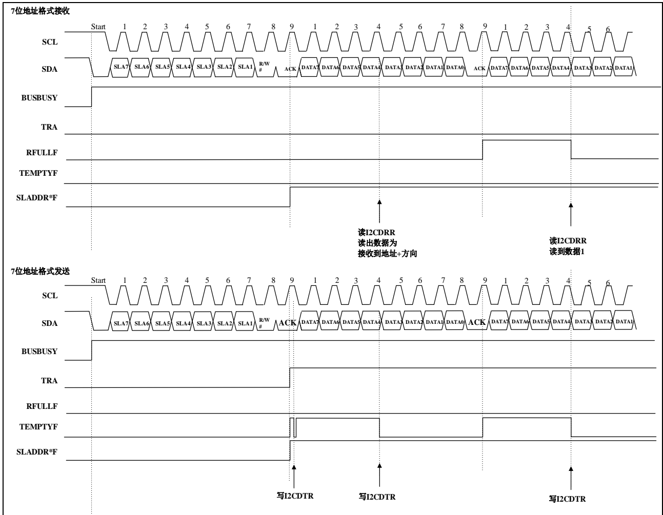
图 23-12 选择 7 位地址格式时的时序
