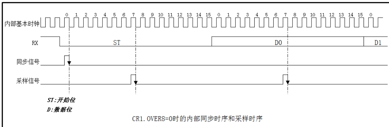
图 22-5 UART 内部同步和采样时序
