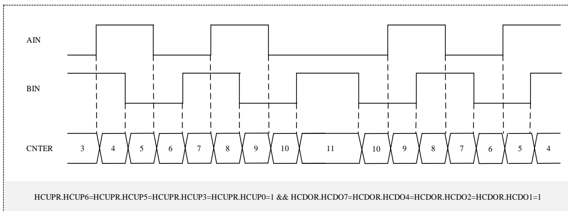
图 18-13 位置计数模式-相位差计数（4 倍计数）
