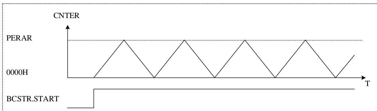
图 18-3 三角波波形
