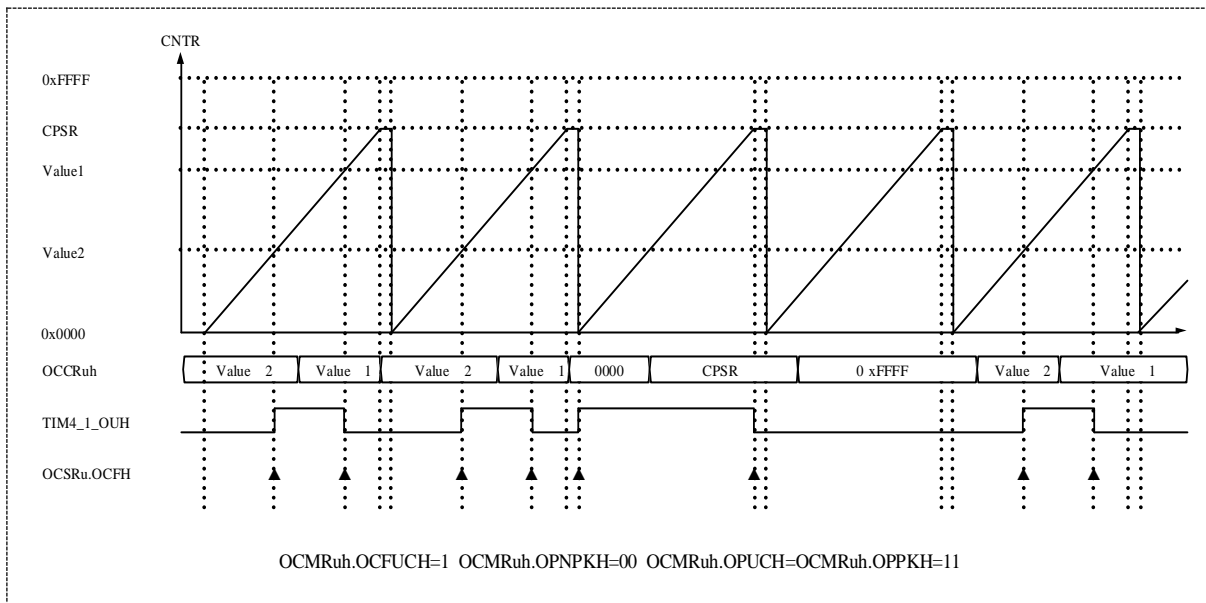
图 15-16 锯齿波独立 PWM 输出例
