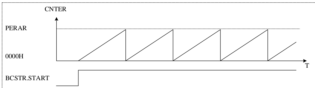
图 18-2 锯齿波波形（递加计数）
