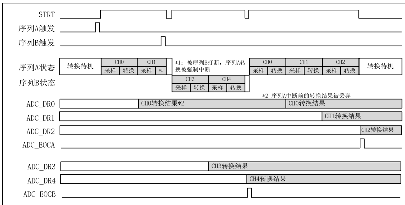
图 14-6 双序列扫描模式 (RSCHSEL=1 序列 A 从第一个通道重新启动)
