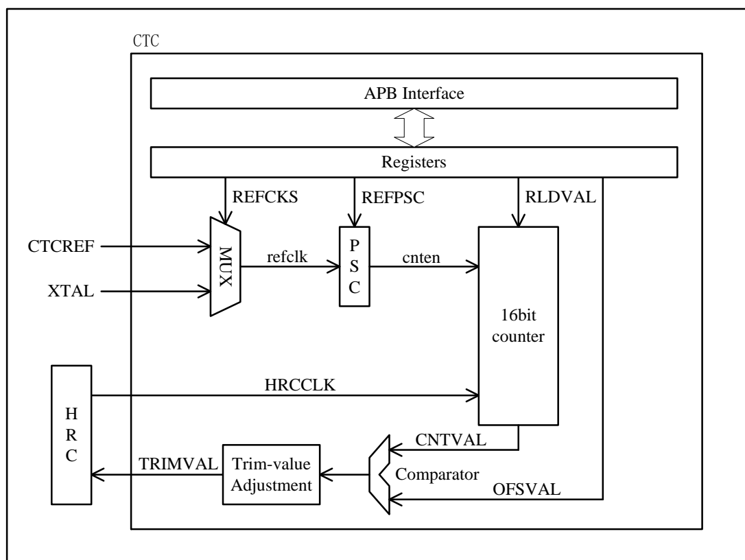
图 12-1 CTC 的基本框图
