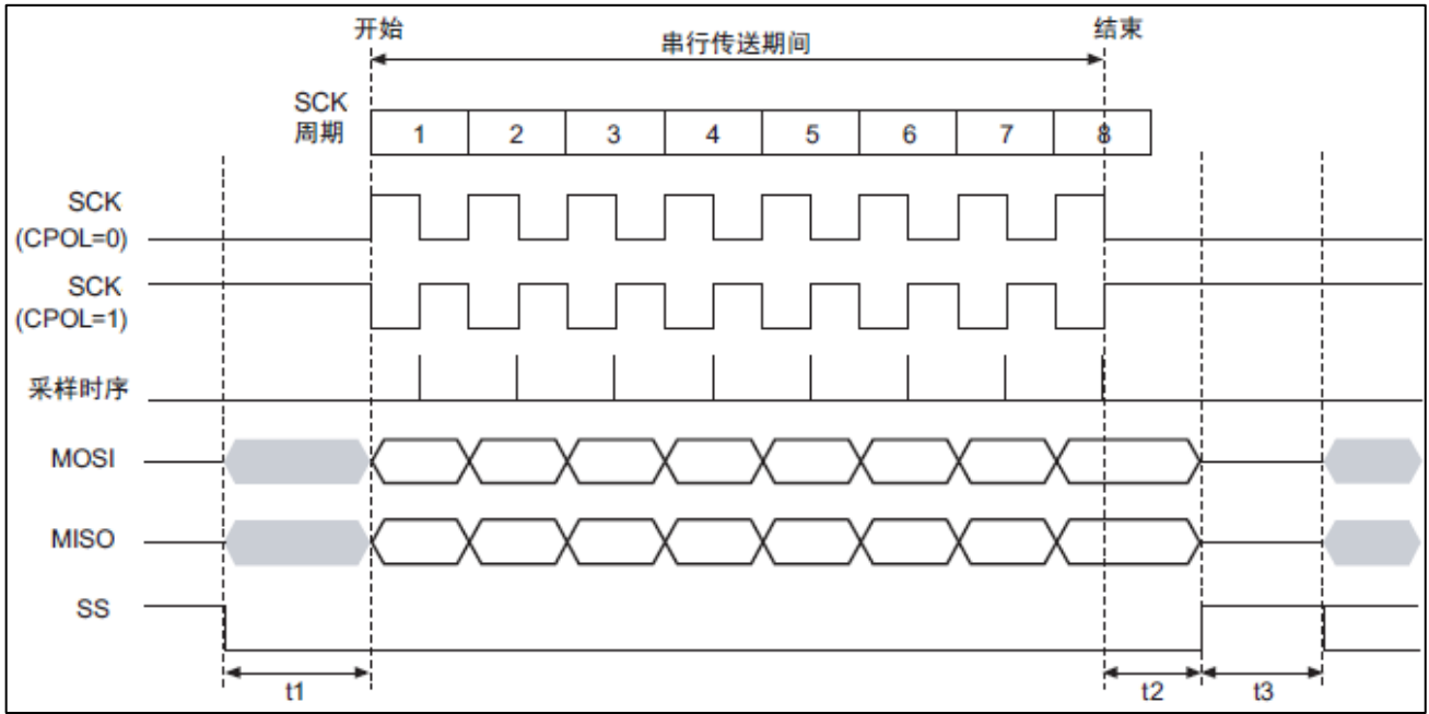
图 24-6 数据传送格式 (CPHA=1)
