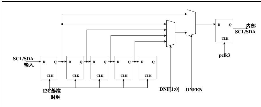
图 23-14 数字滤波电路框图
