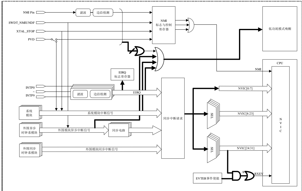
图 10-1 中断系统框图
