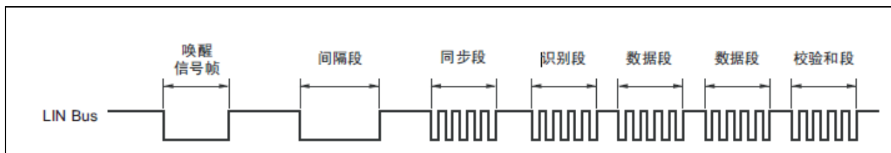
图 22-13 LIN 总线数据行为
