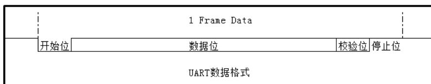
图 22-2 UART 数据格式
