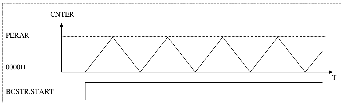
图 17-3 三角波波形
