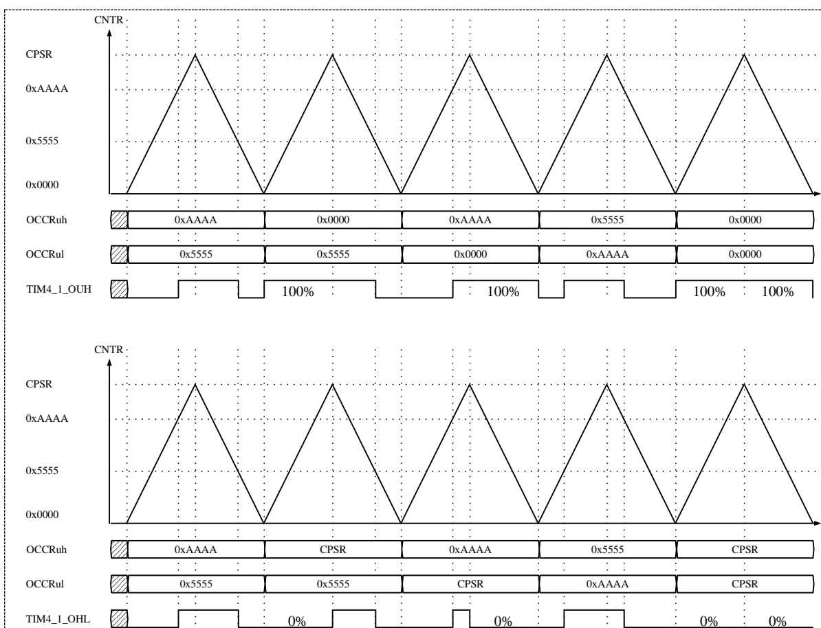
图 15-7 三角波模式波形输出例
