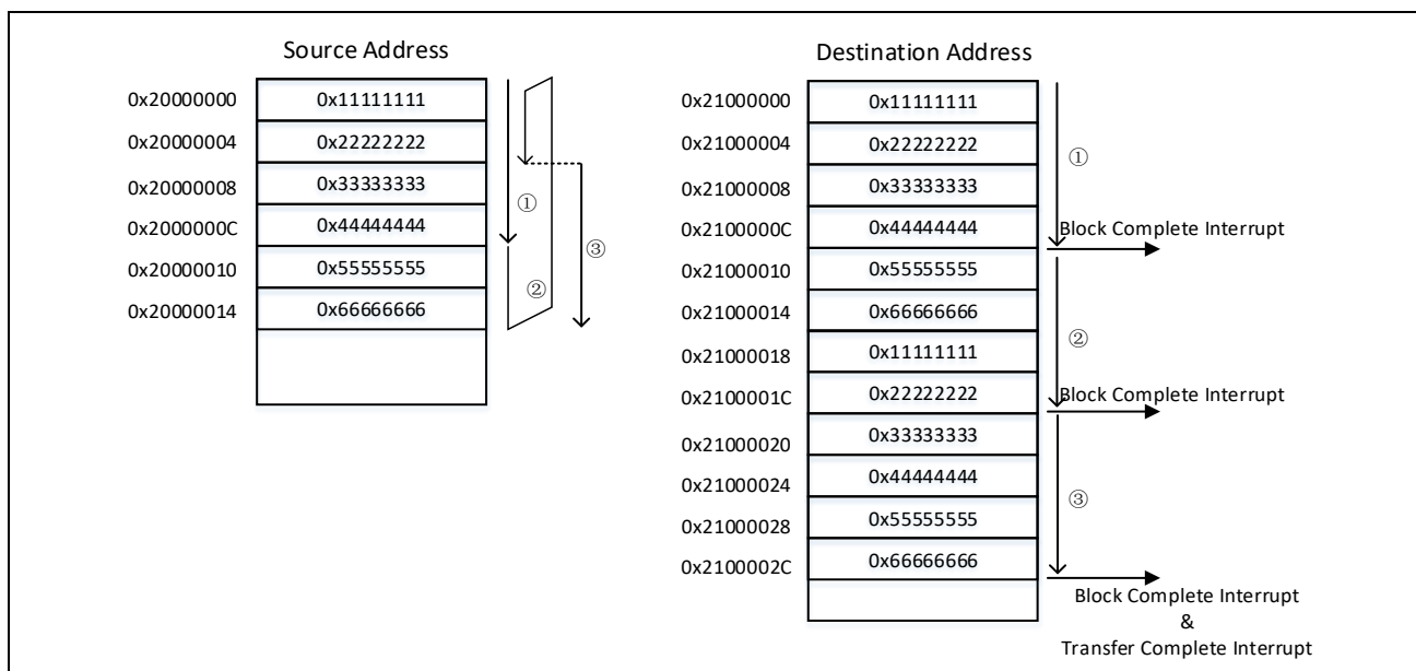
图 11-4 应用例 1: 存储器到存储器传输
