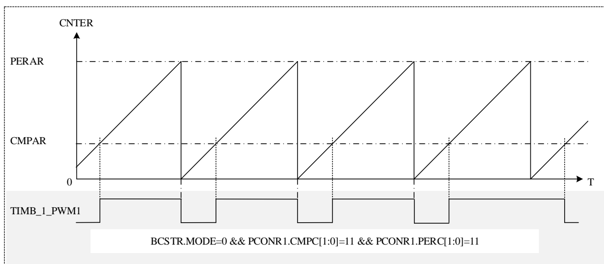
图 17-11 单边对齐 PWM 输出例
