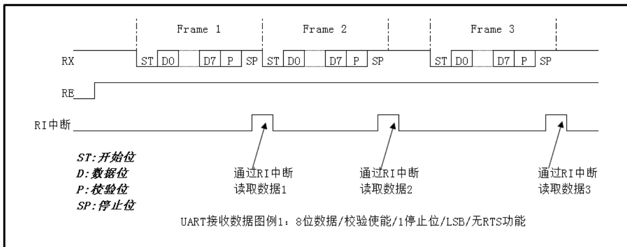
图 22-6 UART 接收数据图例 1
