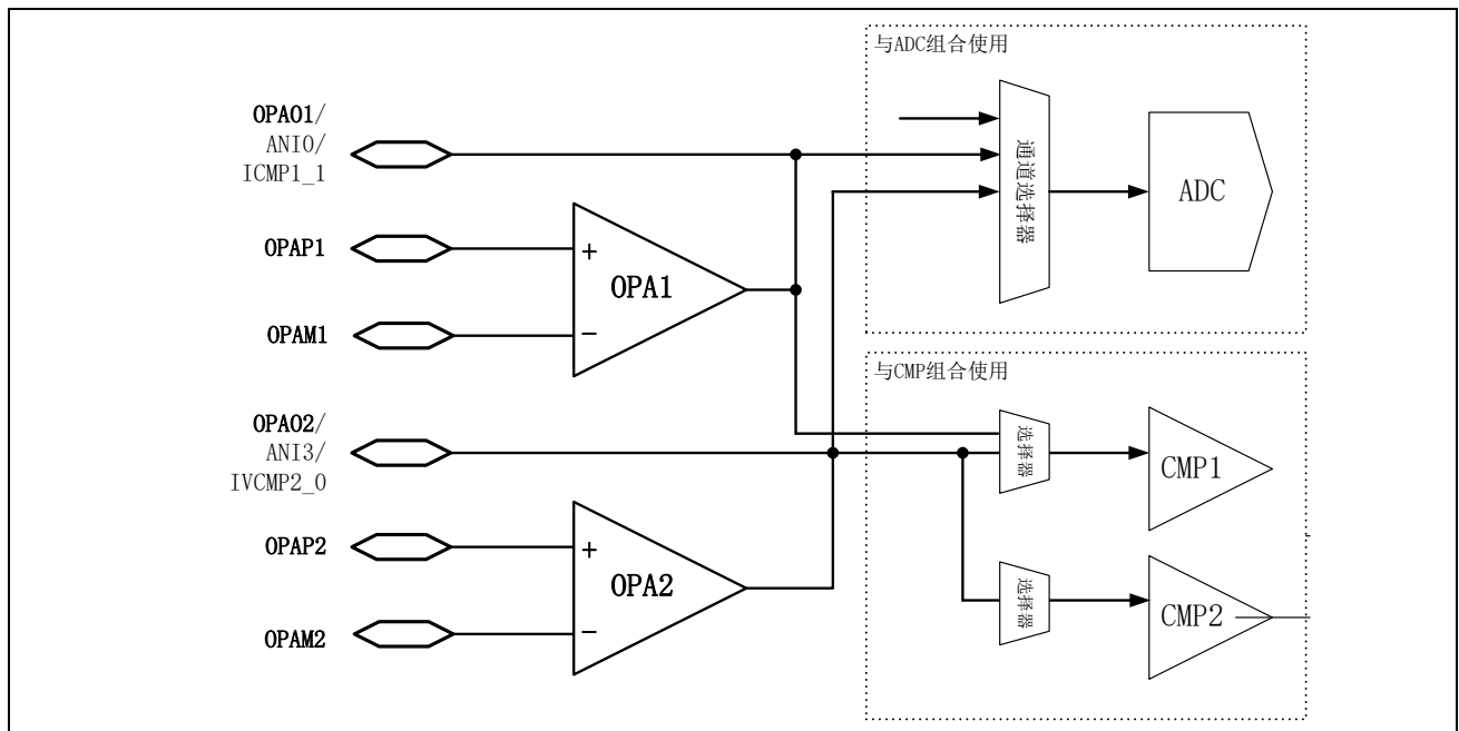
图 14-10 OPA 与 ADC/CMP 组合工作示意图
