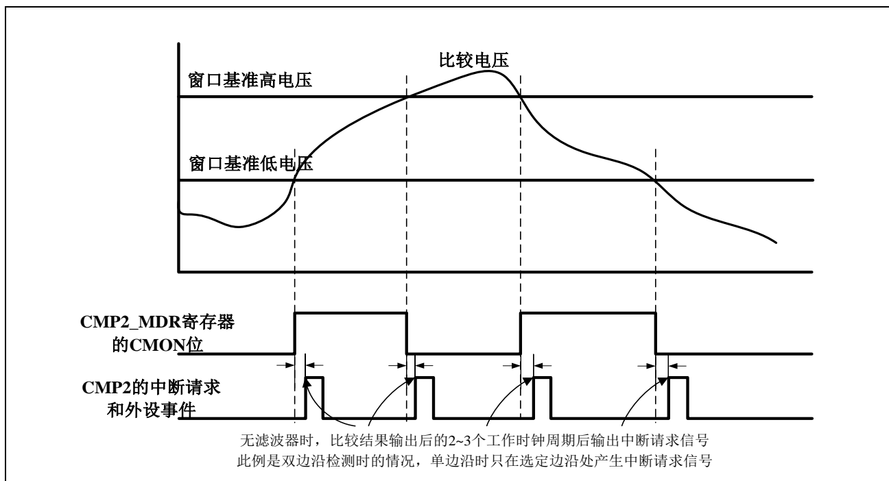
图 13-3 窗口比较模式工作示意图
