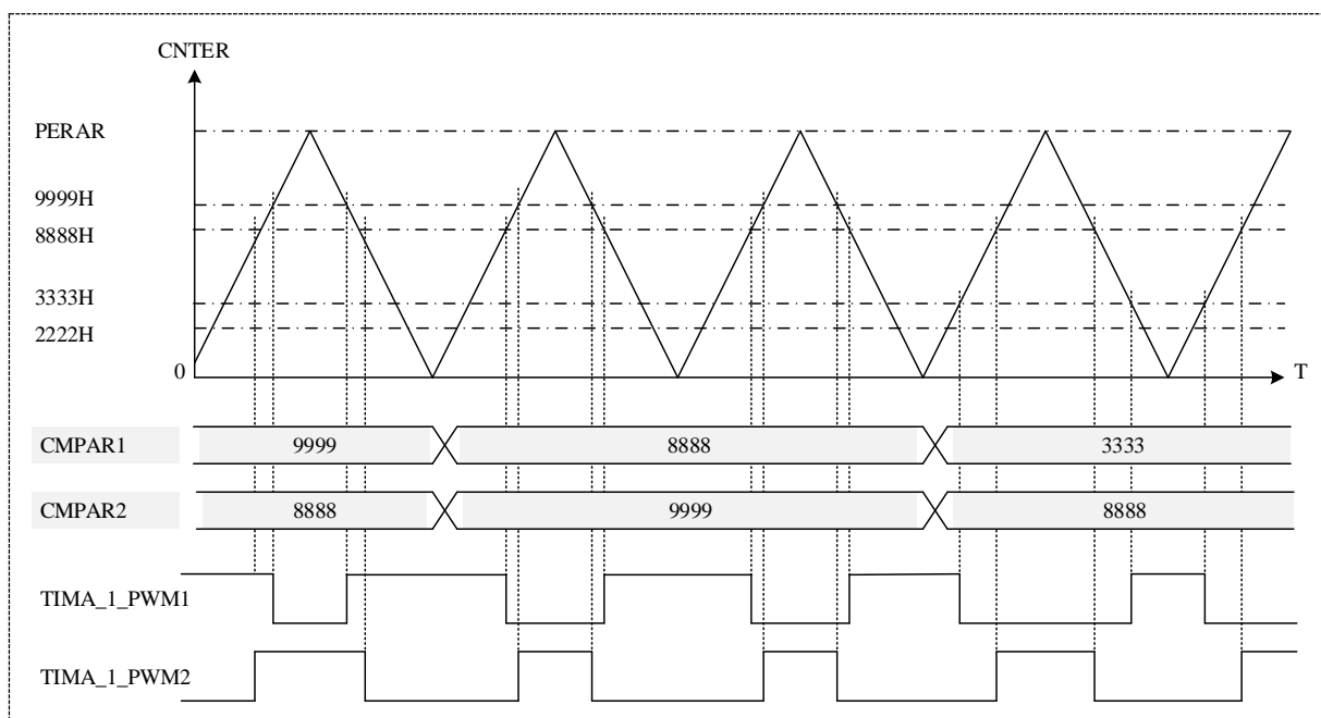
图 18-9 双边对称 PWM 输出例
