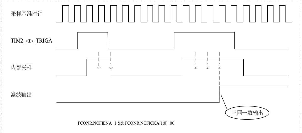
图 19-7 TRIG 输入端口的数字滤波
