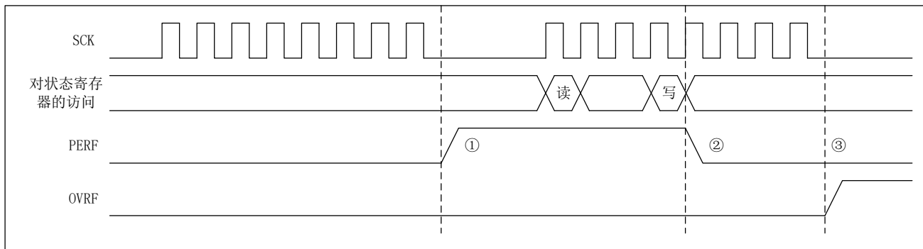
图 24-11 奇偶校验错误
