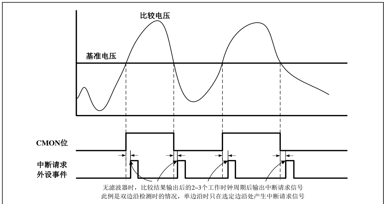
图 13-2 普通比较模式工作示意图
