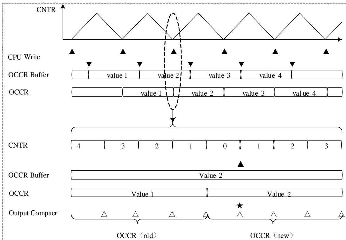
图 15-11 OCCR 缓冲数据传输 (周期间隔响应链接禁止时)
