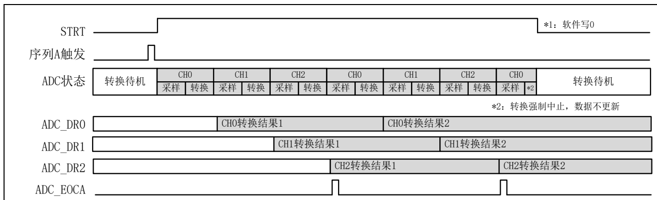
图 14-4 序列 A 连续扫描
