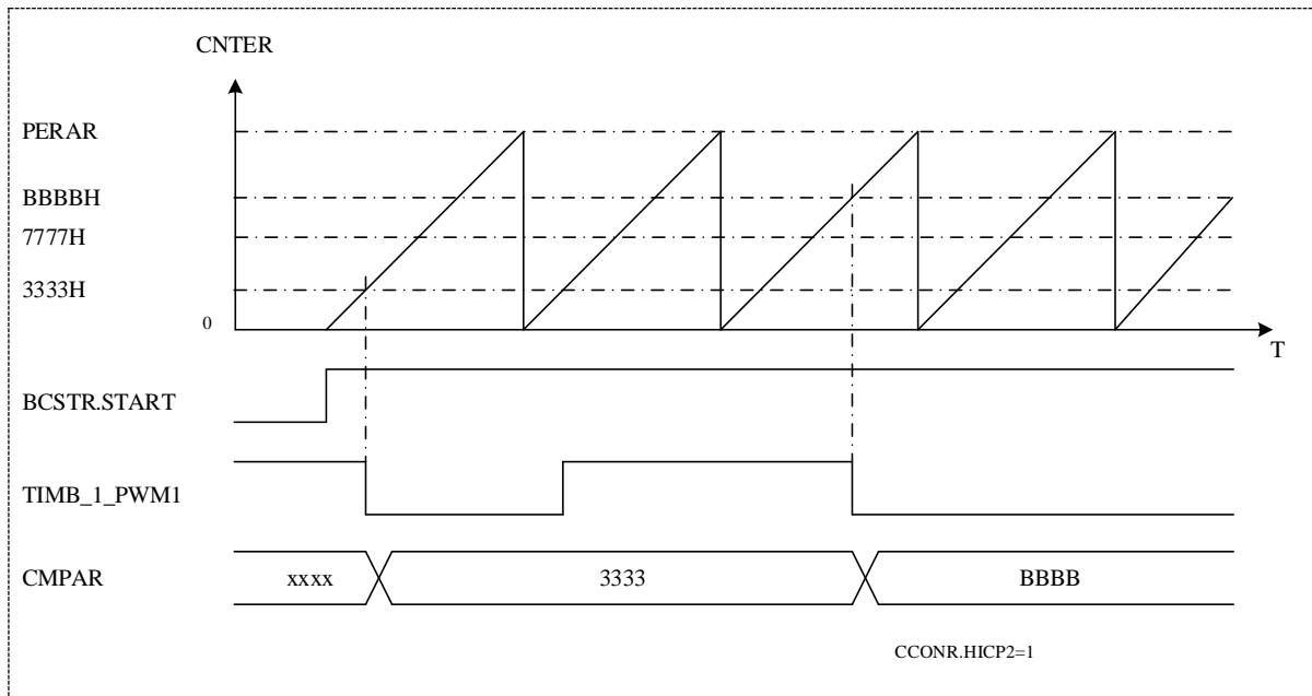
图 17-5 捕获输入动作
