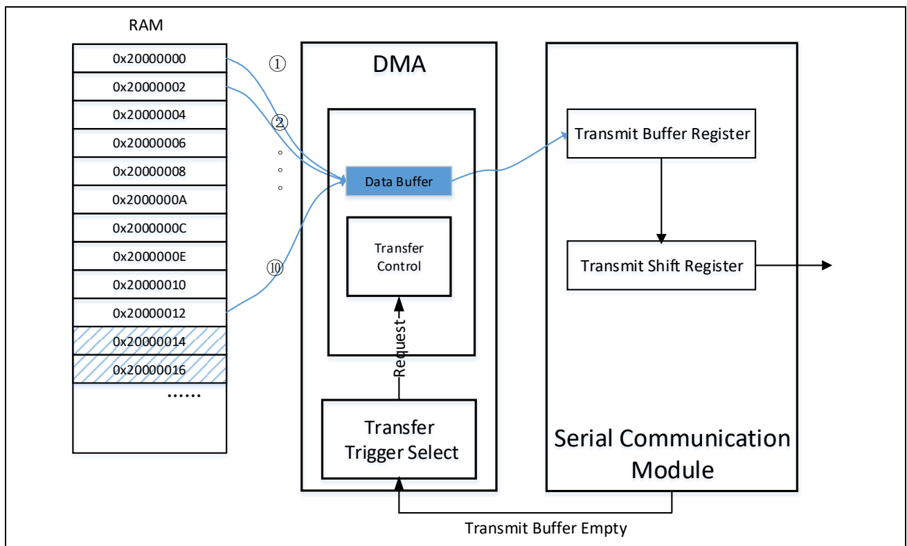
图 11-5 应用例 2：存储器到外围电路的传输
