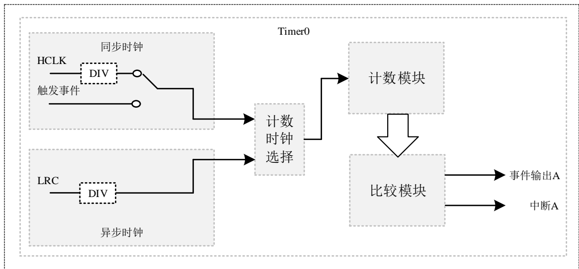
图 20-1 Timer0 基本框图
