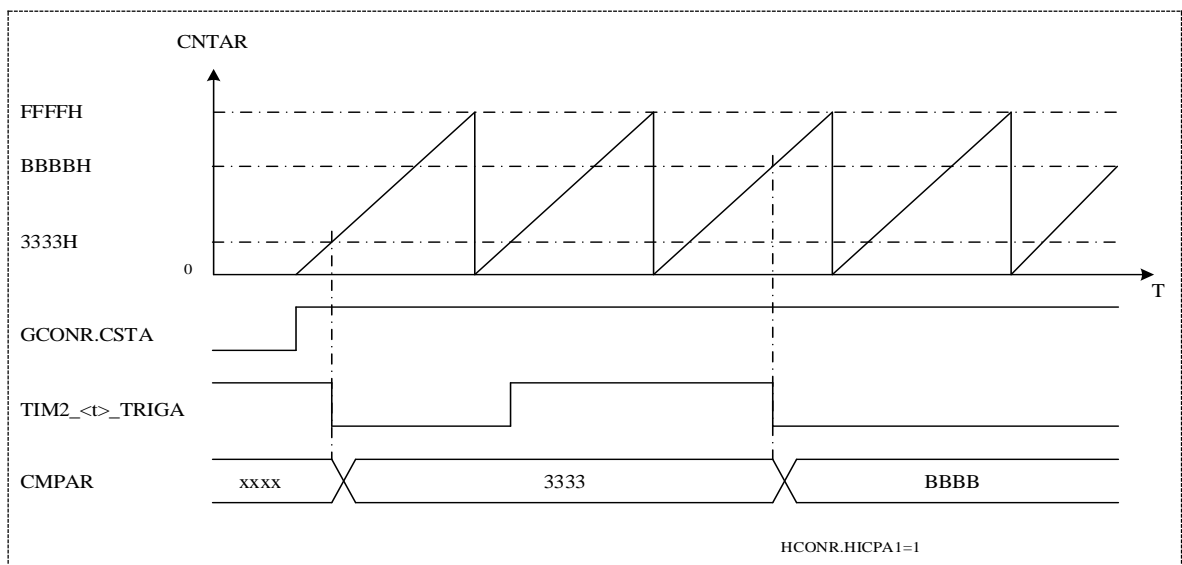
图 19-4 捕获输入动作
