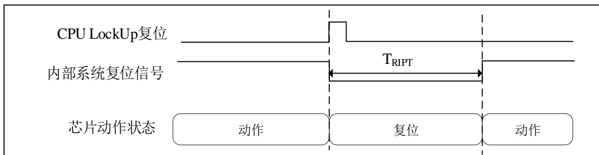
图 3-7 M0+ Lockup 复位
