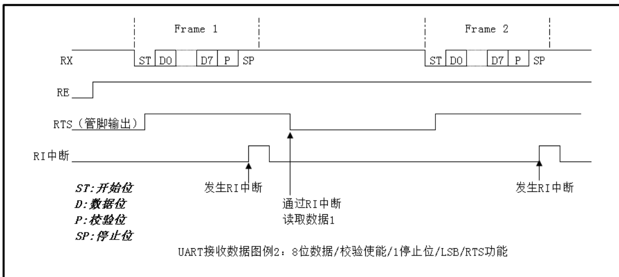
图 22-7 UART 接收数据图例 2
