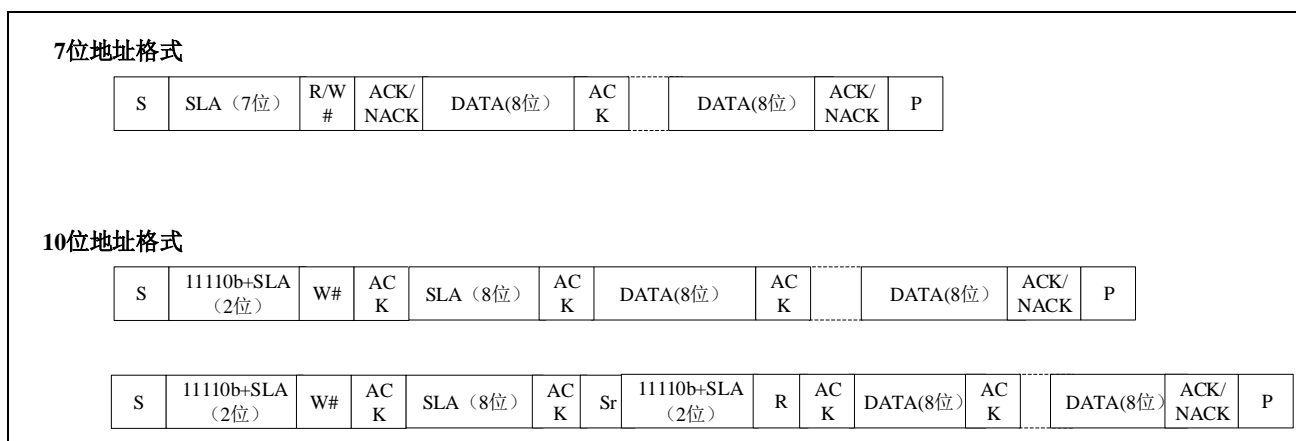
图 23-4 I 2 C 总线的数据格式
