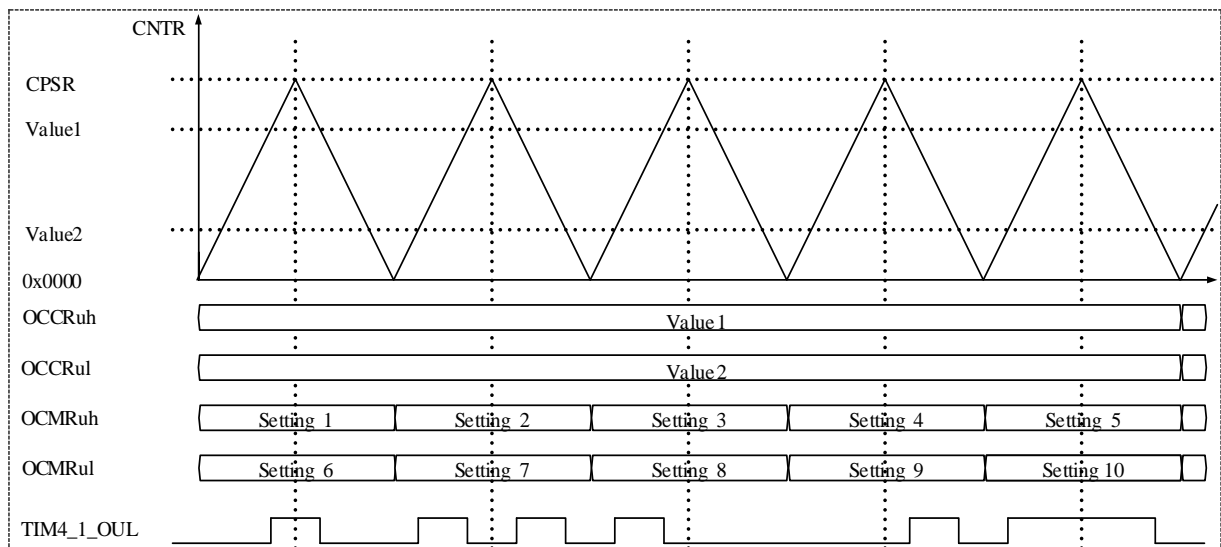
图 15-13 输出比较缓冲数据传输 (OCMR 缓冲使能)
