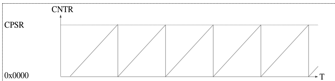
图 15-2 Timer4 锯齿波波形
