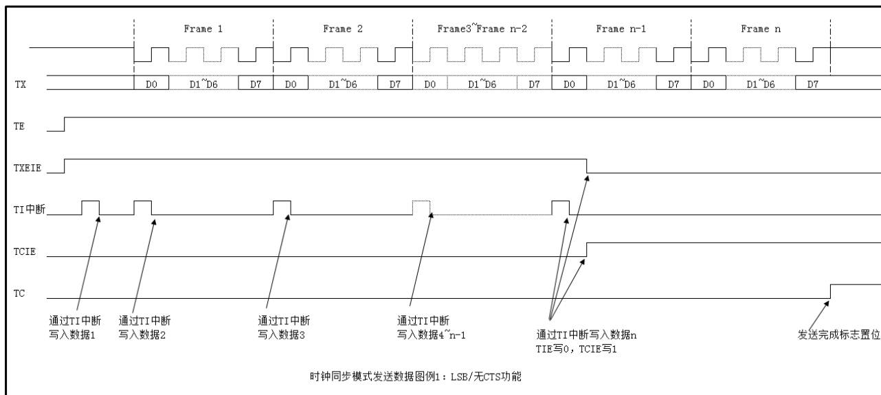
图 22-15 时钟同步模式发送数据图例 1
