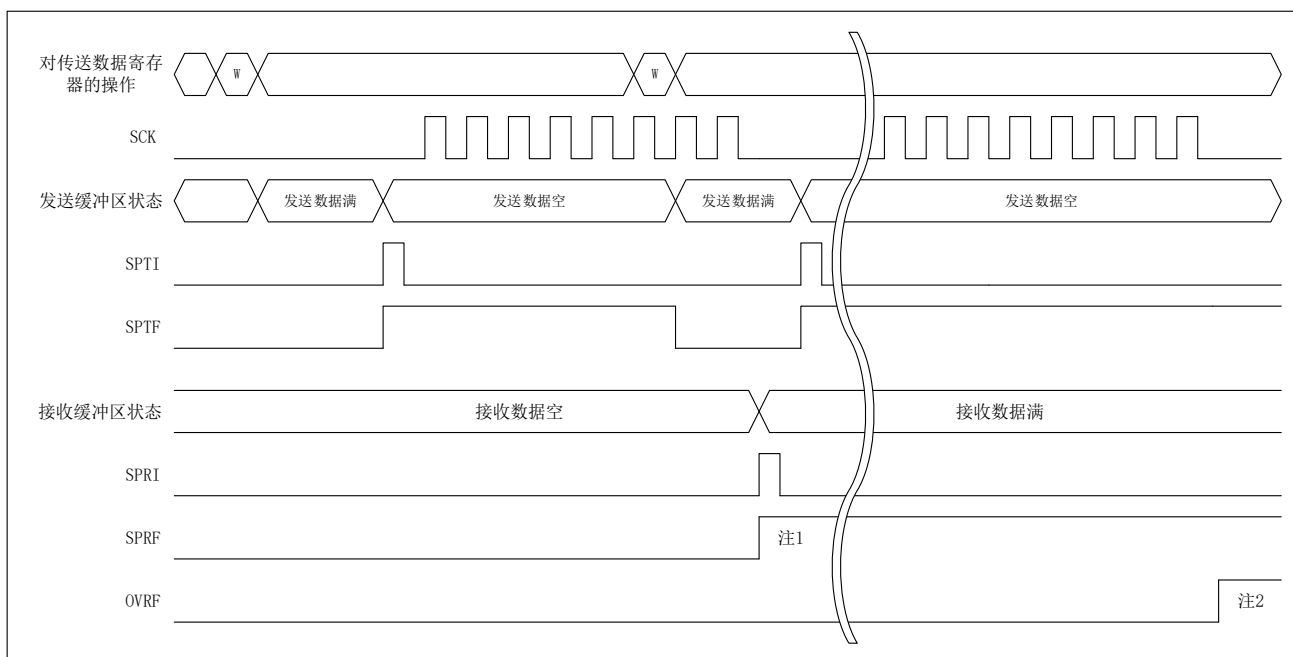
图 24-7 全双工同步串行通信
