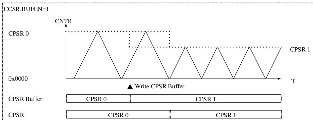
图 15-10 缓存使能时修改三角波计数周期
