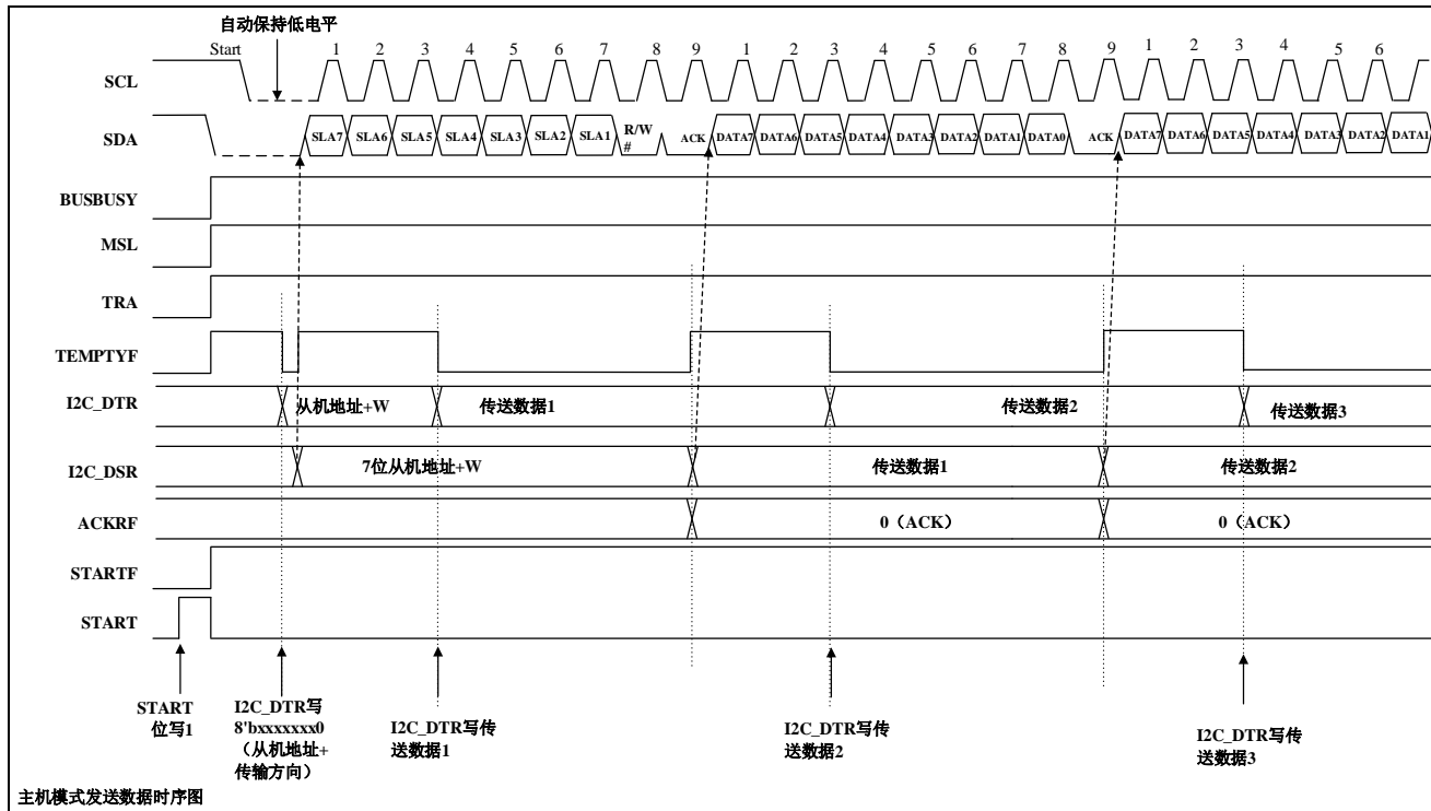
图 23-5 7 位地址格式的主机发送数据时序图（例）
