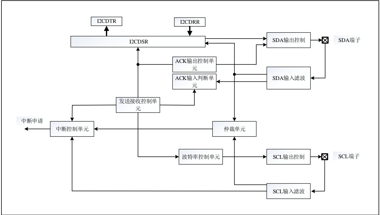
图 23-1 I 2 C 系统框图
