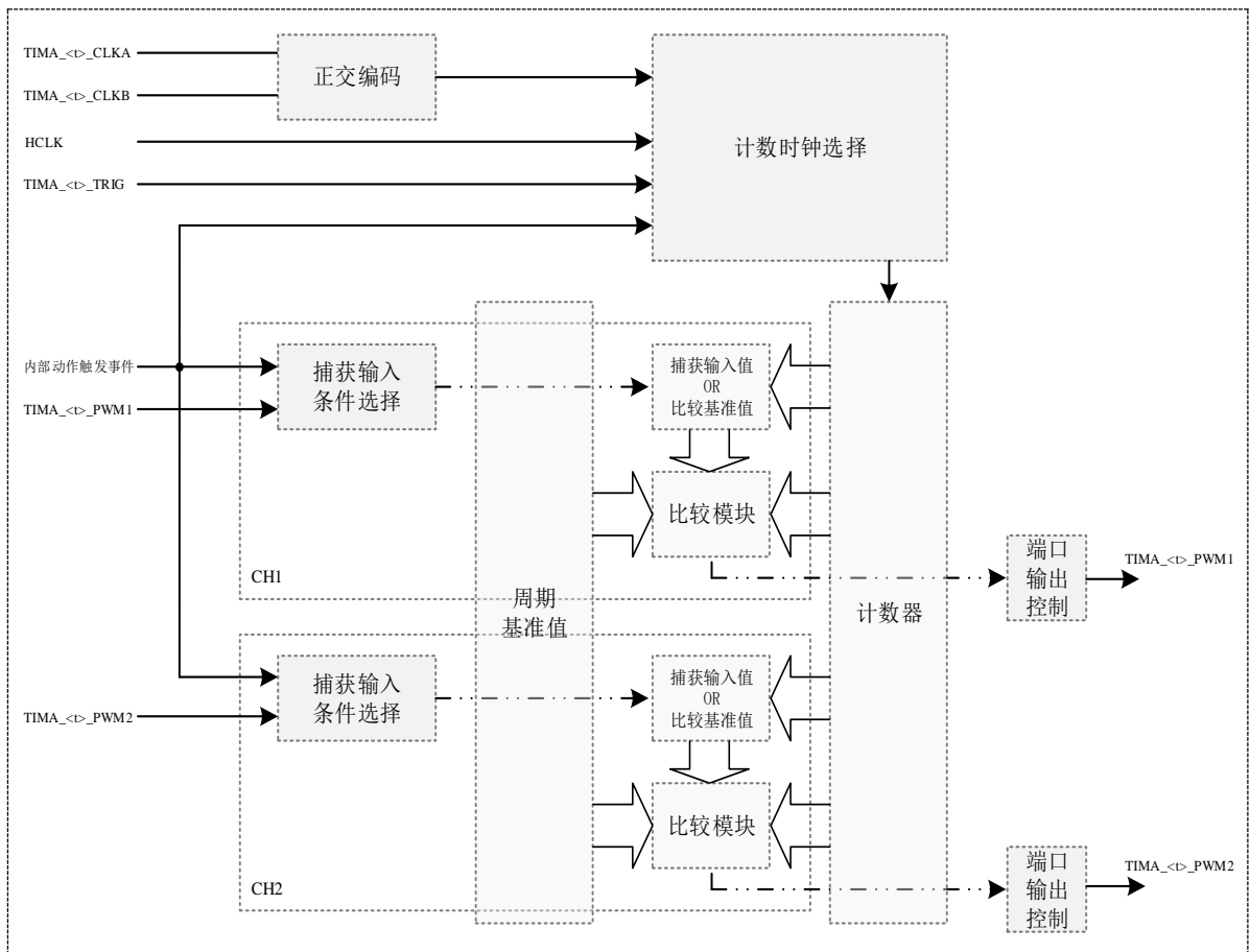
图 18-1 TimerA 基本框图
