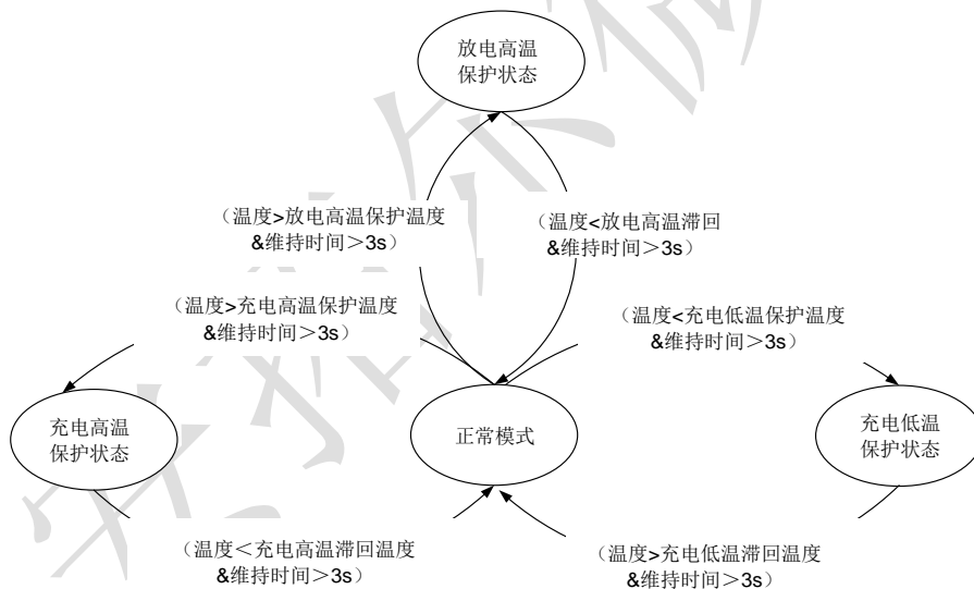
图 9 温度保护状态转移图
