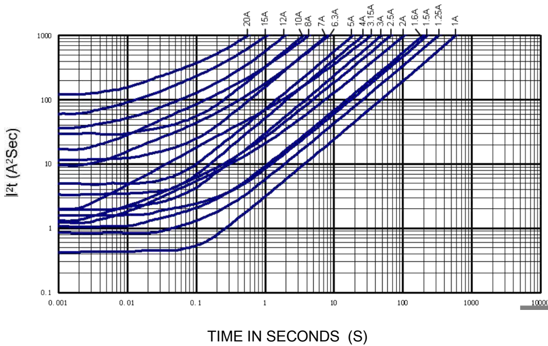
8-4 I 2 t-t 图/CHARACTERISTICS DIAGRAM(I 2 t-t)
