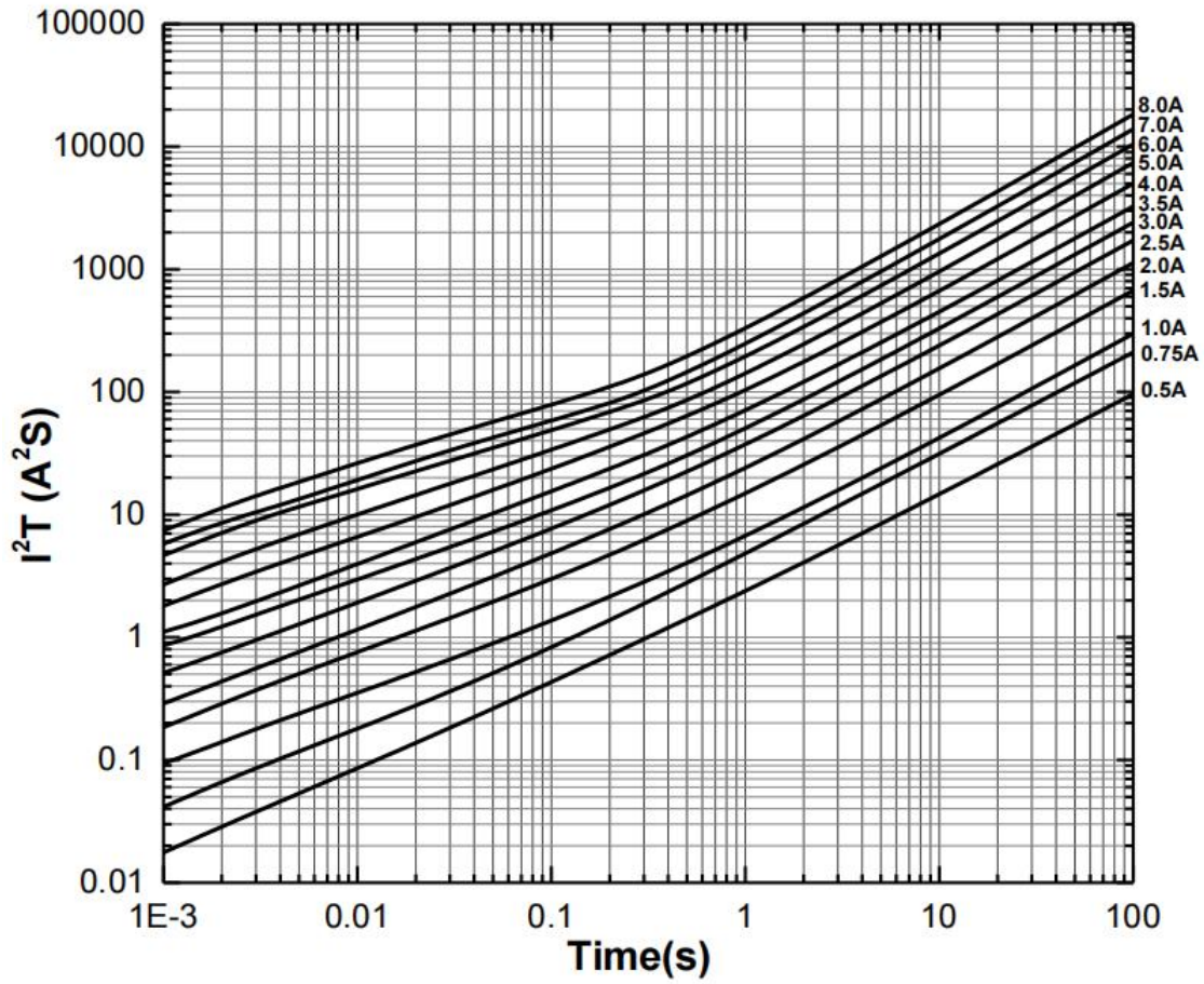
5-3 时间 T — I^2T 特性曲线/Time- I^2T Curve:
