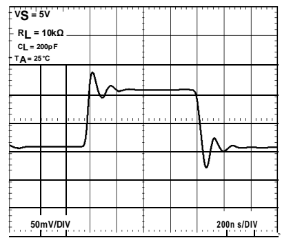
图45. 小信号瞬态响应
