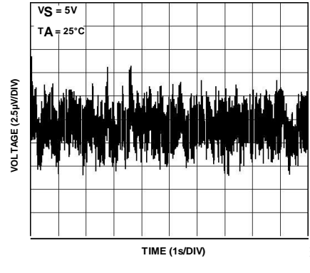
图44. 0.1 Hz 至 10 Hz 输入电压噪声
