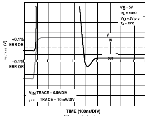
图 51. 建立时间
