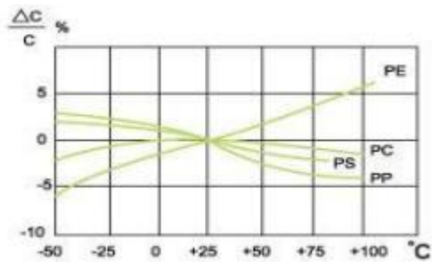
容量变化率与温度的关系
