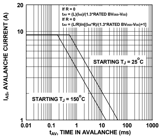
图 12. 非箝位感性开关特性
