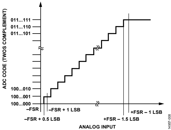
图30. ADC理想传输函数 (FSR表示满量程范围)
