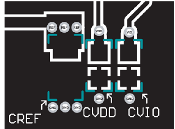
图63. AD4003布局布线示例 (底层)
