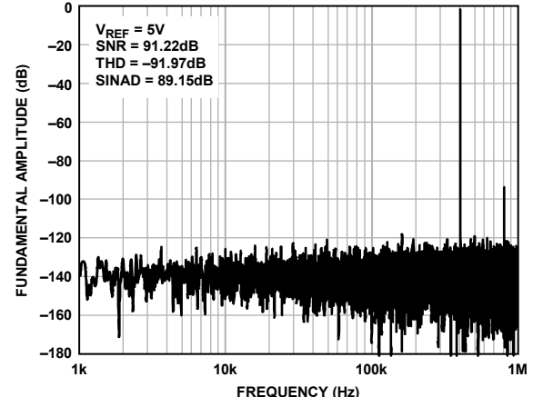
图16. 400 kHz、 -0.5\text{ dBFS} 输入音FFT, 宽视图
