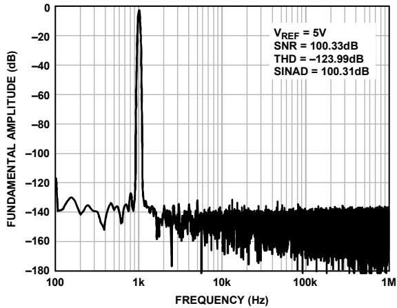
图12. 1 kHz、 -0.5\text{ dBFS} 输入音FFT, 宽视图, V_{REF} = 5\text{ V}
