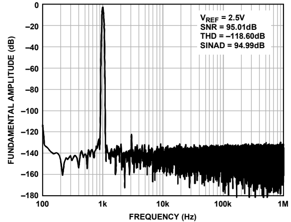
图15. 1 kHz、 -0.5\text{ dBFS} 输入音FFT, 宽视图, V_{REF} = 2.5\text{ V}
