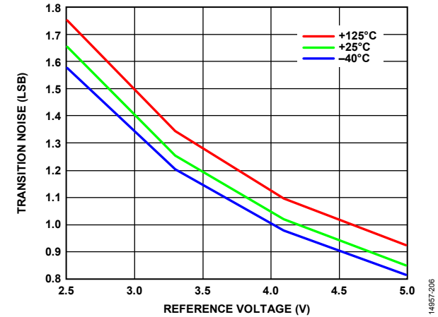
图10. 转换噪声与基准电压的关系
