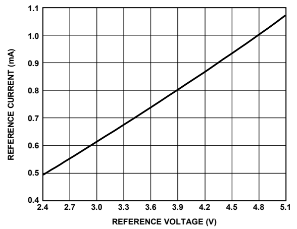
图21. 基准电流与基准电压的关系
