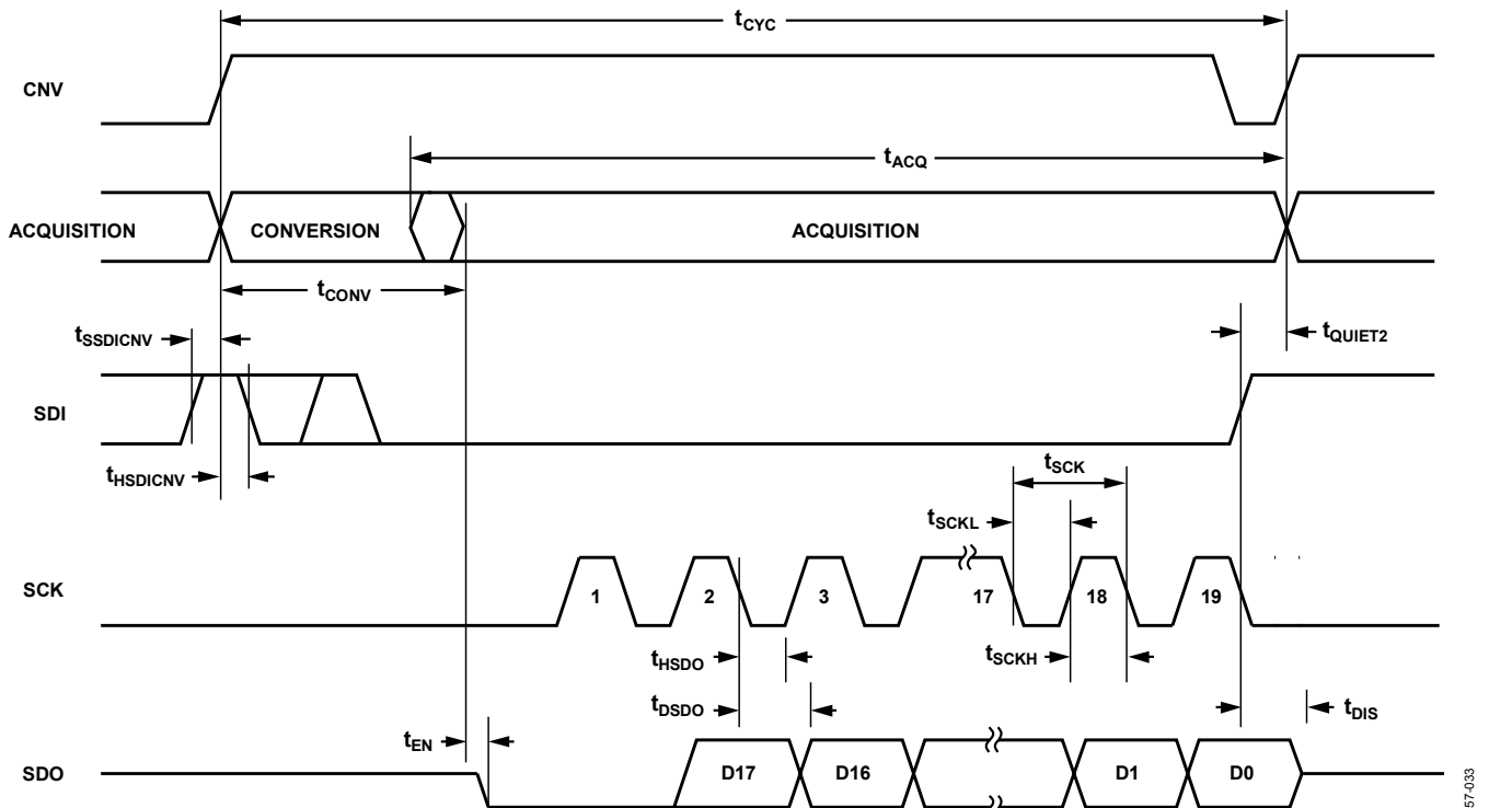
图59. \overline{\text{CS}} 模式（四线式且有繁忙指示）串行接口时序图
