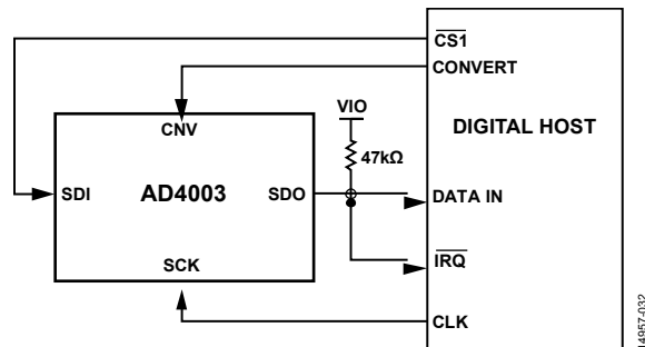
图58. \overline{\text{CS}} 模式（四线式且有繁忙指示）连接图
