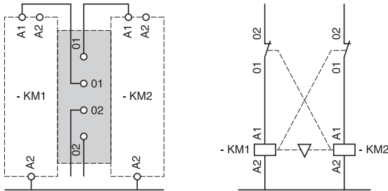
低速 / 高速配线组件、螺钉夹紧端子 LAD9PV/GV
