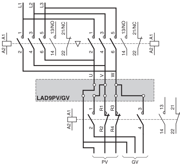
低速 / 高速配线组件、螺钉夹紧端子 LAD9PV/GV
