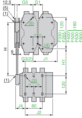
装配 B
