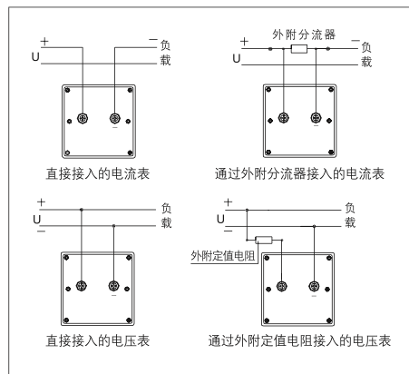
■ 6C2-A、V接线图
