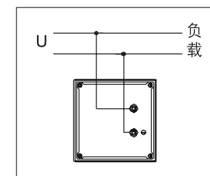
■ 42L6-Hz接线图
