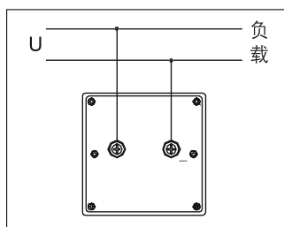
■ 6L2-Hz接线图
