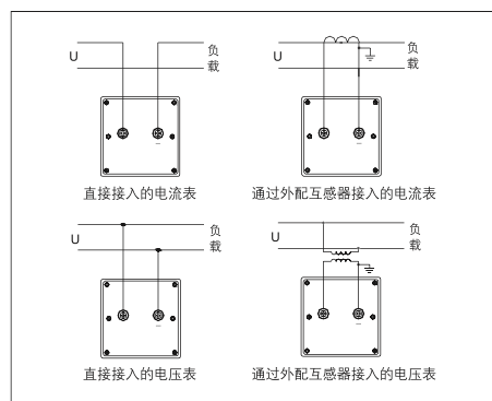
■ 6L2-A、V接线图
