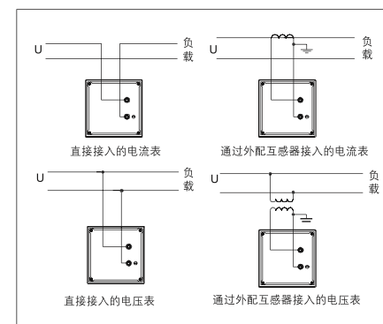
■ 42L6-A、V接线图
