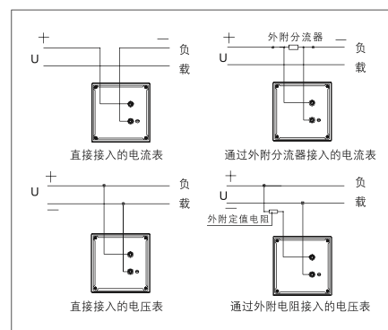
■ 42C3-A、V接线图
