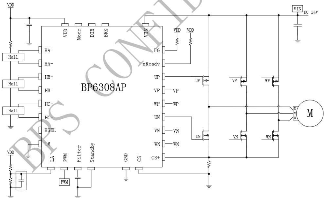
图 1 BP6308AP 典型应用图
