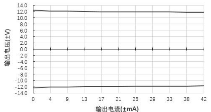
输出电压 VS 负载关系曲线
