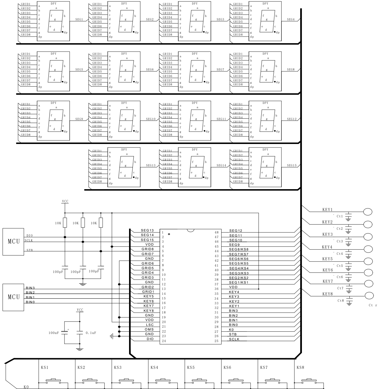
TM1649 驱动共阳数码屏接线电路图:
