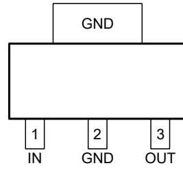
SOT-223-3
