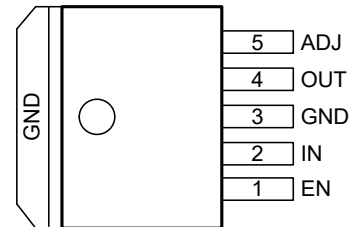
TO-263-5B
