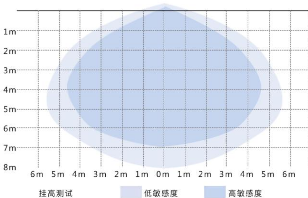
吸顶安装图
