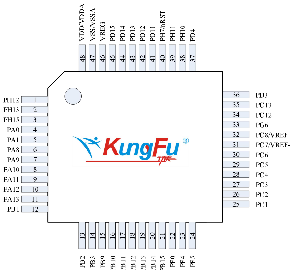
图 2-6 LQFP48
