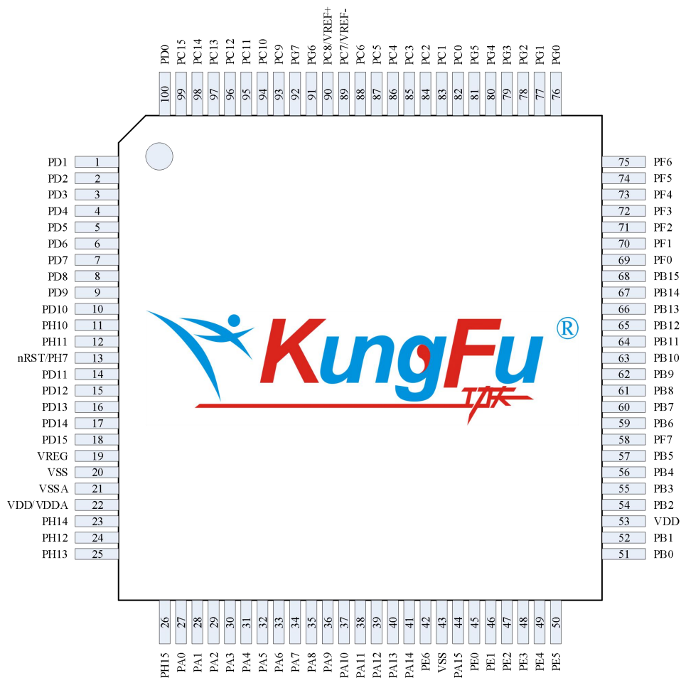
图 2-8 LQFP100
