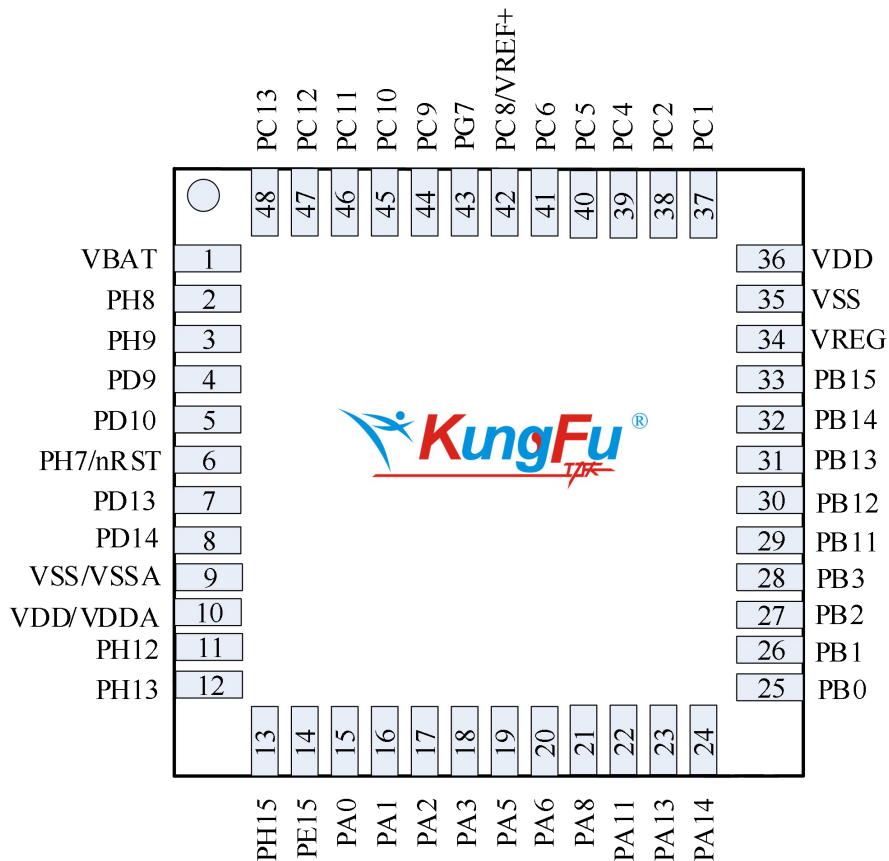
图 2-4 QFPN48
