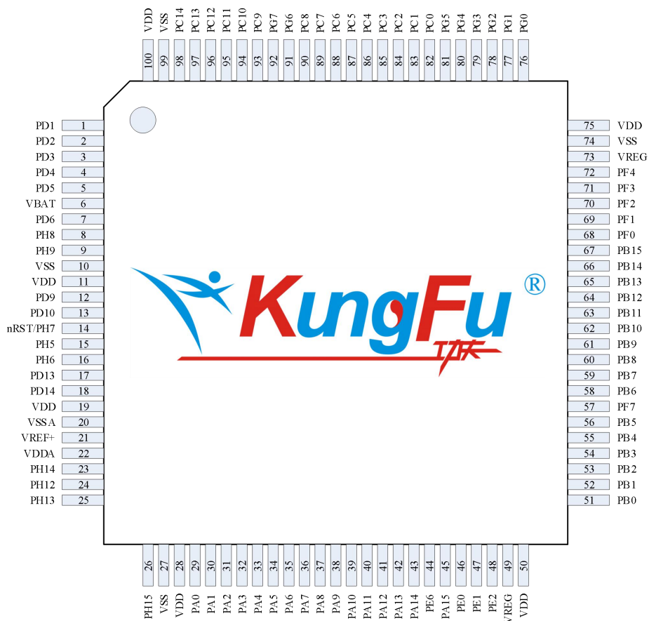
图 2-6 LQFP100
