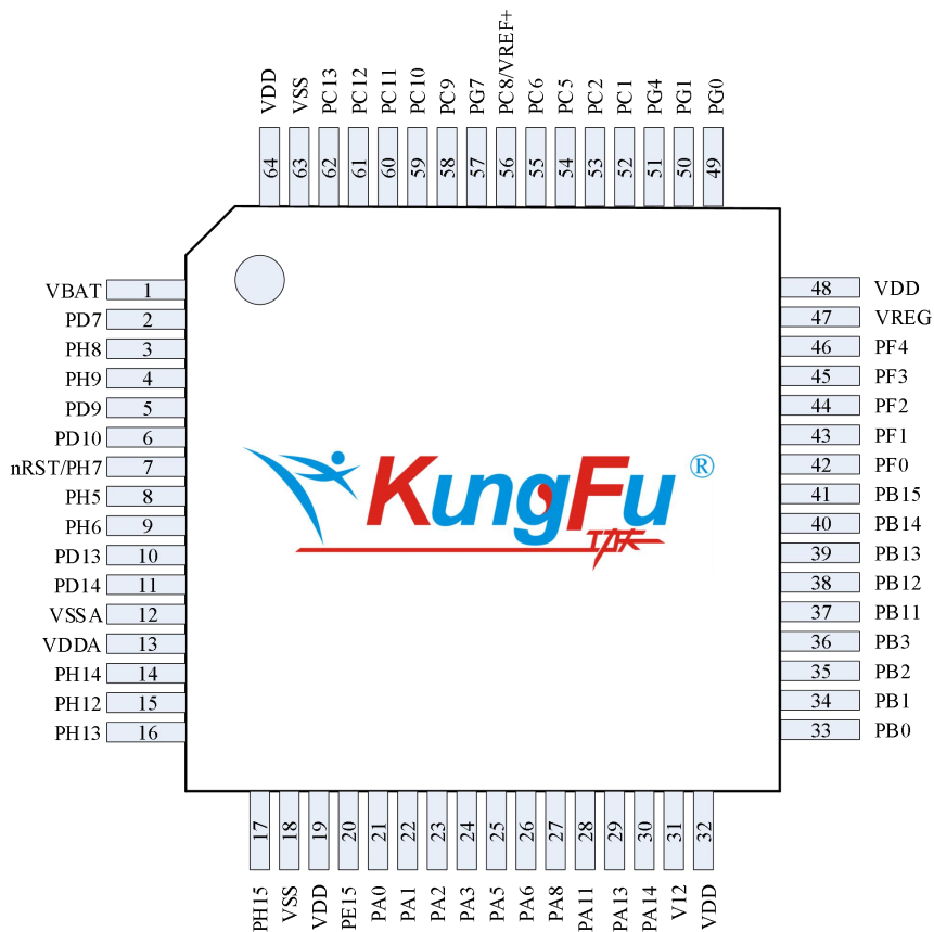
图 2-5 LQFP64
