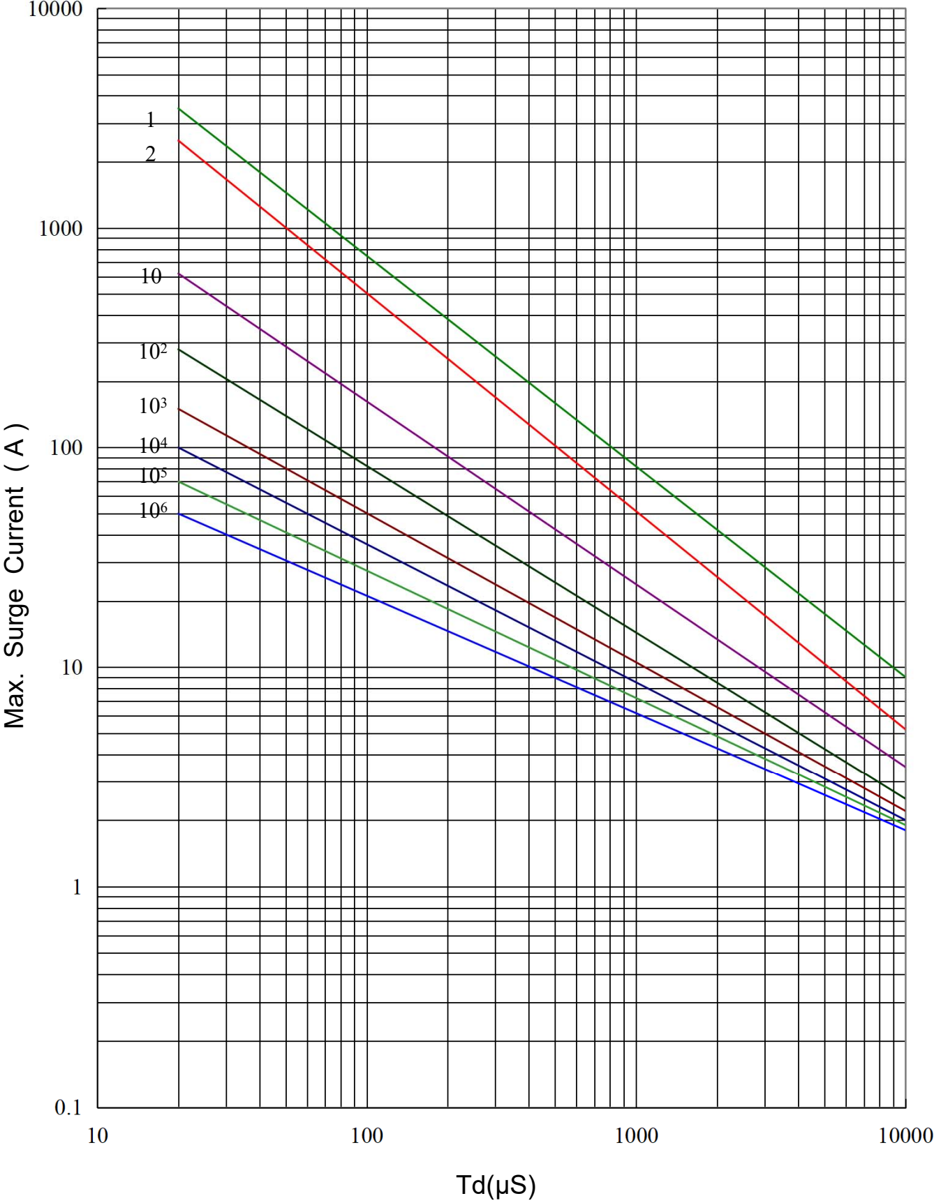
TVR10561KP323M
