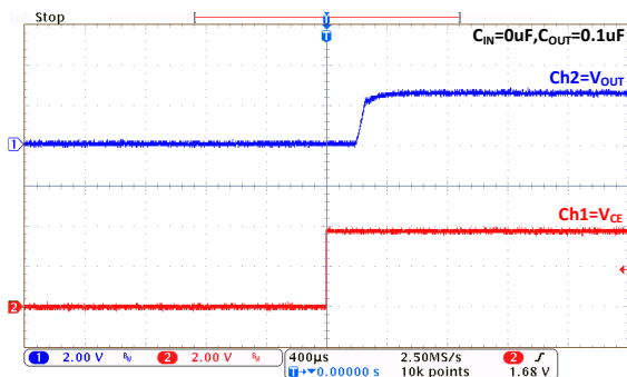
EN Enable: MD5125F ( I_{OUT}=1mA )
