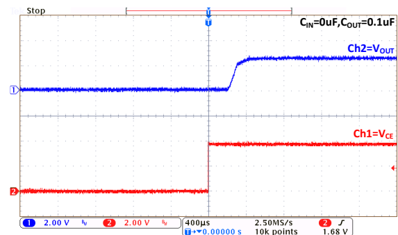
EN Enable: MD5125F ( I_{OUT}=100mA )
