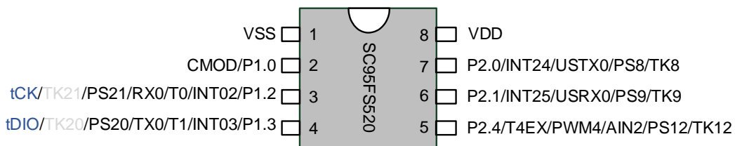
SC95FS520 管脚配置图 (SOP8)
