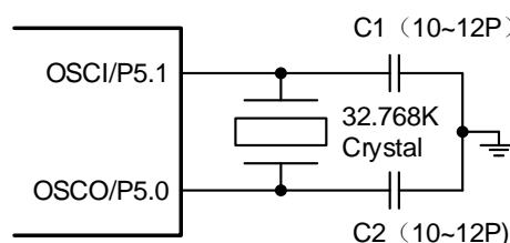
32.768kHz 外部晶振连接图
