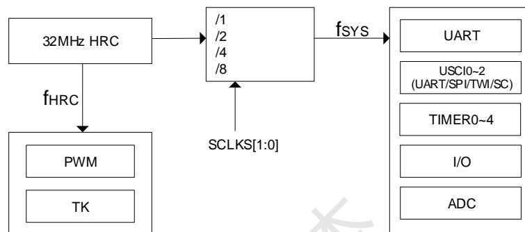
SC95FS52X 内部时钟关系
