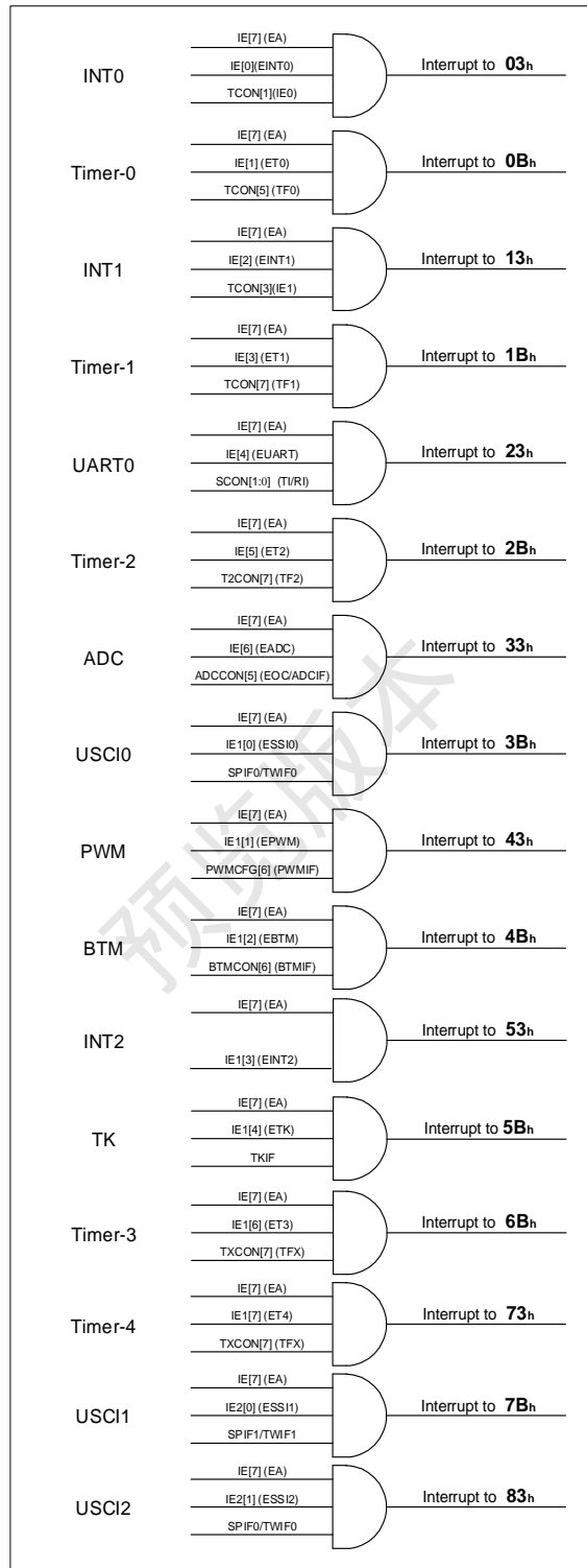
SC95FS52X 中断结构和向量
