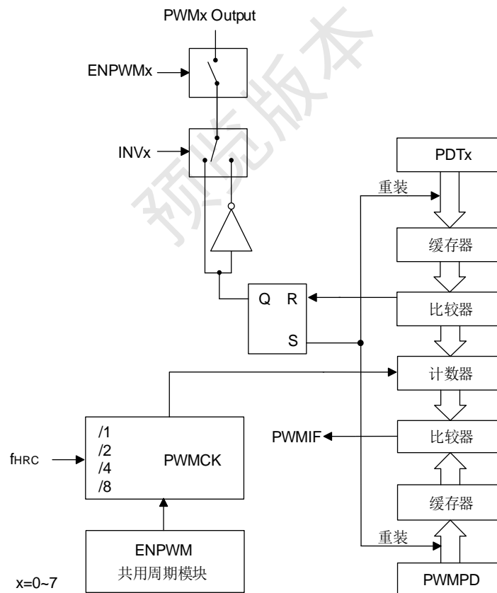
SC95FS52X PWM 独立模式框图
