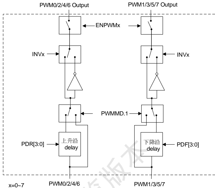
SC95FS52X PWM 互补模式框图
