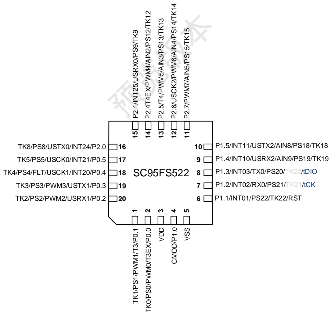
SC95FS522 管脚配置图 (QFN20 3*3)
