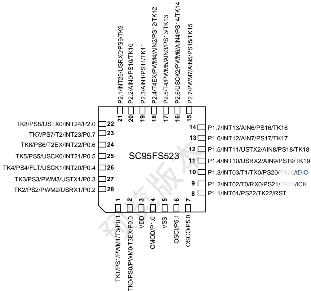
SC95FS523 管脚配置图 (QFN28 4*4)
