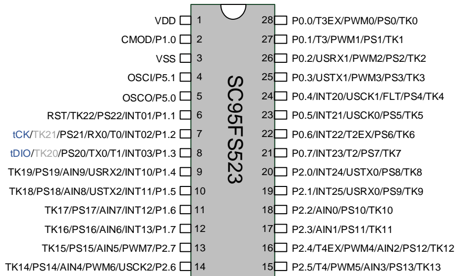
SC95FS523 管脚配置图 (SOP28/TSSOP28)
