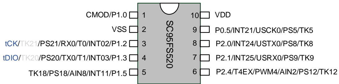
SC95FS520 管脚配置图 (MSOP10)
