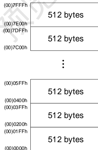
SC95FS52X 32 Kbytes Flash ROM Sector 分区示意
