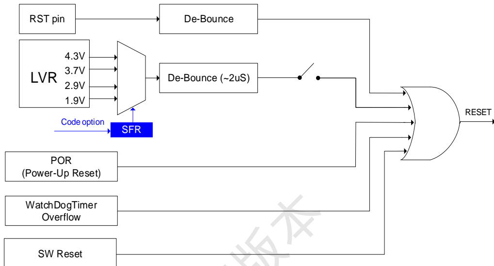
SC95FS52X 复位电路图
