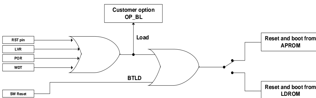
SC95FS52X 复位后启动区域切换示意图
