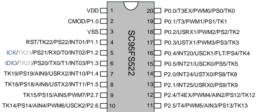
SC95FS522 管脚配置图
