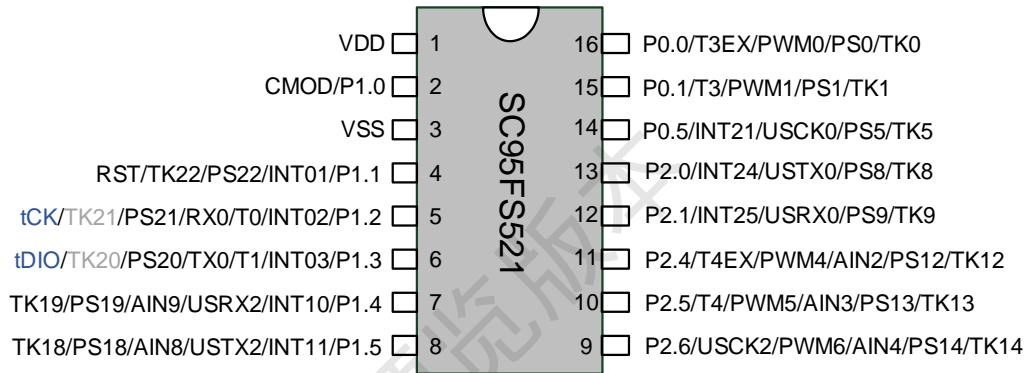
SC95FS521 管脚配置图
