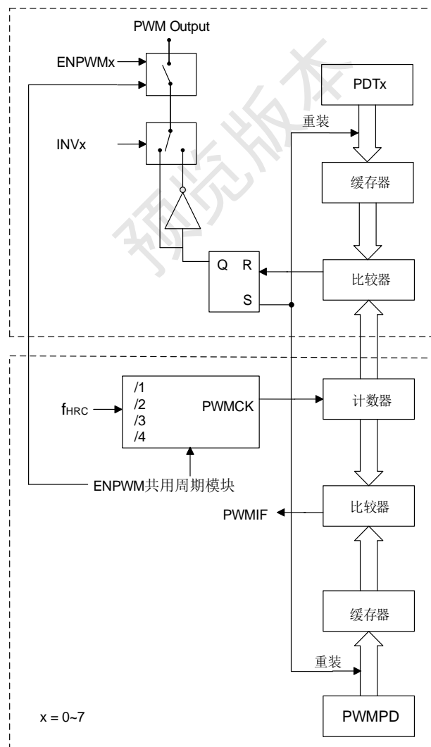
SC95FS52X PWM 结构框图
