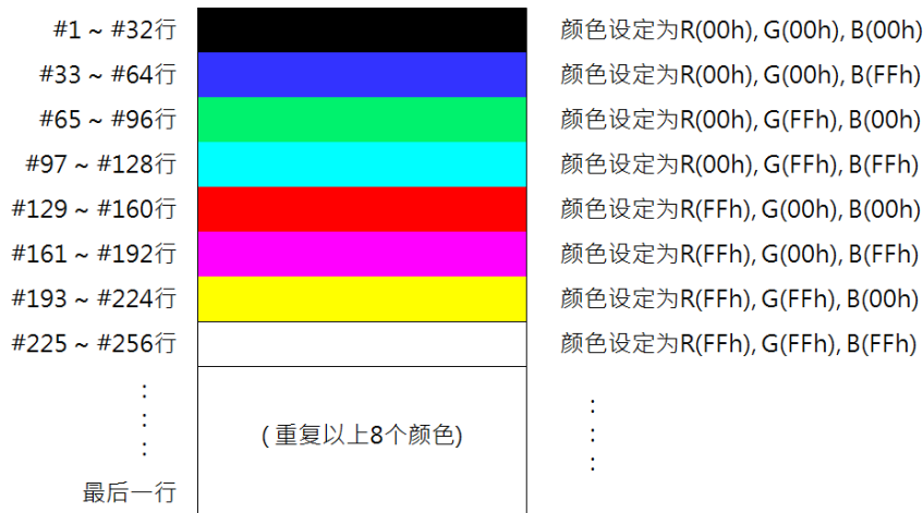
图 5-1: 彩条 (Color Bar) 显示
