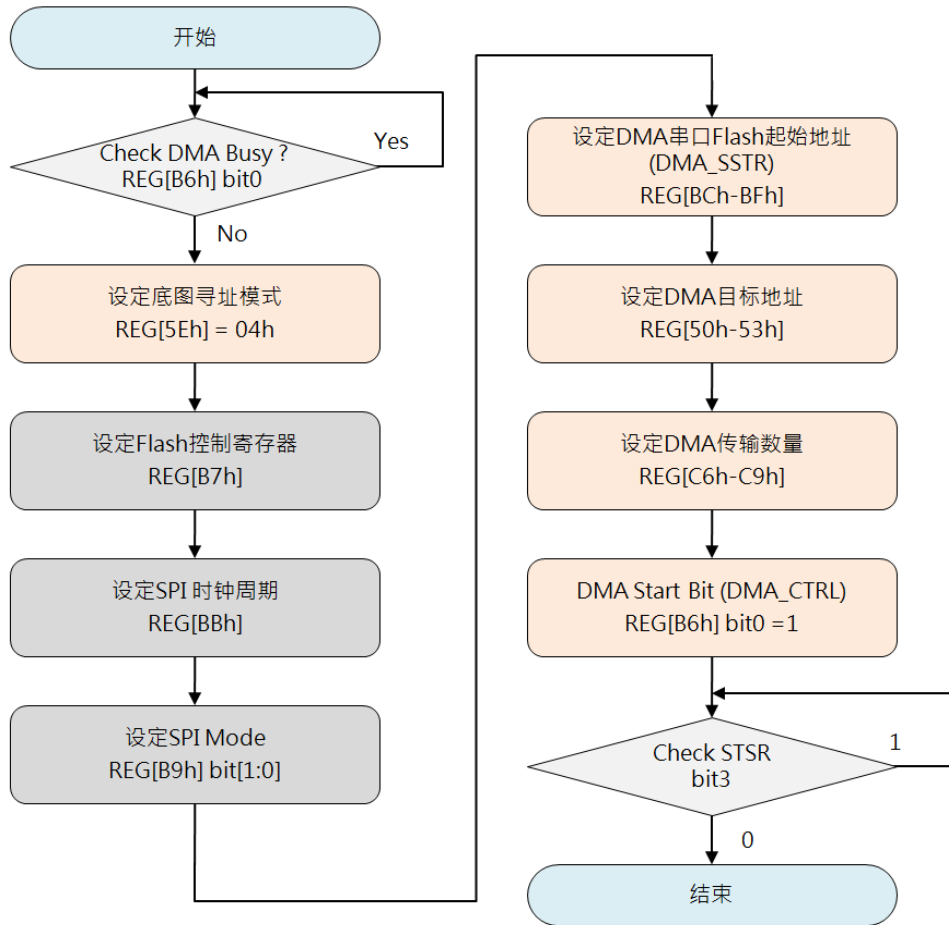
图 8-3: 使用 Serial Flash 进行 CGRAM 的初始化流程图
