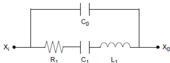
图 A-4: 晶振等效电路图
