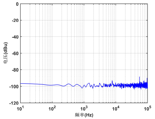
图 14 输出电压噪声(内部供电, 带载)
