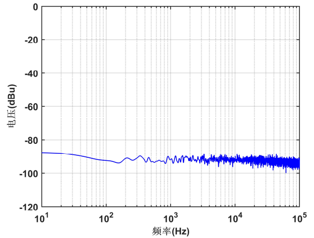
图 18 输出电压噪声(12V 线性电源外部供电, 带载)
