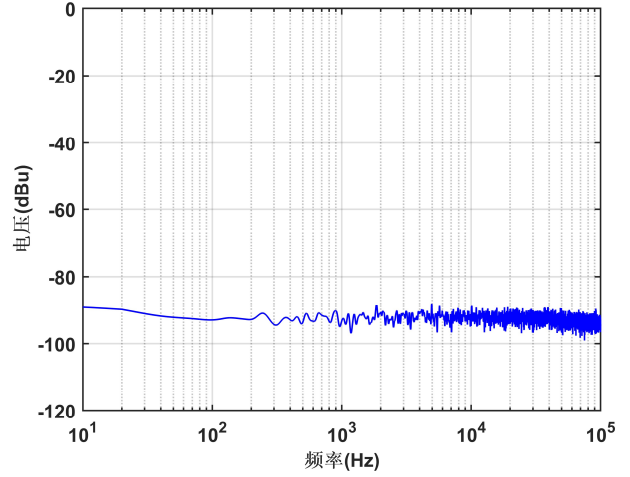
图 16 输出电压噪声(12V 开关电源外部供电, 带载)
