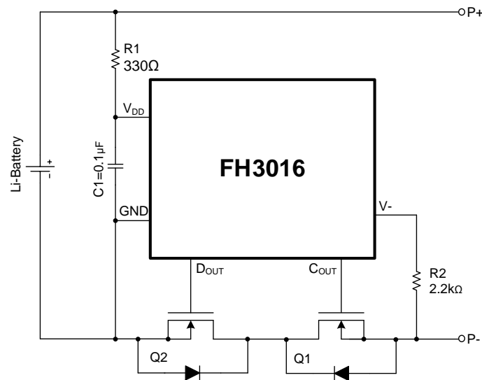
图-3 FH3016 系列典型应用电路图
