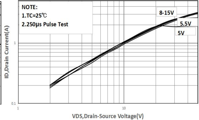
图 2 输出特性曲线, Tc=150°C
