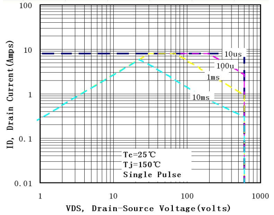
图 6-2 SIF2N65FB (TO-220FP) 最大安全工作区曲线
