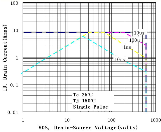
图 6-1 SIF2N65FB (TO-220) 最大安全工作区曲线
