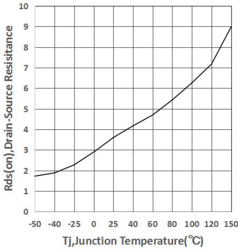
图 3 归一化导通电阻与温度曲线
