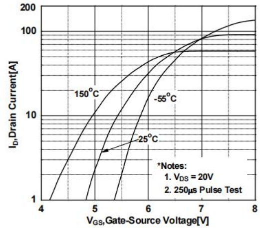
图 2 转移特性
