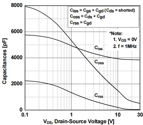
图 5 电容特性
