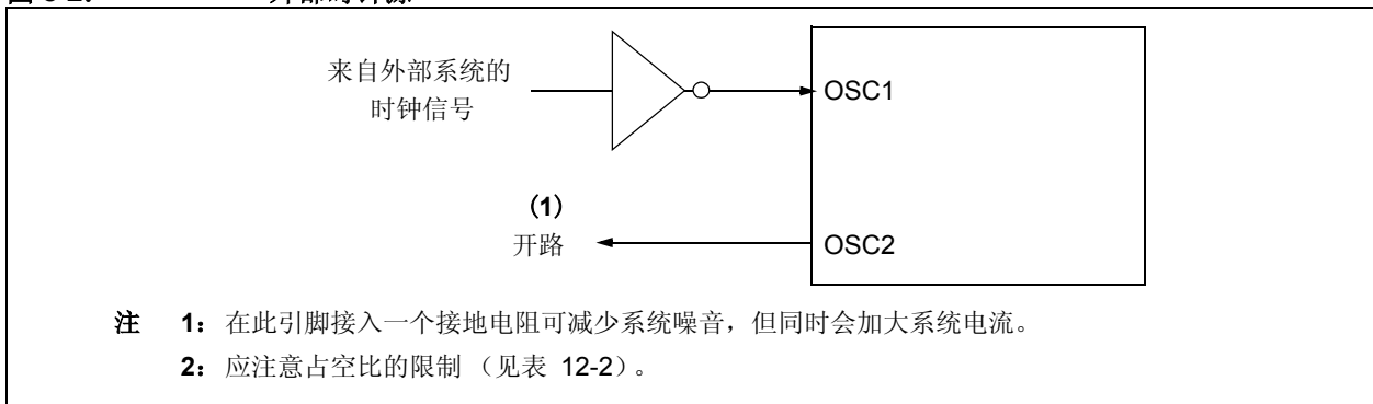
图 8-2: 外部时钟源
