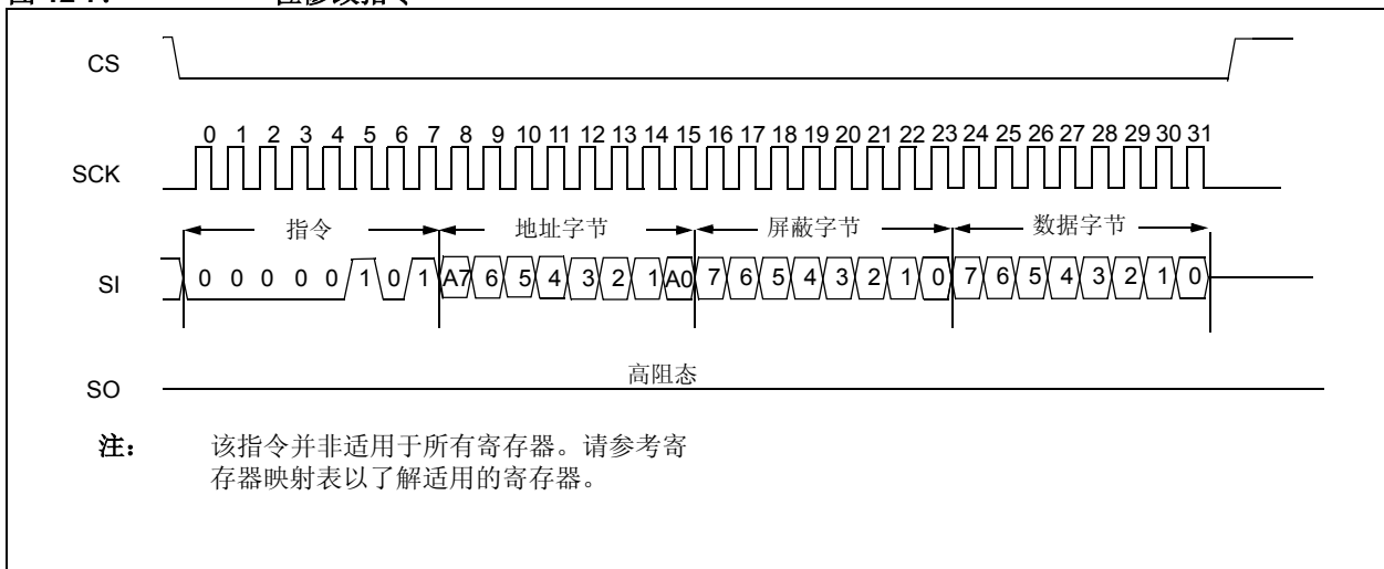
图 12-7: 位修改指令
