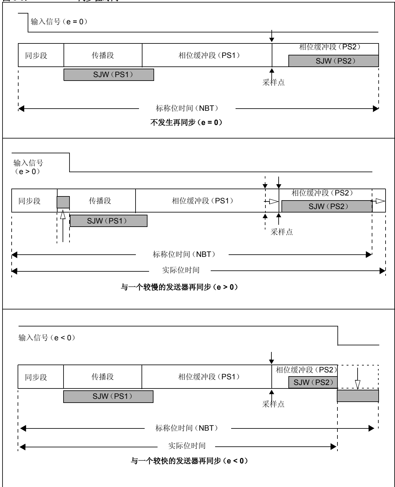
图 5-3: 同步位时间
