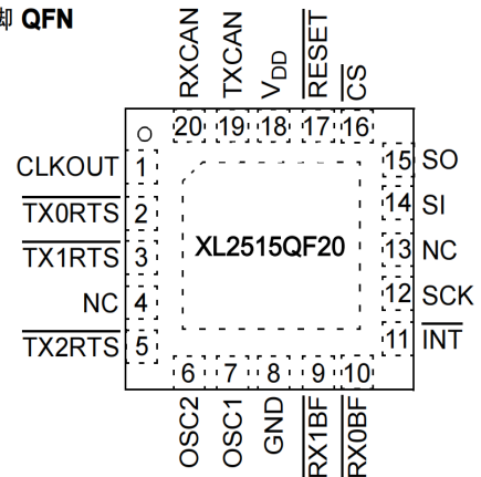
20 引脚 QFN
