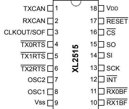
18 引脚 DIP/SOP
