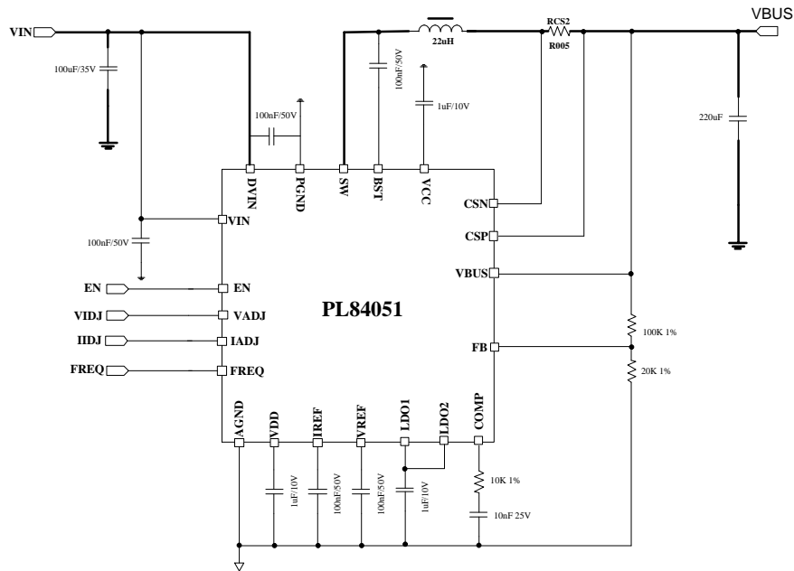
Fig. 20 Application Schematic (VABT:24V VBUS:12V IOOUT:5A)
