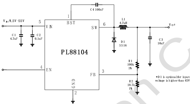
Fig. 1 Schematic
