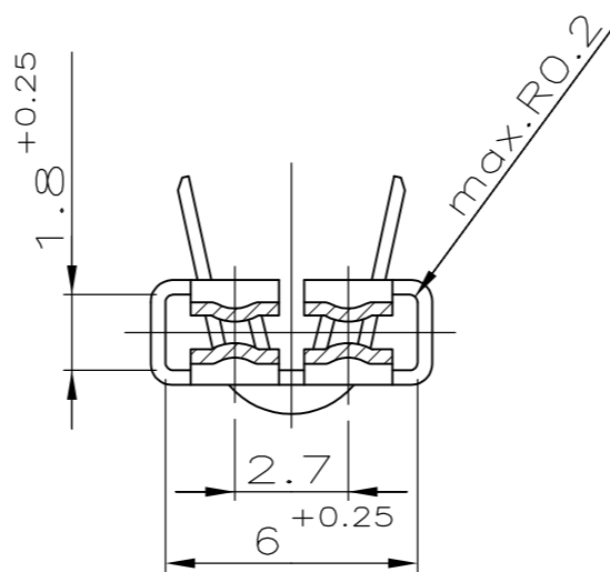
Schnitt A-A
