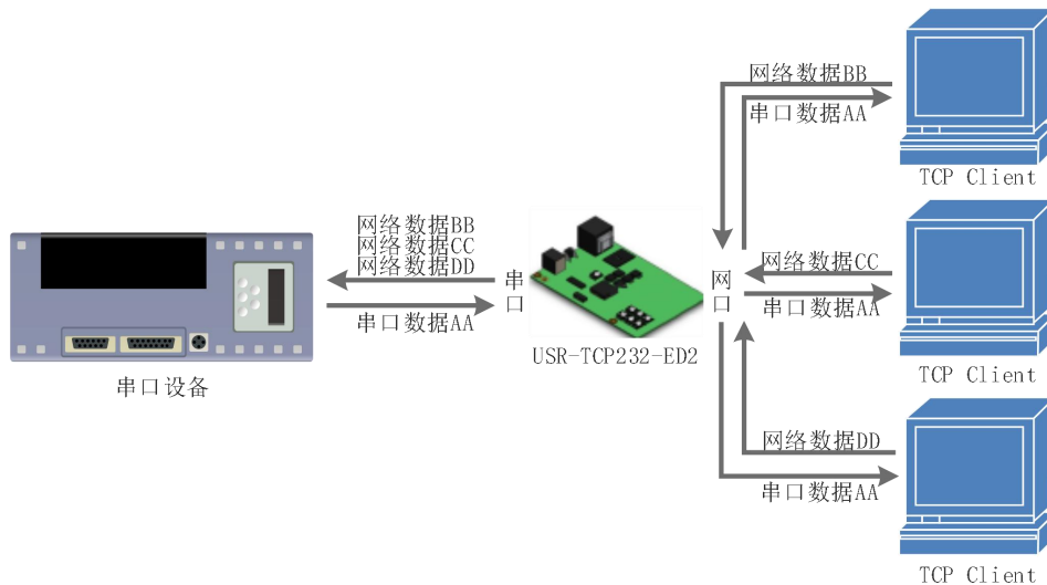
图 16 TCP Server 模式说明
