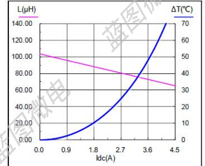
SMS1360-101M
