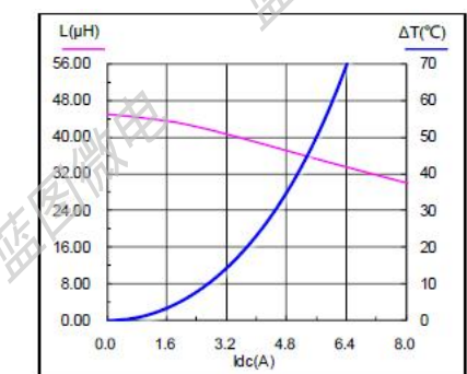
SMS1360-470M
