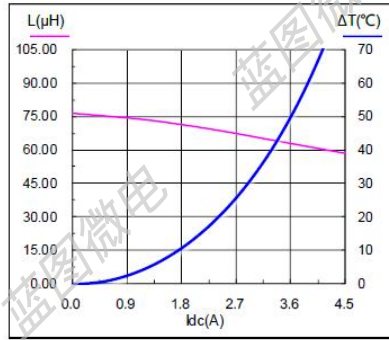
SMS1360-820M
