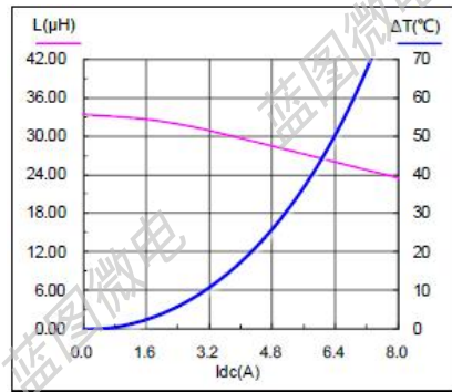
SMS1350-330M
