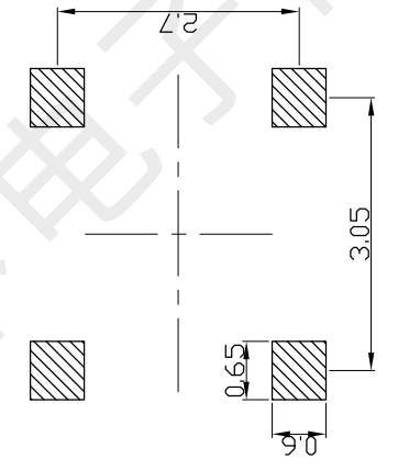
印刷板安装孔图
