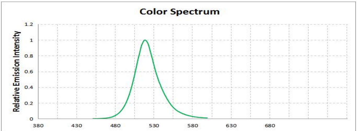
光谱图, T_a=25^\circ\text{C}
