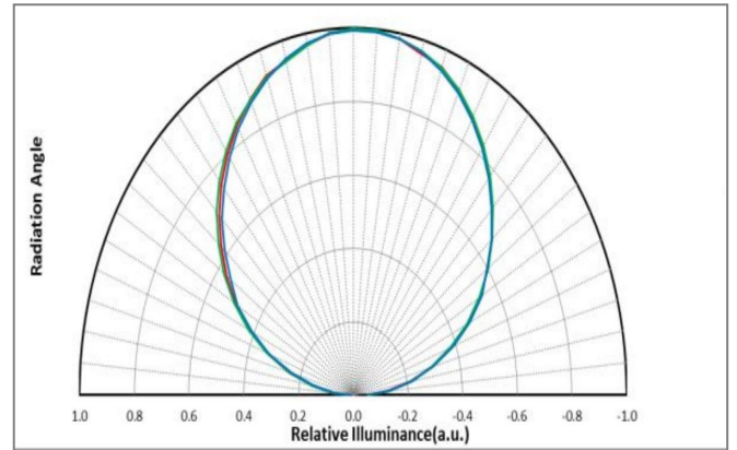
角度图, T_a=25^\circ\text{C}
