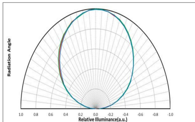
角度图, Ta=25°C
