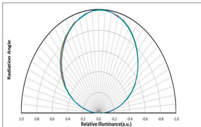
角度图, T_a=25^\circ\text{C}
