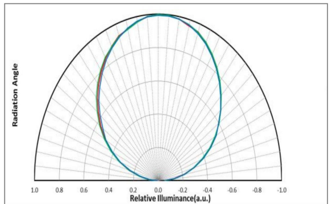
角度图, Ta=25°C
