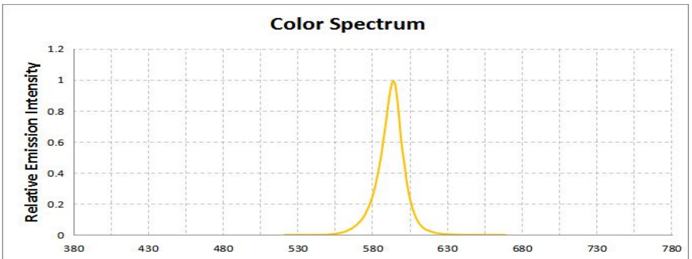
光谱图, Ta=25°C
