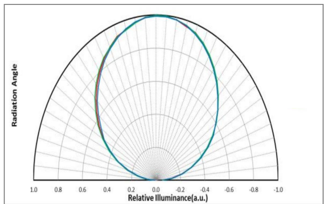
角度图, Ta=25°C
