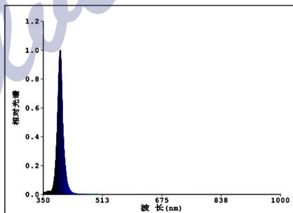
峰值波长
