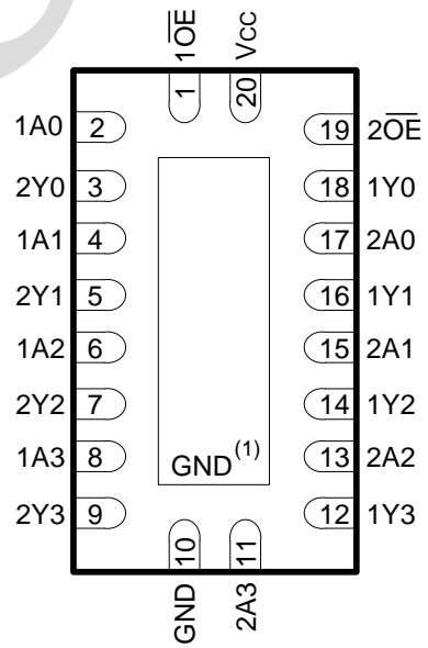
DHVQFN20
