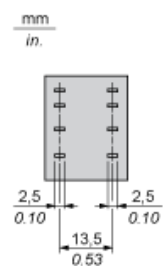
销钉侧视图
