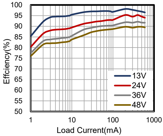
图 13.2-1 Efficiency 12V Output
