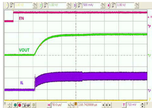
图 25. 启动, 3\ \Omega 负载
