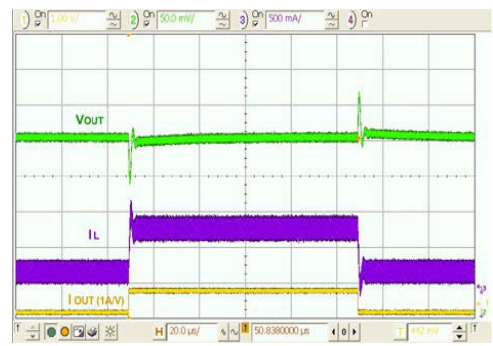
图 19. 负载瞬态, 200-800-200 mA, 100 ns 边沿
