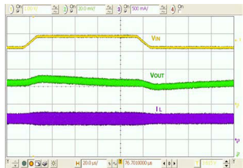
图 21. 线路瞬变, 3.3-3.9-3.3 V_{IN} , 10 \mu\text{s} 边沿, 600 mA 负载
