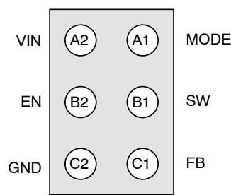
图 3. 焊球仰视图
