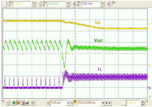
图 22. 组合线路/负载瞬态, 3.9\text{--}3.3\text{ V}_{IN} , 10\ \mu\text{s} 边沿, 36\text{--}400\text{ mA} 负载, 100\text{ ns} 边沿
