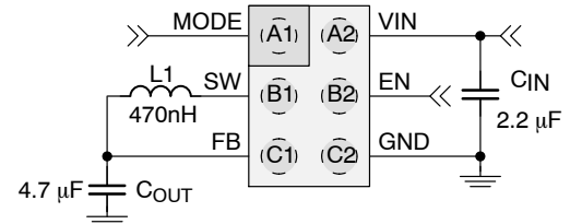
图 1. 典型应用
