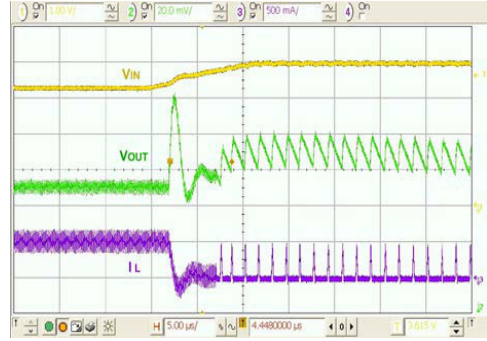
图 23. 组合线路/负载瞬态, 3.3\text{--}3.9\text{ V}_{IN} , 10\ \mu\text{s} 边沿, 400\text{--}36\text{ mA} 负载, 100\text{ ns} 边沿
