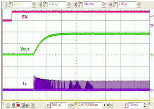
图 24. 启动, 50\ \Omega 负载
